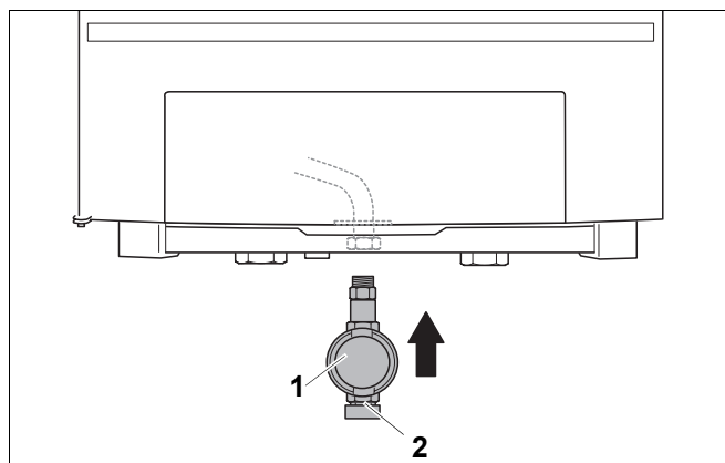
Рис. 4 Подключение газа
