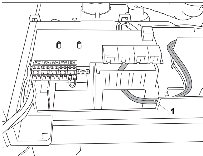
Рис. 19 Укладка подводящего кабеля насоса
