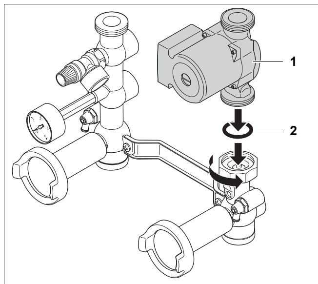
Рис. 8 Сборка насоса
