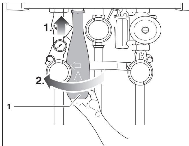
Рис. 11 Монтаж сифона
