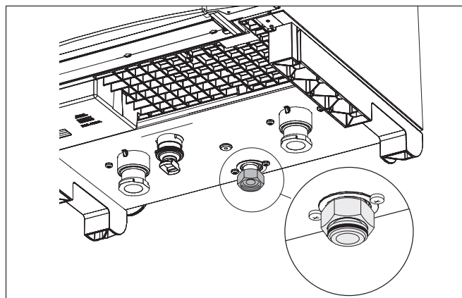
Рис. 3 Резиновая прокладка
