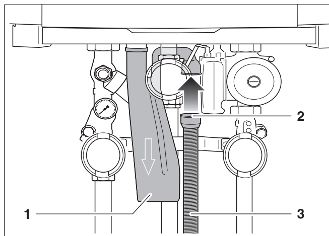
Рис. 12 Монтаж гофрированного шланга
