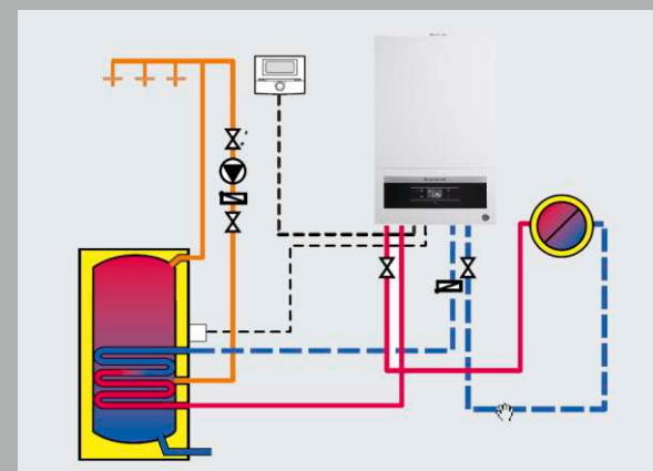
Приготовление горячей воды в баке косвенного нагрева
