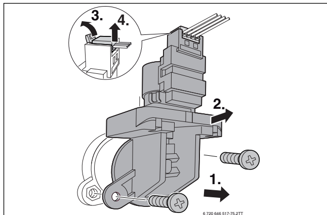
Мал. 70 Зняття 3-ходового клапана
