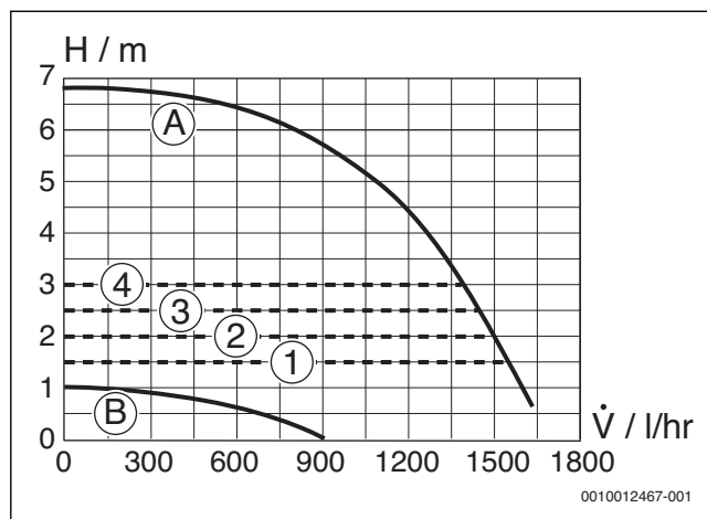
Мал. 83 Характеристики насоса та криві характеристик насоса
