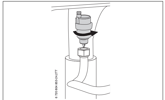
Мал. 68 Демонтаж автоматичного повітровідокремлювача
