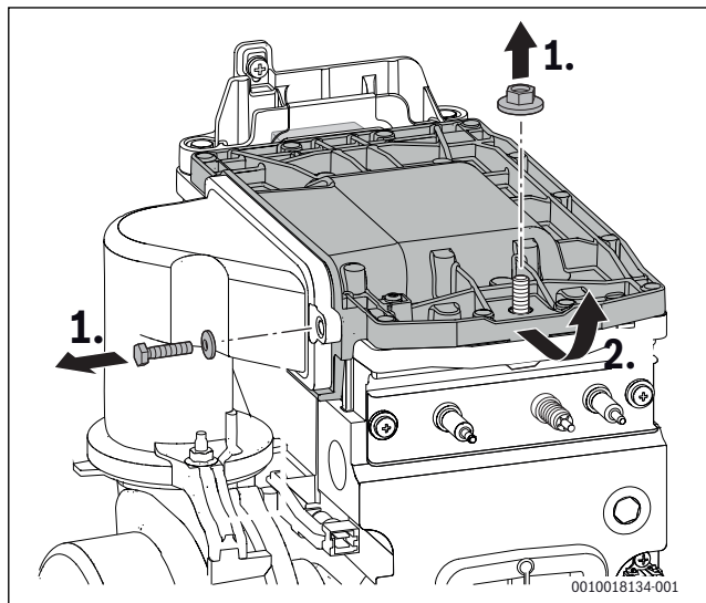
Мал. 58 Послабте кришку пальника
