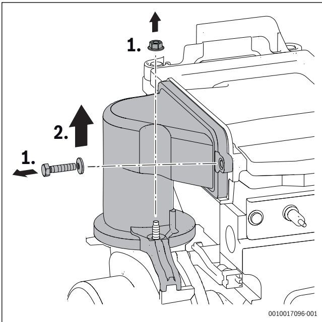
Мал. 66 Демонтуйте змішувальну камеру
