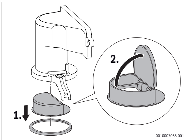
Мал. 67 Зворотний клапан змішувальної камери
