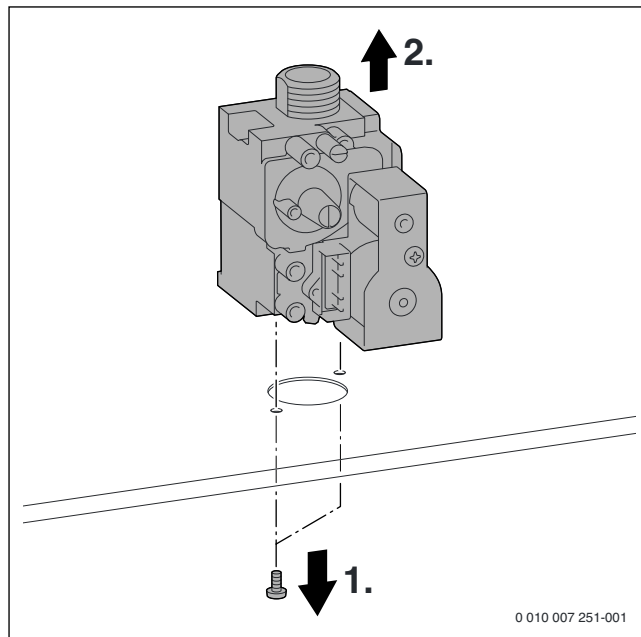
Мал. 74 Демонтаж газової арматури
