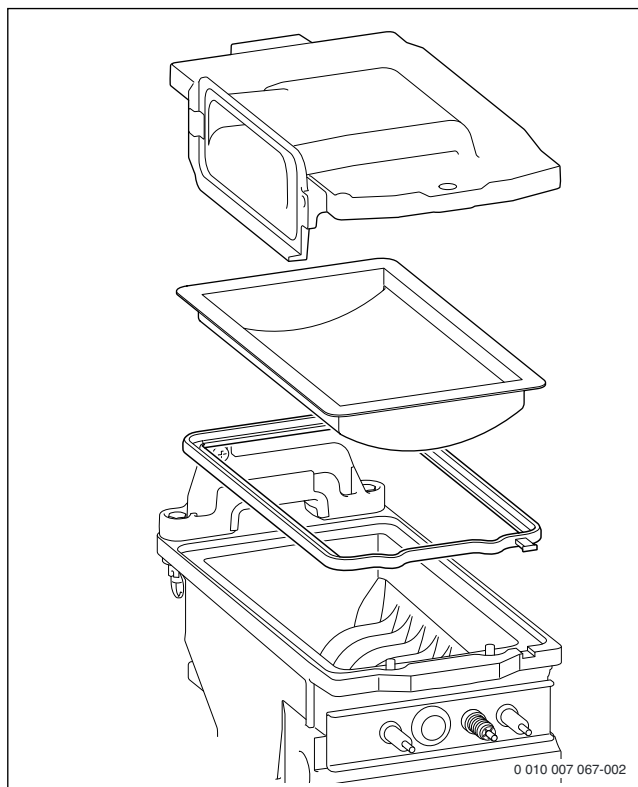
Мал. 59 Пальник
