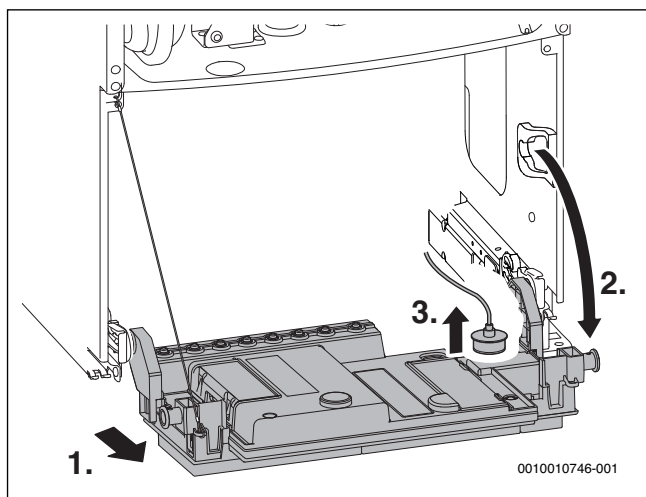
Мал. 76 Відкидання системи керування вниз
