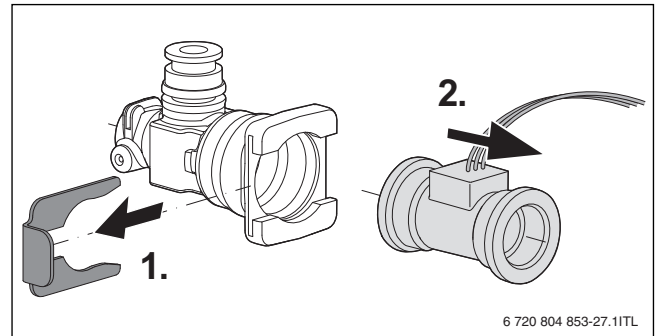
Мал. 55 Демонтаж турбіни на трубі холодної води
