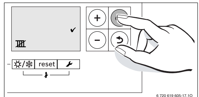
Мал. 44 Підтвердження літнього режиму вручну
