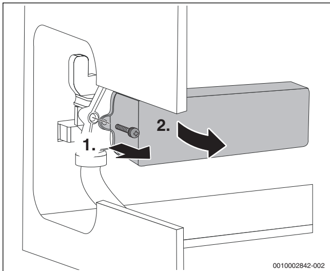
Мал. 53 Демонтаж пластинчастого теплообмінника
