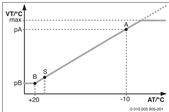
Мал. 82 Крива опалення
