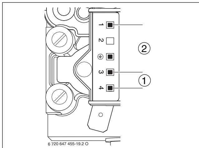
Мал. 71 Точки вимірювання на газовій арматурі
