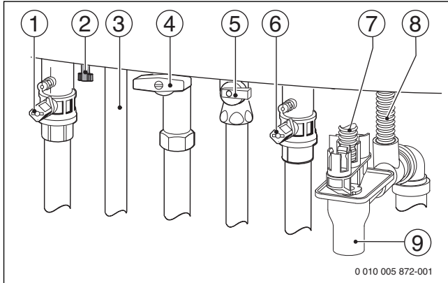
Мал. 28 Під'єднання з боку газо- та водопроводу (додаткова опція)
