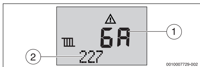
Мал. 80 Приклад: індикація несправності, що призводить до блокування
