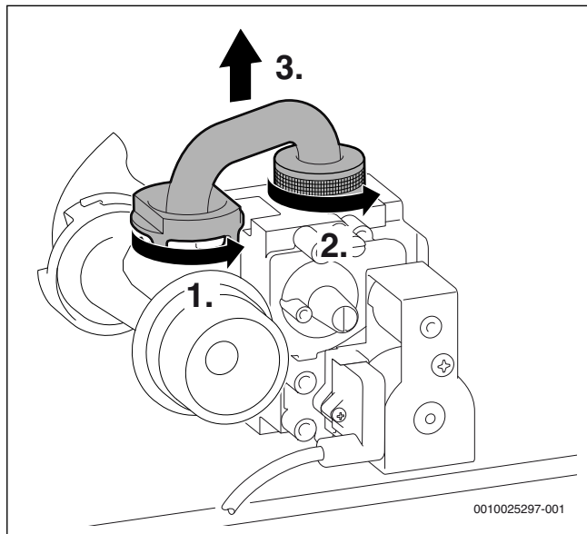
Мал. 72 Демонтаж газової труби
