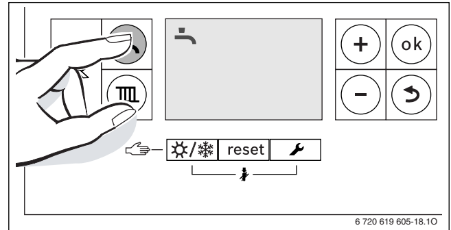
Мал. 39 Індикація режиму нагріву води
