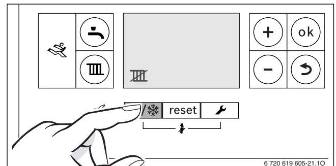
Мал. 43 Увімкнення літнього режиму вручну
