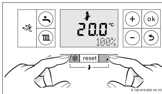
Мал. 51 100 % (максимальна номінальна теплопродуктивність гарячої води)
