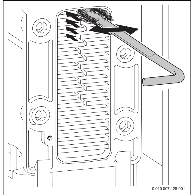
Мал. 62 Чищення котлового блоку, який включає камеру згоряння і теплообмінник, за допомогою щітки
