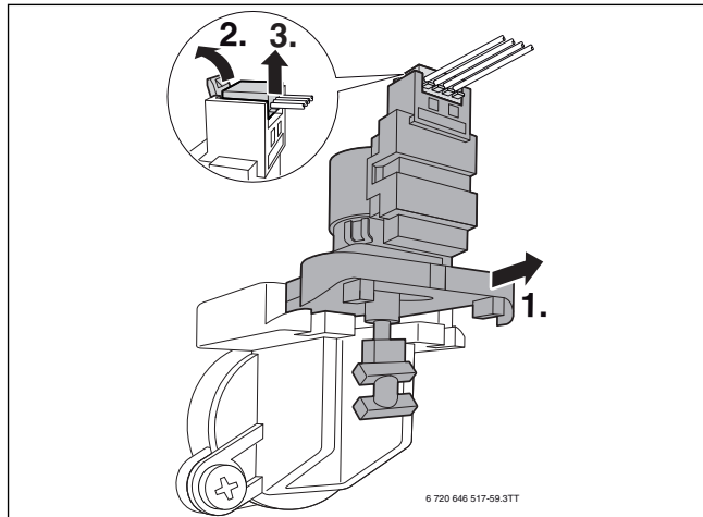
Мал. 69 Демонтаж двигуна 3-ходового клапана
