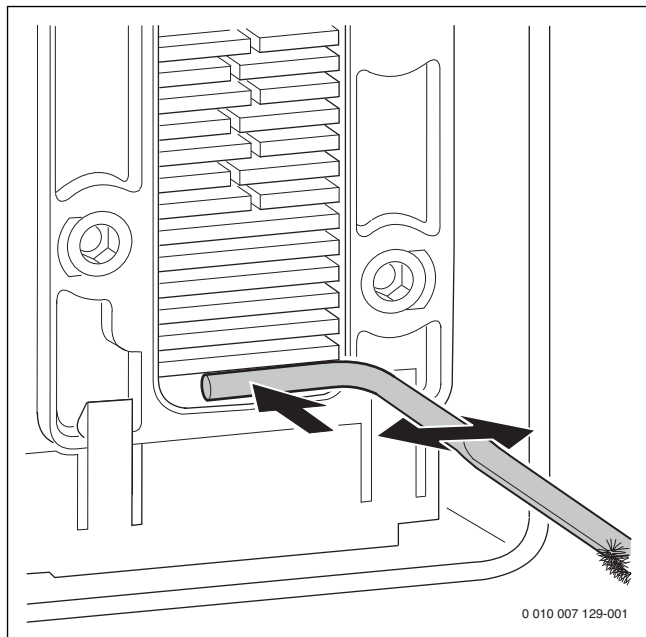
Мал. 64 Очищення конденсаційної ванни
