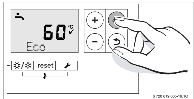
Мал. 40 Підтвердження індикації режиму eco
