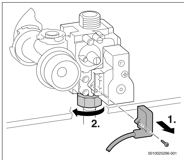
Мал. 73 Знімання штекера та відкручування накидної гайки
