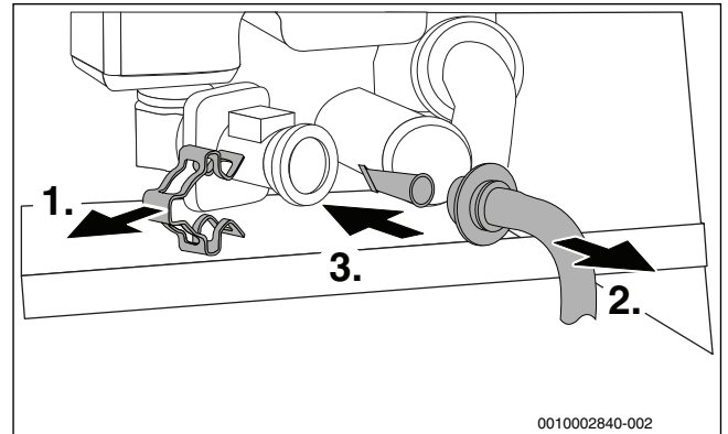
Мал. 54 Демонтаж фільтра в трубі холодної води
