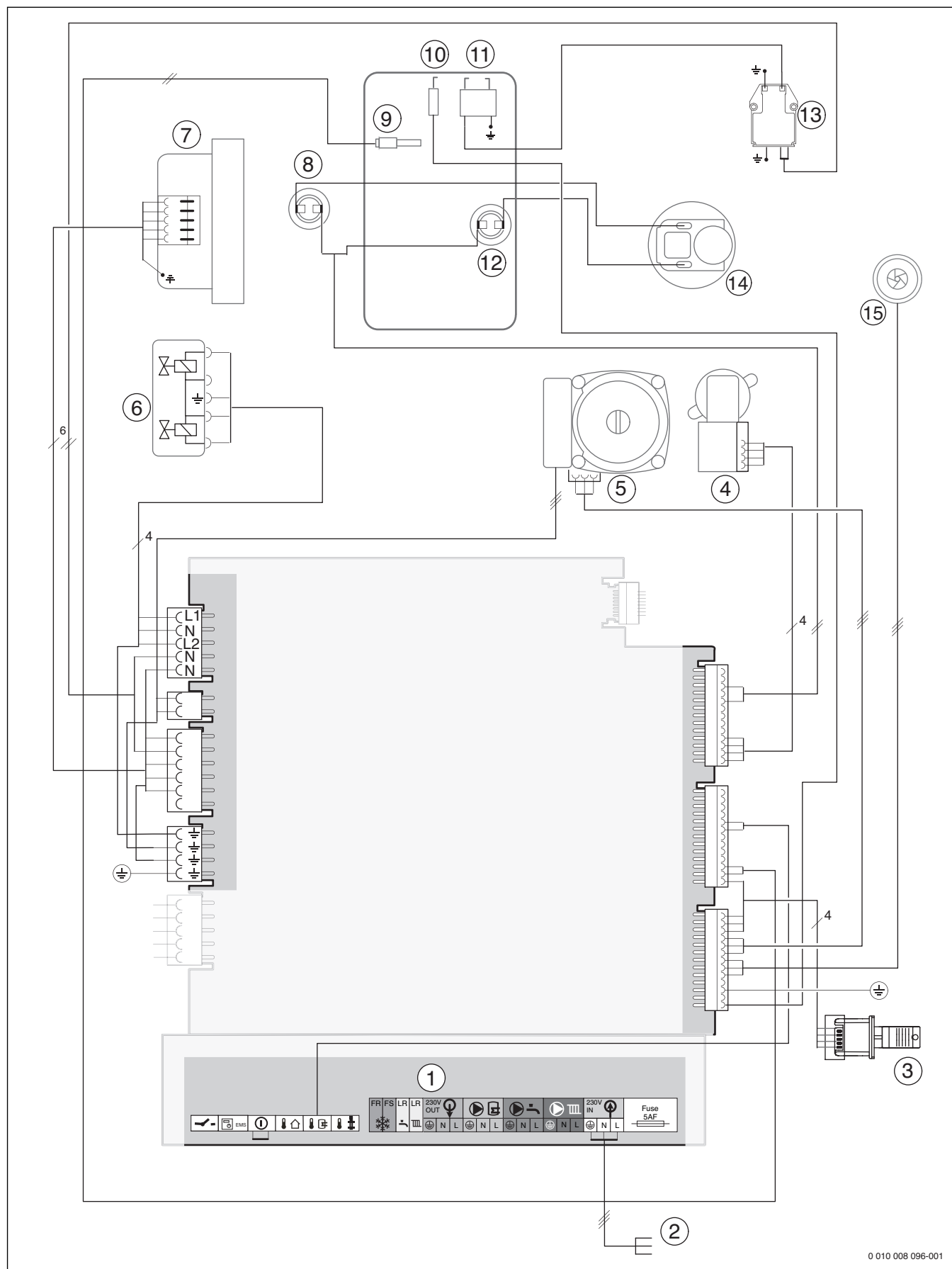
Мал. 81 Електричні підключення
