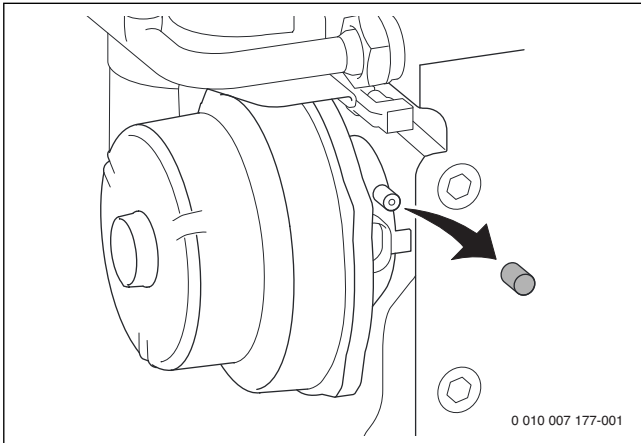
Мал. 60 Штуцер для вимірювання на змішувальній камері
