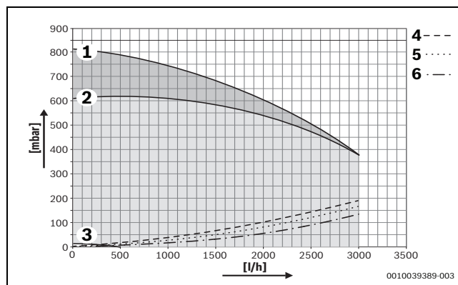
Мал. 52 Залишковий напір насоса GB272-50
