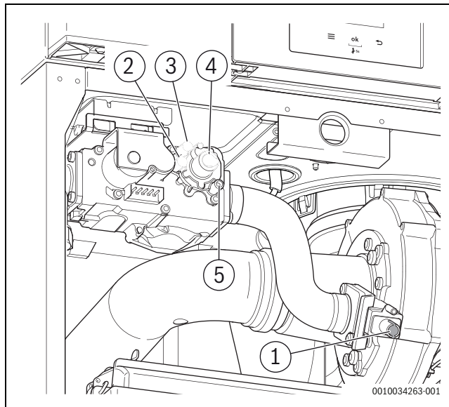
Мал. 33 Огляд штуцерів для вимірювання та регулювальних гвинтів ≥ 85 кВт
