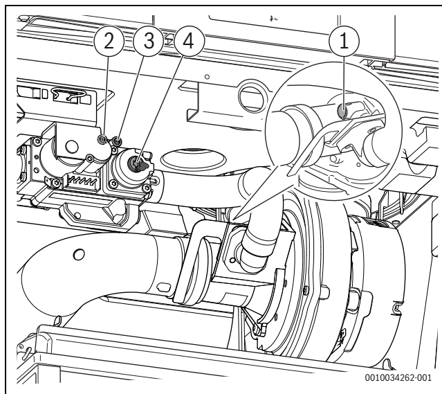
Мал. 32 Огляд штуцерів для вимірювання та регулювальних гвинтів ≤ 70 кВт
