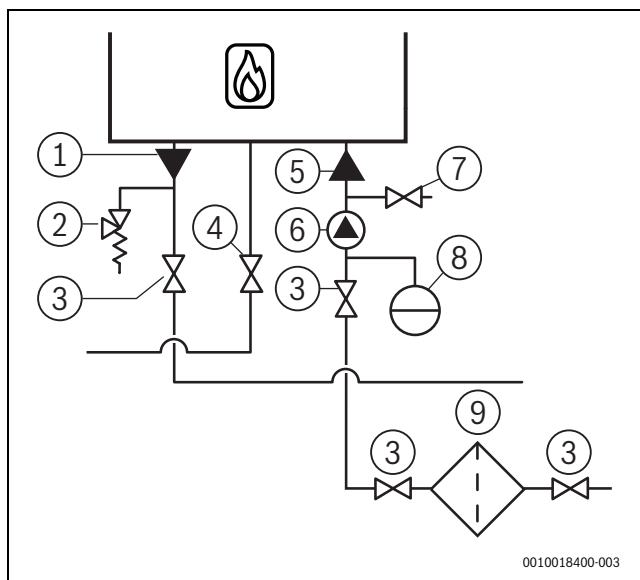
Мал. 18 Підключення труб для води системи опалення
