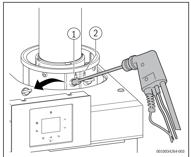
Мал. 34 Зняти заглушку на підключенні до димоходу
