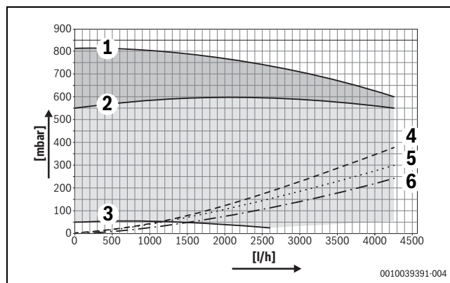
Мал. 53 Залишковий напір насоса 85kW-≤100kW
