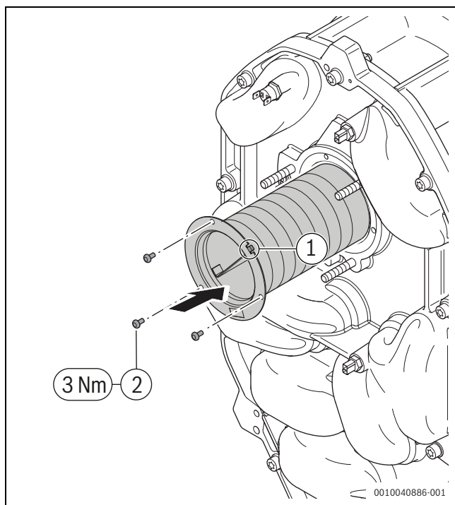
Мал. 44 Монтаж пальника
