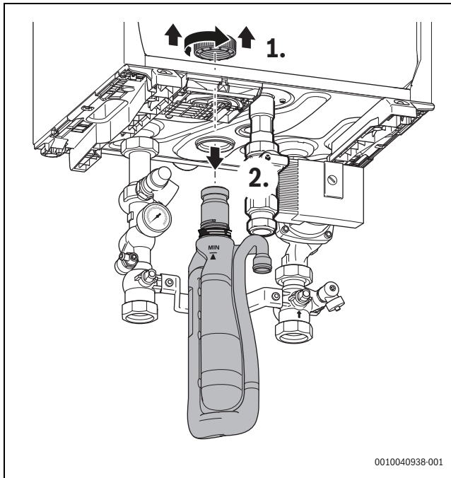
Мал. 43 Демонтаж сифона котла
