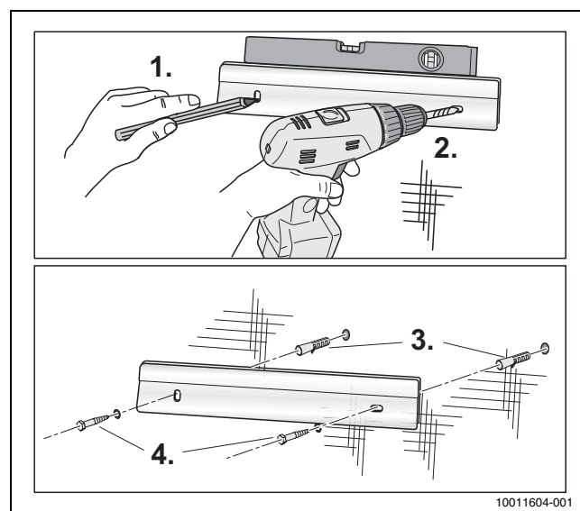
Мал. 11 Установка монтажної планки на бетонну стіну
