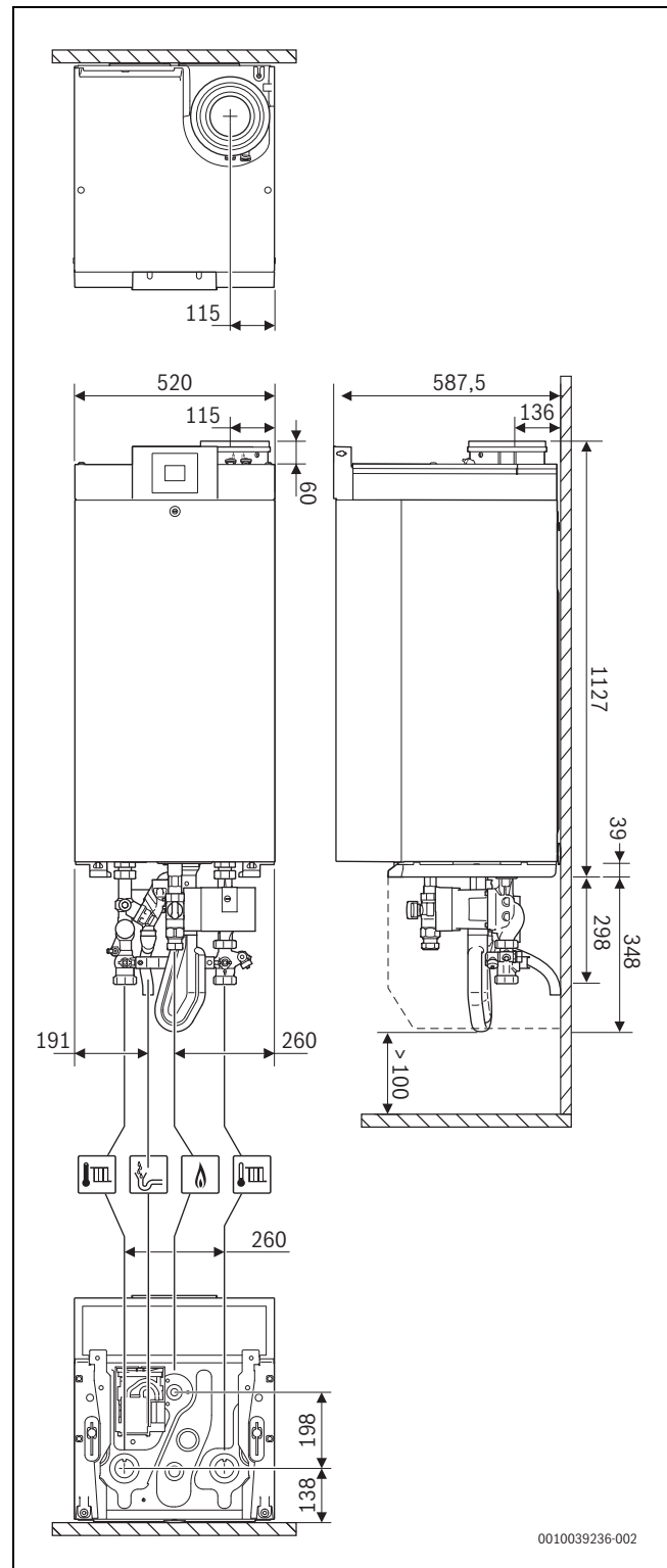
Мал. 3 Розміри на стіні [мм]
