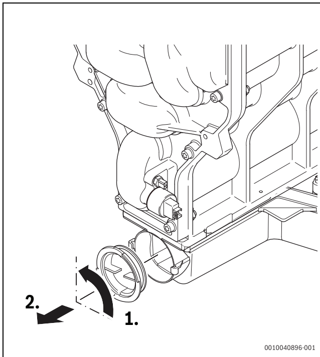
Мал. 42 Відкрити кришку конденсатовловлювача.
