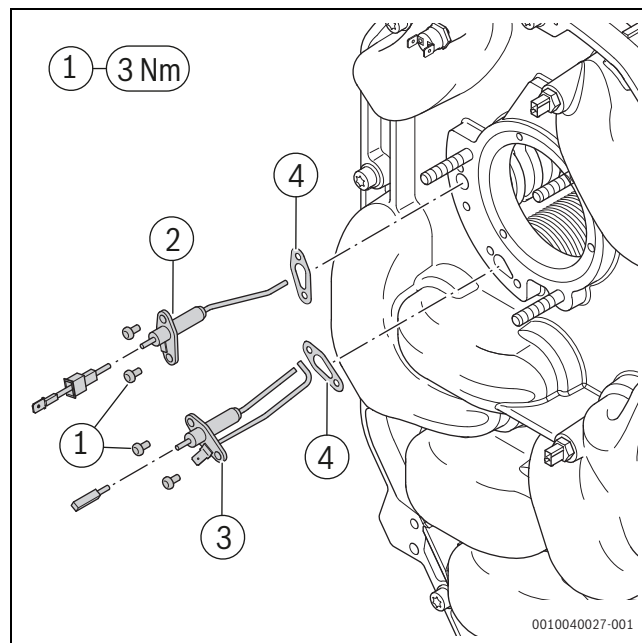
Мал. 48 Заміна іонізувального та запальвального електрода
