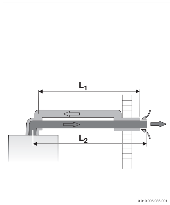
Мал. 7 Горизонтальне відведення димових газів за допомогою роздільної труби C_{12}
