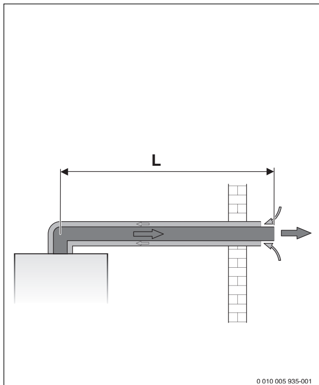
Мал. 6 Горизонтальне відведення відпрацьованих газів за допомогою концентричної труби C_{12}
