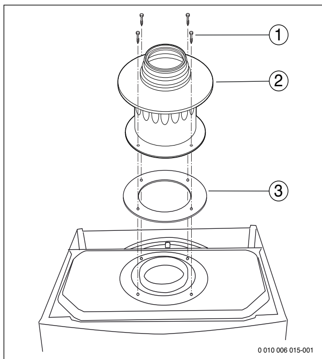
Мал. 19 При вертикальному відведенні димових газів B_{22} і потужності приладу = 35 кВт: встановлювати адаптер димових газів і дросельну заслінку
