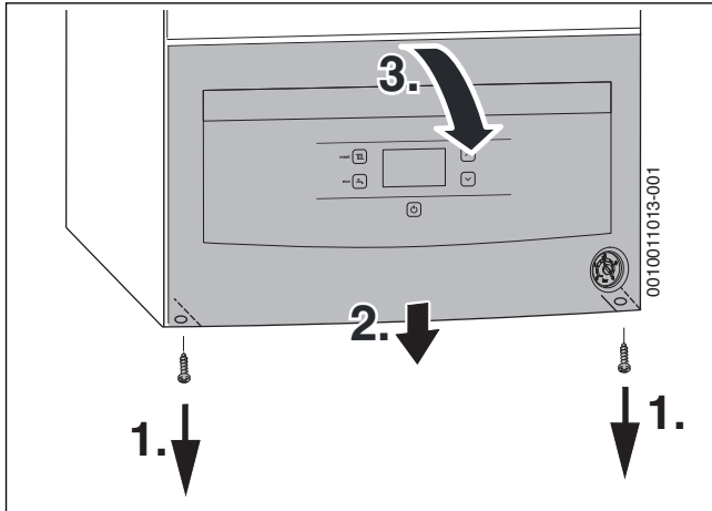
Мал. 16 Відкидання системи керування вниз
