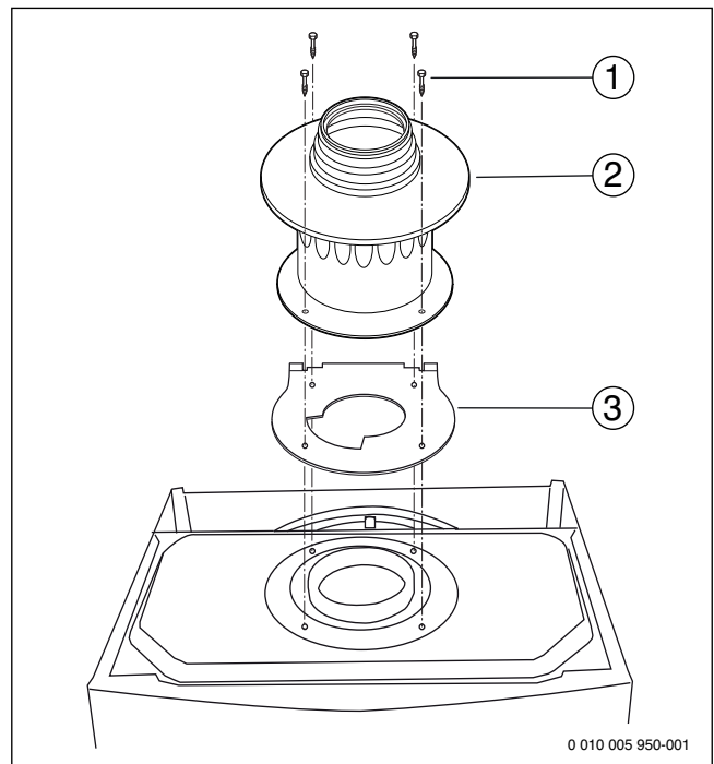
Мал. 18 При відведенні димових газів B_{22} і потужності приладу < 35 кВт: встановлювати адаптер димових газів і дросельну заслінку
