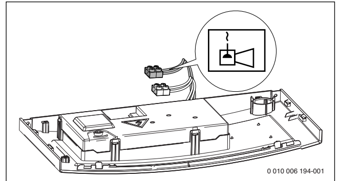
Мал. 25 Підключення контакту аварійного сигналу
