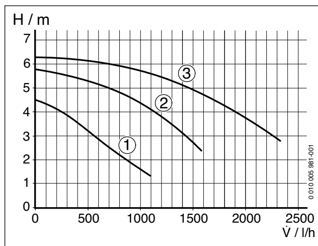
Мал. 30 Характеристична крива насоса опалювального контуру (потужність приладу = 35 кВт)
