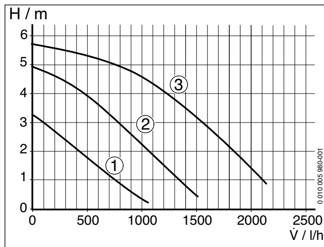
Мал. 29 Характеристична крива насоса опалювального контуру (потужність приладу < 35 кВт)
