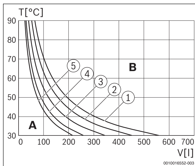
Мал. 12 Характеристична крива мембранного компенсаційного бака 6 л (потужність приладу < 35 кВт)
