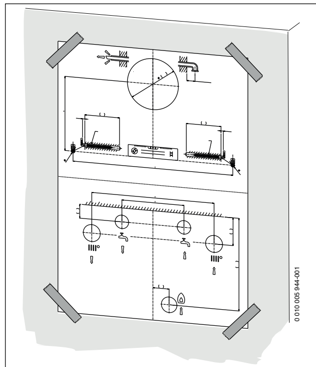
Мал. 14 Монтажний шаблон
