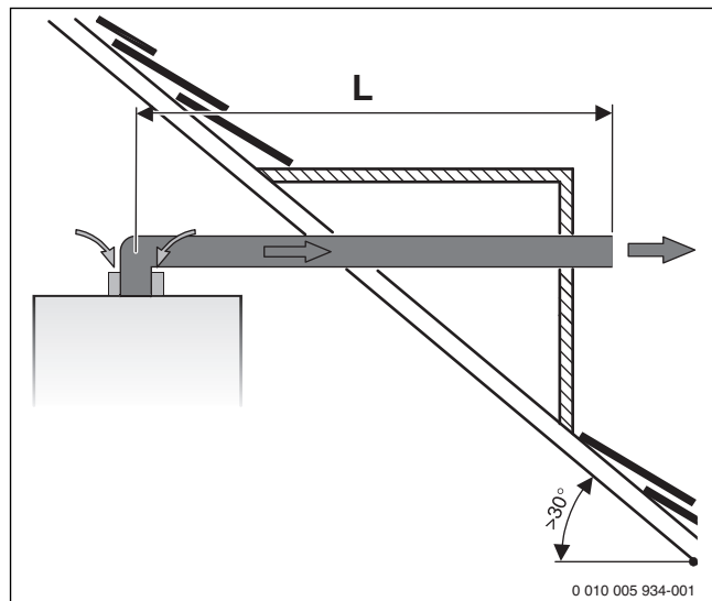
Мал. 4 Горизонтальне відведення димових газів B_{22}
