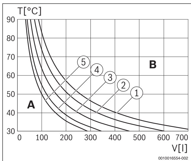
Мал. 13 Характеристична крива мембранного компенсаційного бака 8 л (потужність приладу = 35 кВт)
