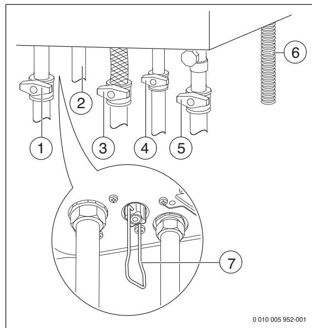
Мал. 20 Під'єднання з боку газо- та водопроводу (приладдя)
