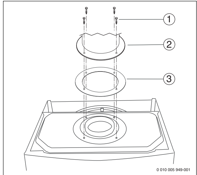
Мал. 17 Кріплення аксесуарів для відведення відпрацьованих газів
