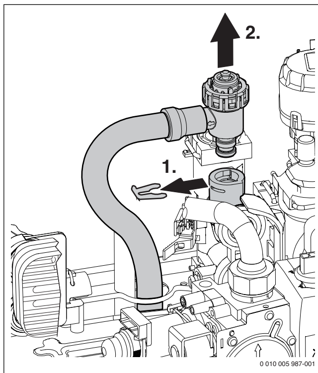
Мал. 35 Знімання запобіжного клапану (контур опалення)
