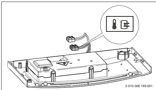
Мал. 24 Підключення датчика температури бака-водонагрівача
