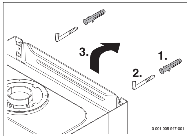
Мал. 15 Кріплення приладу на гачки, що вкручуються
