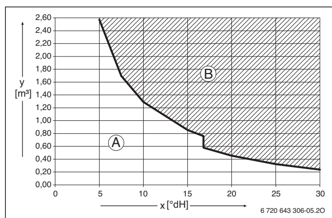
Мал. 11 Вимоги до води для наповнення та підживлення теплогенераторів < 50 кВт
