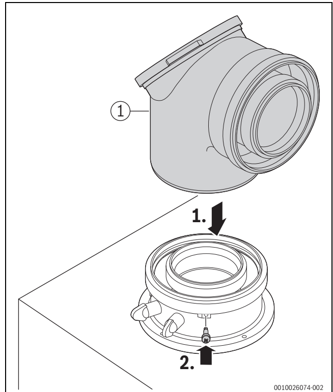
Мал. 35 Встановіть аксесуари для відведення відпрацьованих газів та зафіксуйте гвинтом
