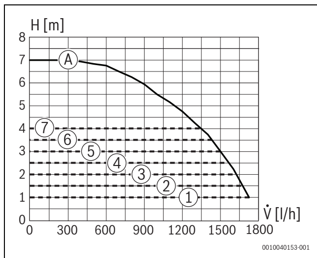
Мал. 73 Характеристики насоса та криві характеристик насоса
