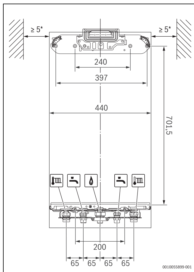
Мал. 3 Вид спереду (мм) з монтажною приєднувальною панеллю (додаткові комплектуючі)
