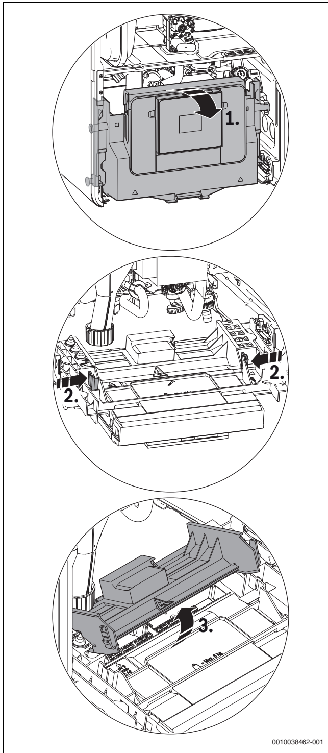
Мал. 37 Відкидання частини корпусу
