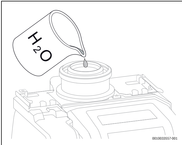
Мал. 34 Наповніть сифон для відведення конденсату водою
