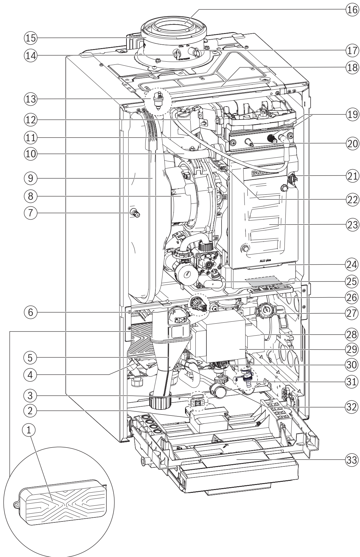
Мал. 5 Огляд виробу, двоконтурний котел
