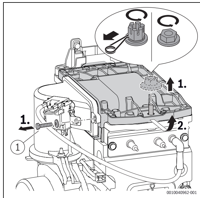
Мал. 51 Демонтаж кришки пальника
