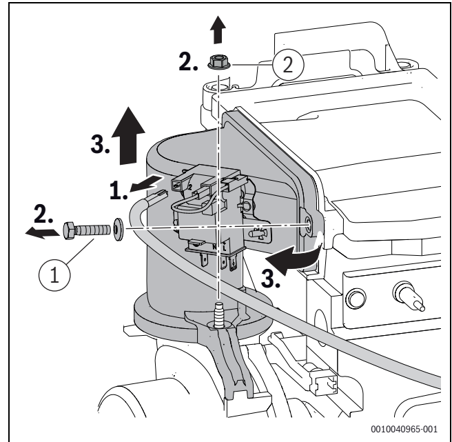
Мал. 54 Демонтуйте змішувальну камеру
