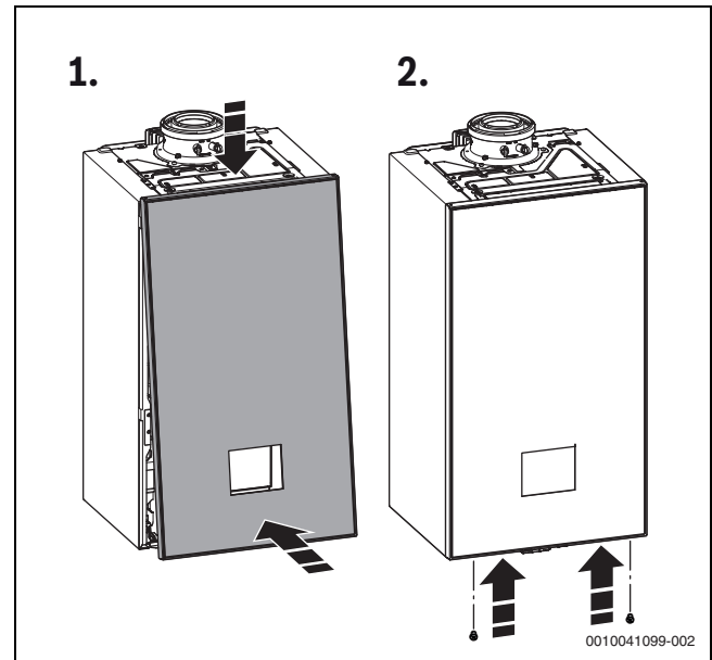
Мал. 42 Монтаж кожуха
