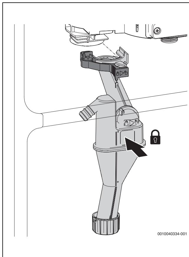
Мал. 65 Встановлення сифона для відведення конденсату
