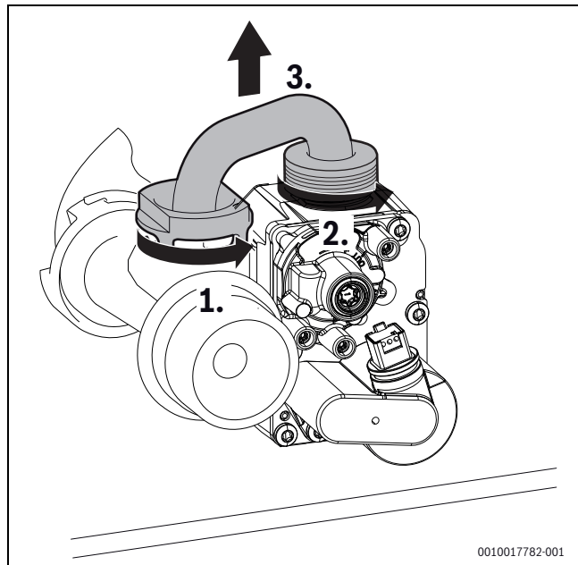
Мал. 66 Демонтаж газової труби
