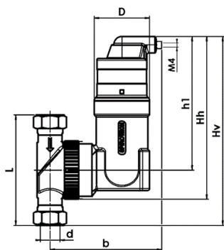
Конструктивні розміри різьбове з'єднання затискного кільця 22 мм і 28 мм
