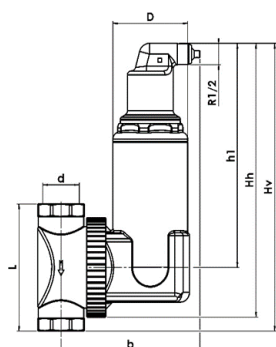
Конструктивні розміри внутр. різьба 1 \frac{1}{4} ", 1 \frac{1}{2} " і 2"
