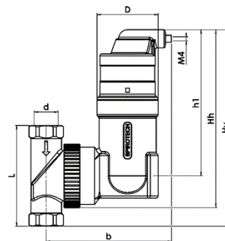
Конструктивні розміри внутр. різьба \frac{3}{4} " і 1"
