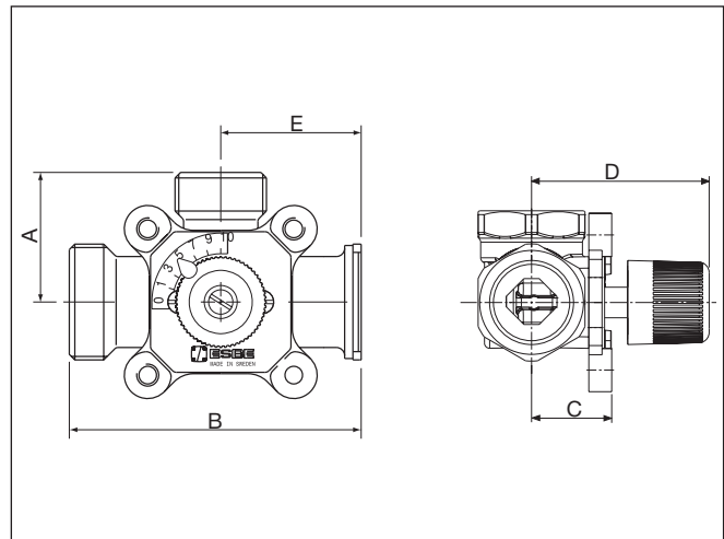
20/2 Габаритні розміри
