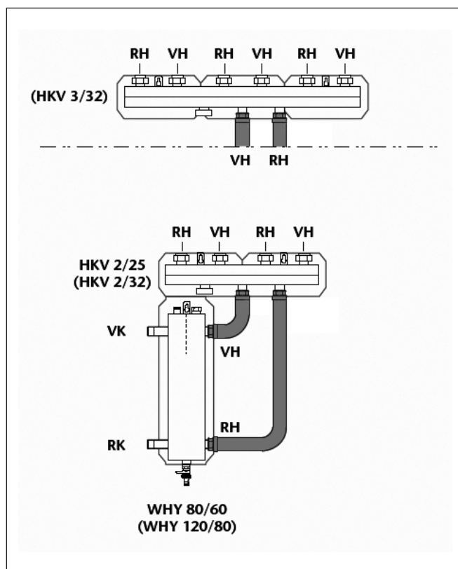
11/1 Труби для з'єднання гідравлічної стрілки WHY 60/80 з розподільчим колектором HKV 2/25 (або WHY 80/120 з HKV 2/32 або HKV 3/32)
