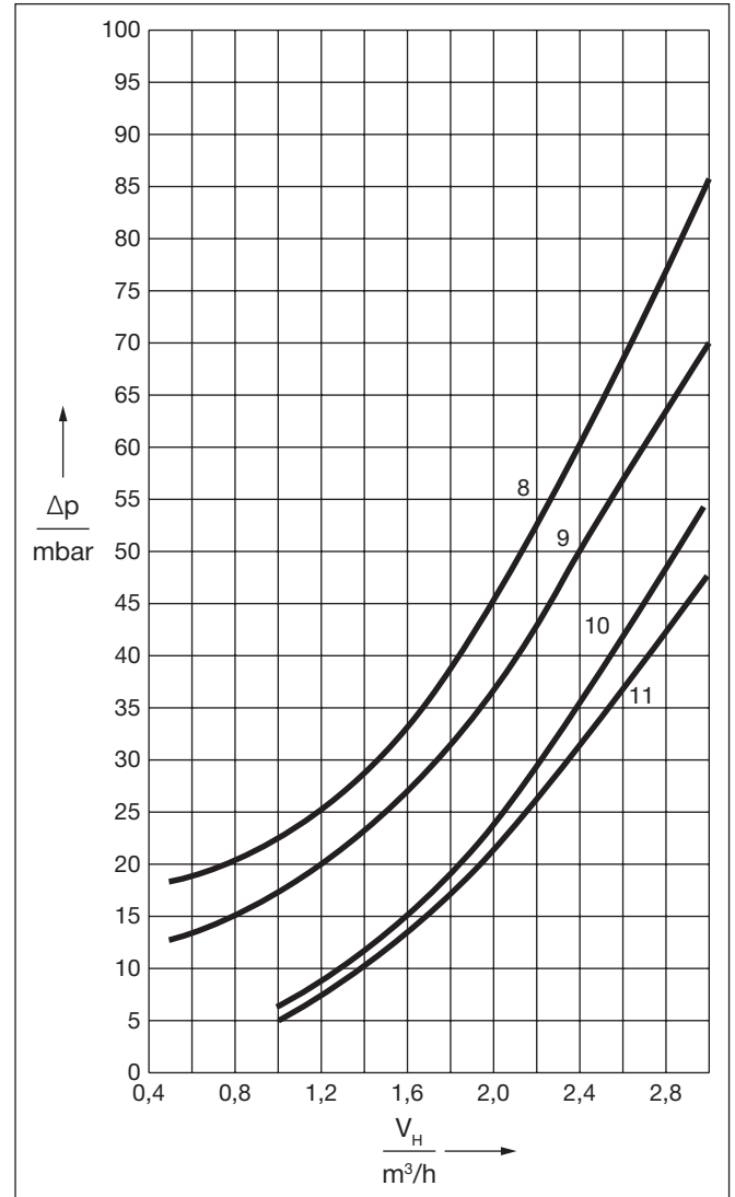
21/2 Гідравлічний опір по воді мережі комплектів швидкого монтажу HS 32, HSM 32, HKV 2/32 і HKV 3/32
