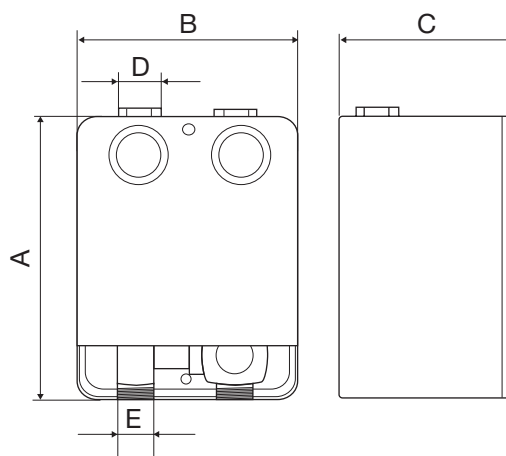
6/1 Габаритні розміри комплектів швидкого монтажу HS/HSM
