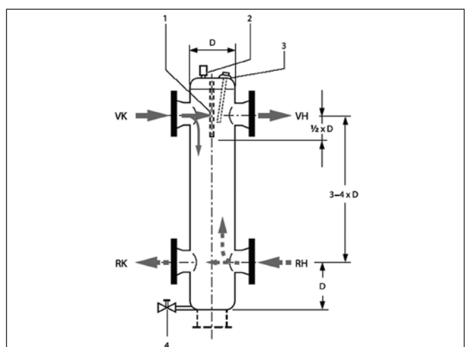
10/3 Конструкція гідравлічної стрілки
