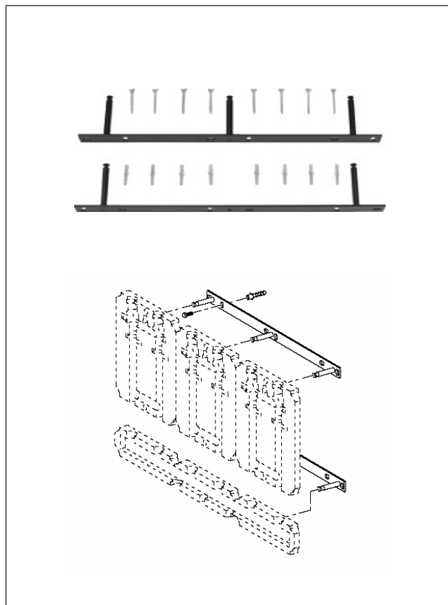
8/1 Комплект настінного монтажу WMS 3 для установки трьох опалювальних контурів
