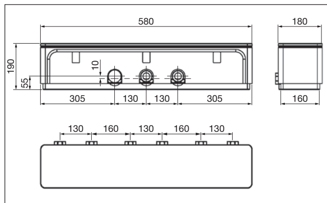
7/2 Габаритні розміри НКВ 3/..
