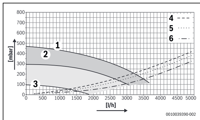
Мал. 53 Залишковий напір насоса GB272-70
