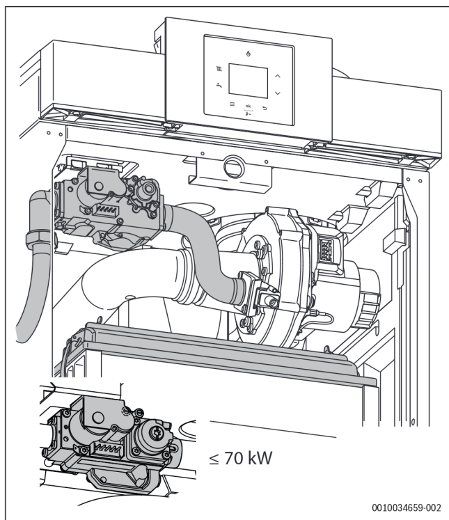
Мал. 36 Огляд газового каналу
