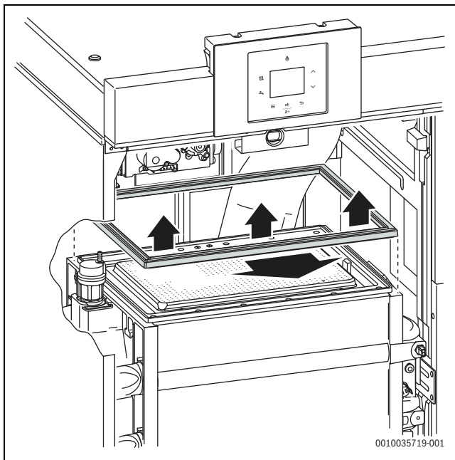
Мал. 42 Зняття ущільнення пальника
