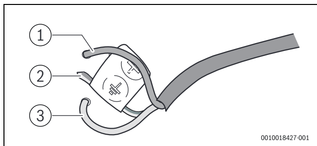
Мал. 31 Приєднання штекера
