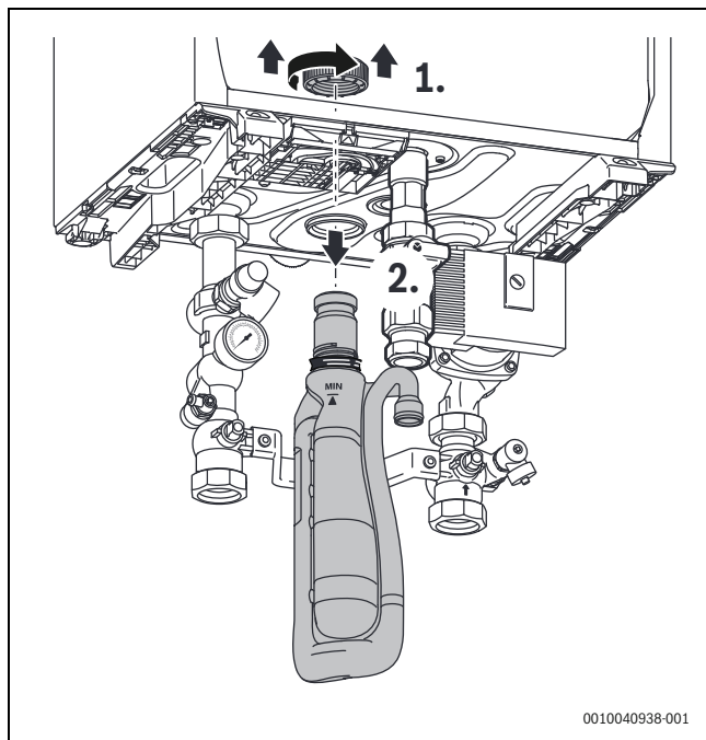
Мал. 45 Демонтаж сифона котла
