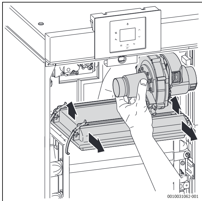
Мал. 41 Зняти газоповітряний блок разом з кришкою пальника.
