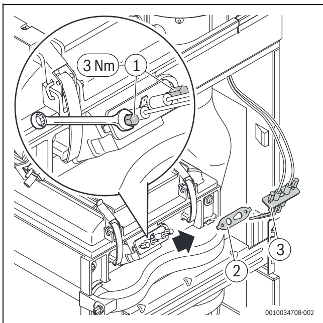
Мал. 48 Встановлення запальника
