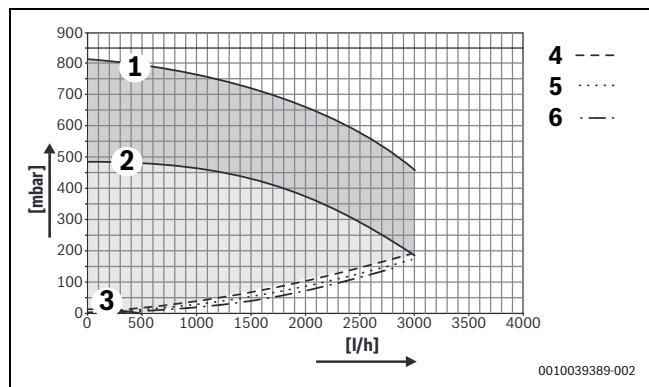
Мал. 52 Залишковий напір насоса GB272-50
