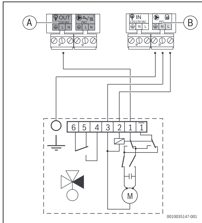
Мал. 29 Схема з'єднань 3-ходового клапана 230 В
