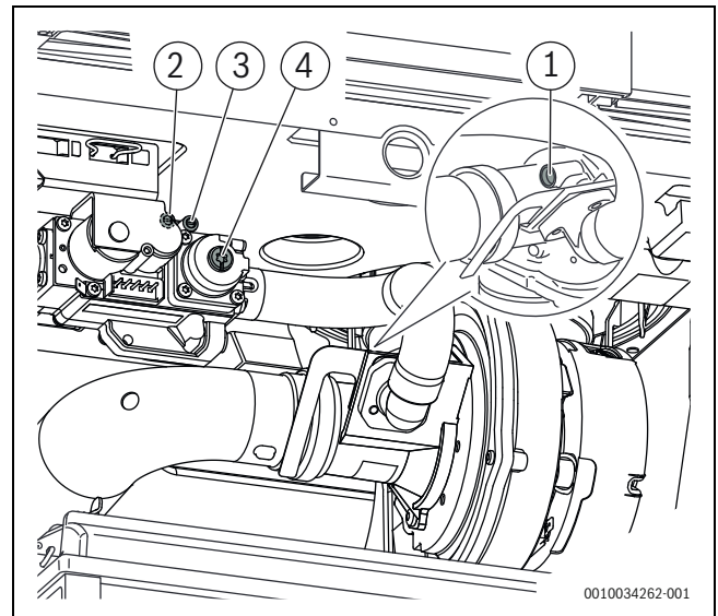
Мал. 32 Огляд штуцерів для вимірювання та регулювальних гвинтів ≤ 70 кВт
