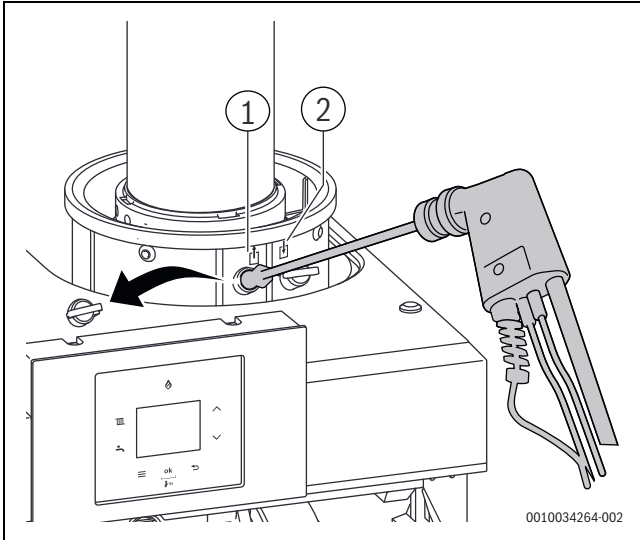
Мал. 34 Зняти заглушку на підключенні до димоходу
