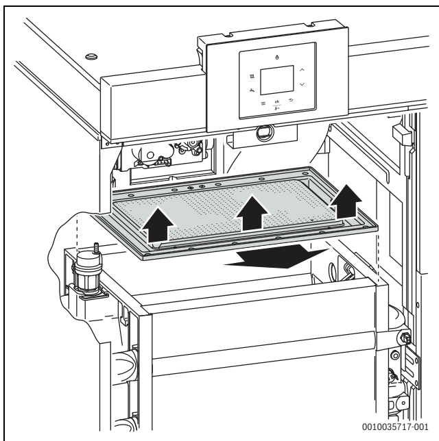
Мал. 43 Зняття пальника
