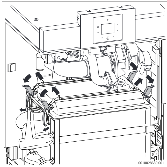
Мал. 40 Відкрити фіксатори
