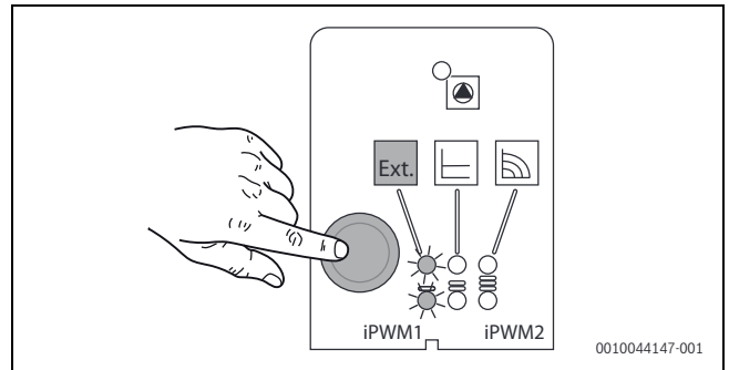
Мал. 27 Налаштування потужності насоса пристроєм ≤ 70 кВт
