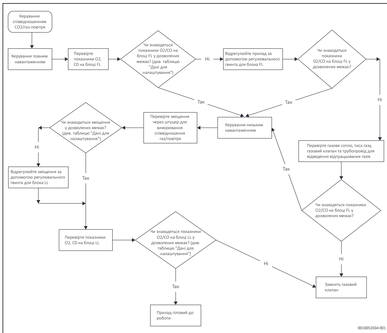
Мал. 35 Блок-схема інструкцій щодо налаштування
