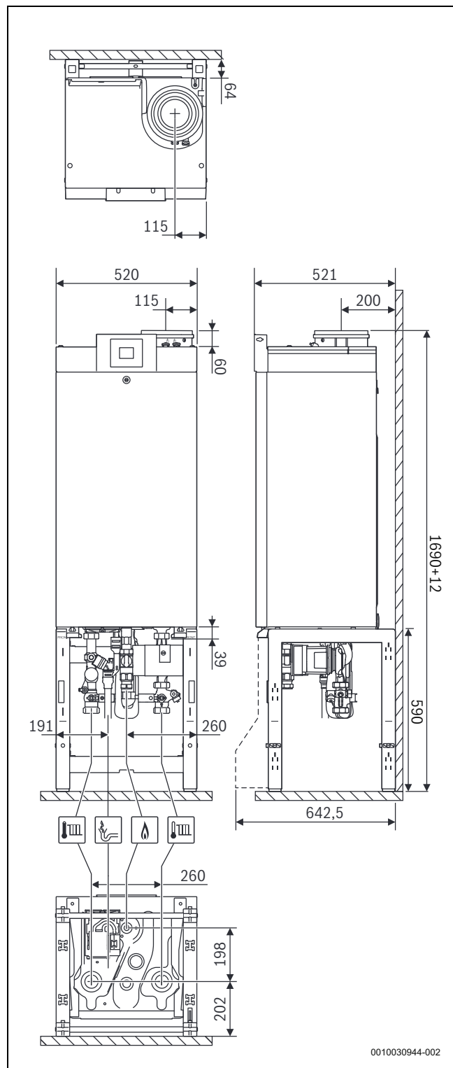
Мал. 2 Розміри на базовій рамі [мм]
