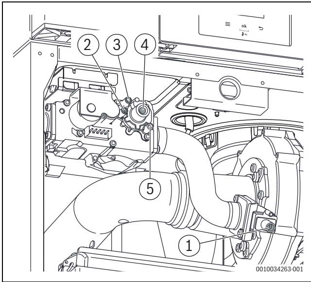
Мал. 33 Огляд штуцерів для вимірювання та регулювальних гвинтів \geq 85 кВт
