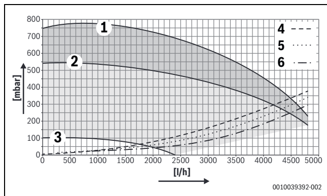
Мал. 55 Залишковий напір насоса GB272-100
