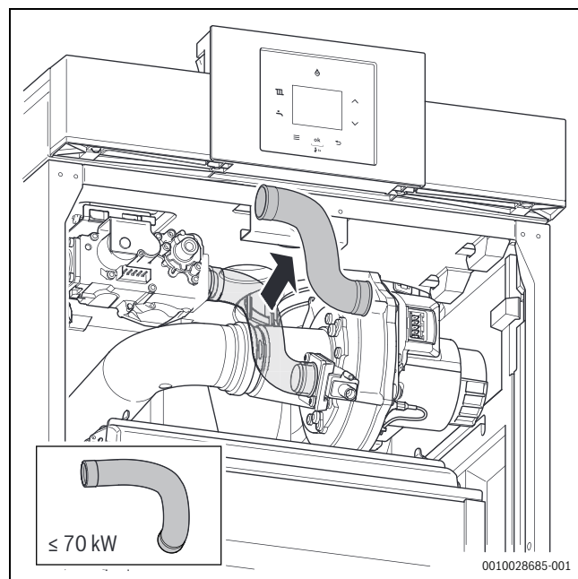
Мал. 38 Демонтаж газового шланга ≥ 85 кВт
