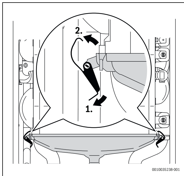
Мал. 46 Відкривання фіксаторів конденсатовловлювача
