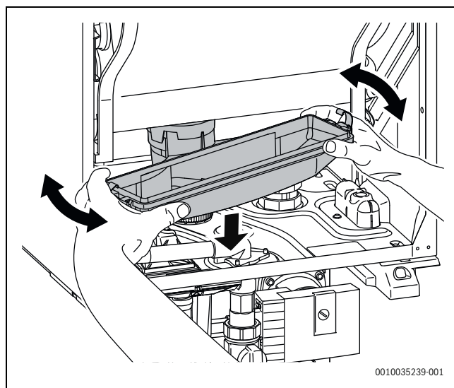
Мал. 47 Демонтувати конденсатовловлювач.
