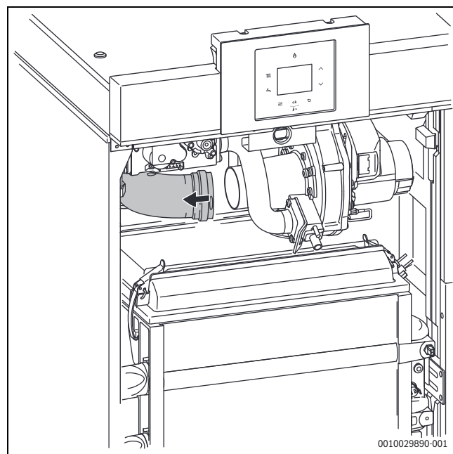
Мал. 39 Демонтаж повітрязабірної труби
