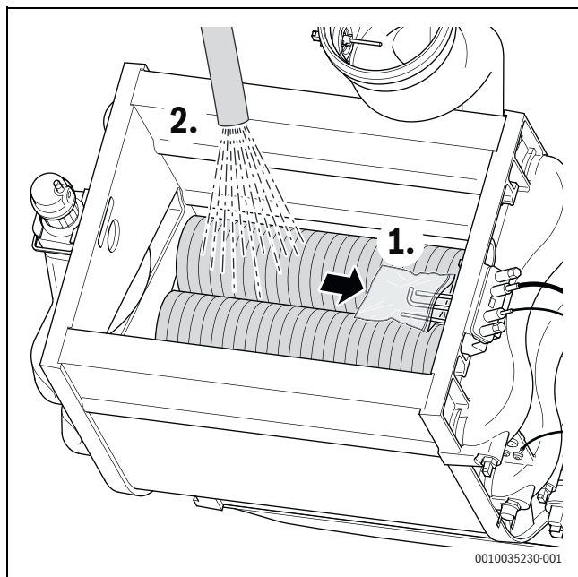
Мал. 44 Чищення теплообмінника
