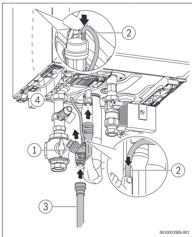
Мал. 17 Монтаж шланга розповітрявача
