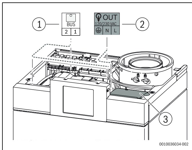
Мал. 30 Встановлення функціонального модуля
