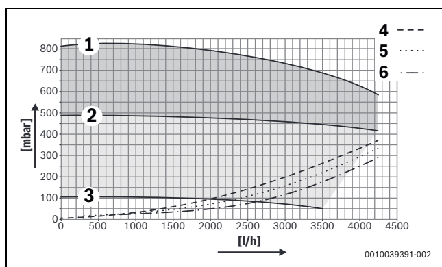
Мал. 54 Залишковий напір насоса GB272-85
