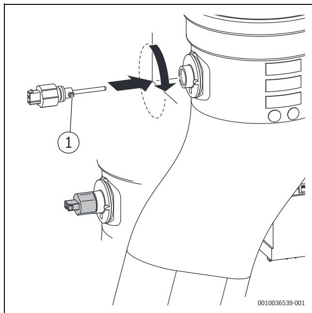
Мал. 49 Заміна датчика температури відпрацьованих газів
