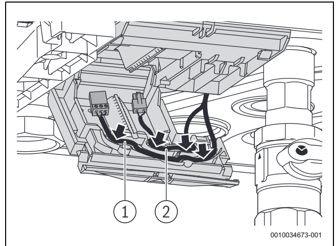
Мал. 26 Підключення насоса
