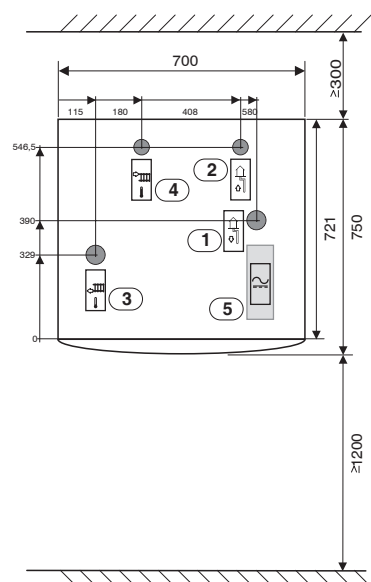
Przyłącza i odległości montażowe pomp ciepła (38–48 kW)
