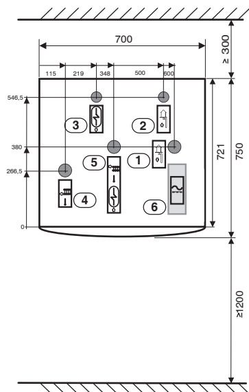
Przyłącza i odległości montażowe pomp ciepła (22–28 kW)
