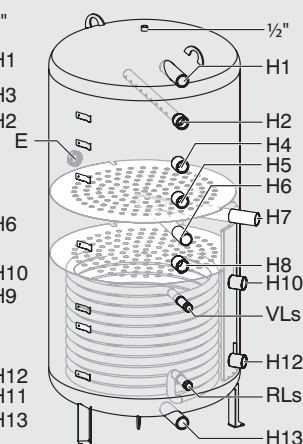
PNRZ 750, 1000.6 E(W)
