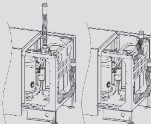
Podłączenie boczne lub górne/boczne za pomocą węży elastycznych
