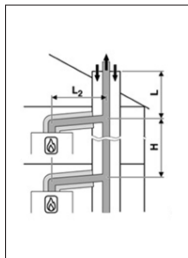
Wykorzystanie wielokrotnego typu C(14)3x ze wspólnym odprowadzaniem spalin
