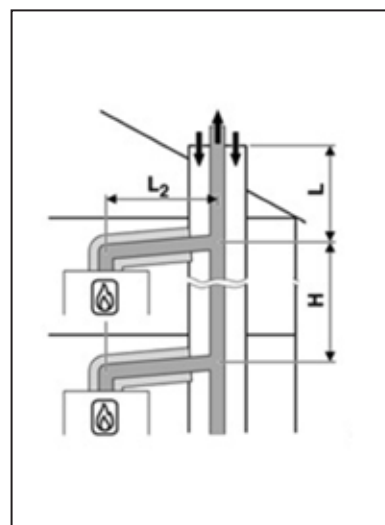
Wykorzystanie wielokrotność typu C(14)3x ze wspólnym odprowadzaniem spalin
