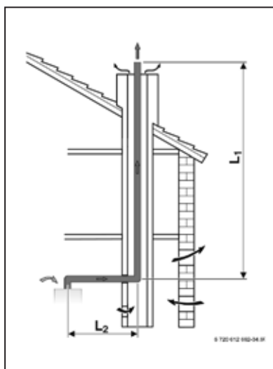
Odprowadzenie spalin w szachcie typu B 23p
