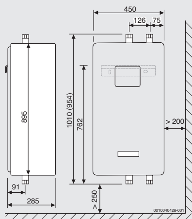
Wymiary i minimalne odstępy, w mm (wartość w nawiasie dla SLP2/3 E)
