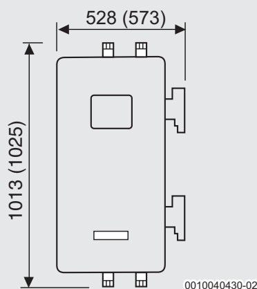
SLP3/3 E i SLP4/3 E (wartość w nawiasie = SLP4/3 E),
