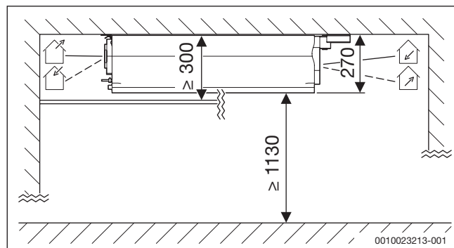
Rys. 3 Wymiary i minimalne odstęp instalacji podsufitowej Logavent
