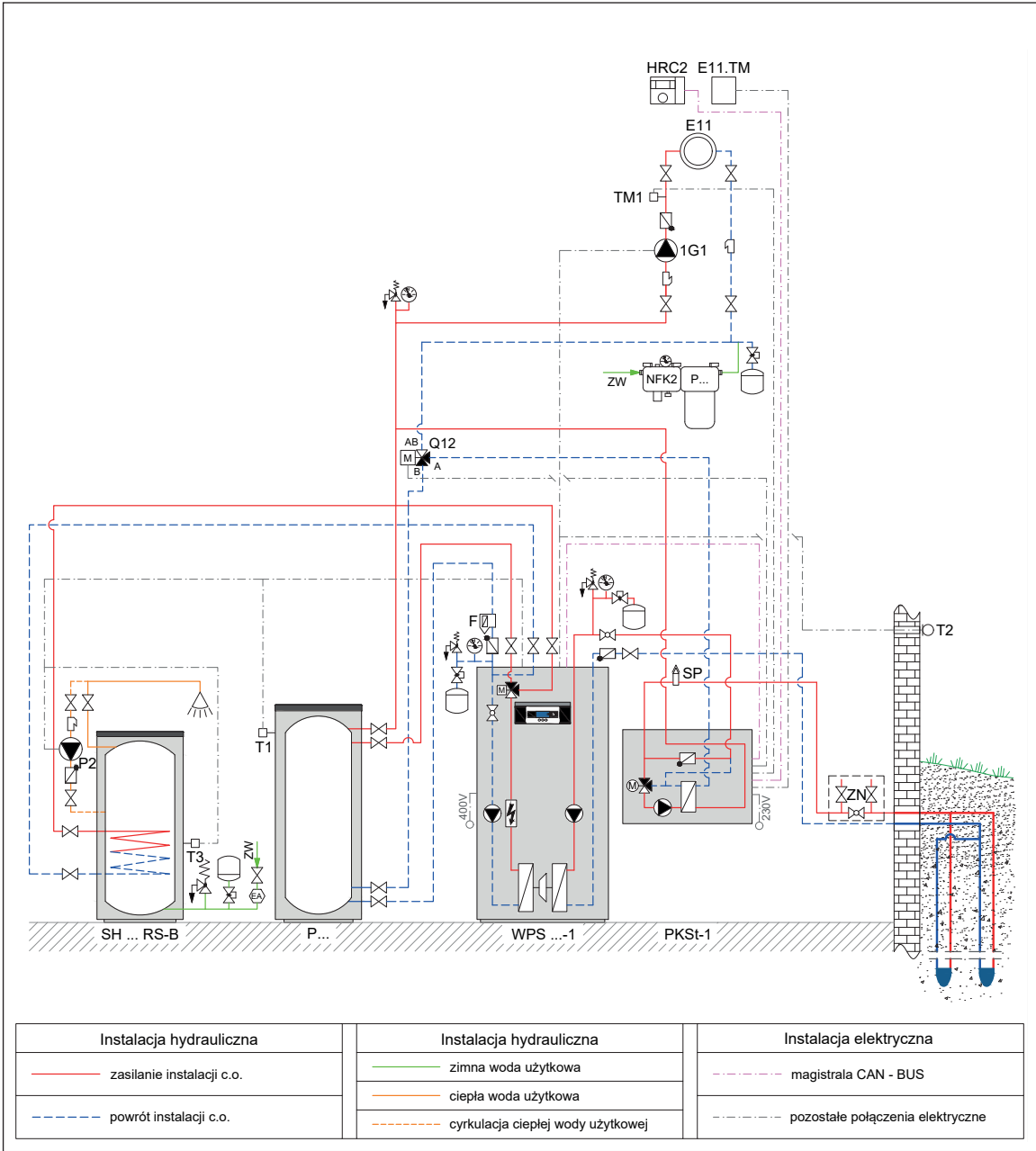
Rys. 165 Schemat hydrauliczny
