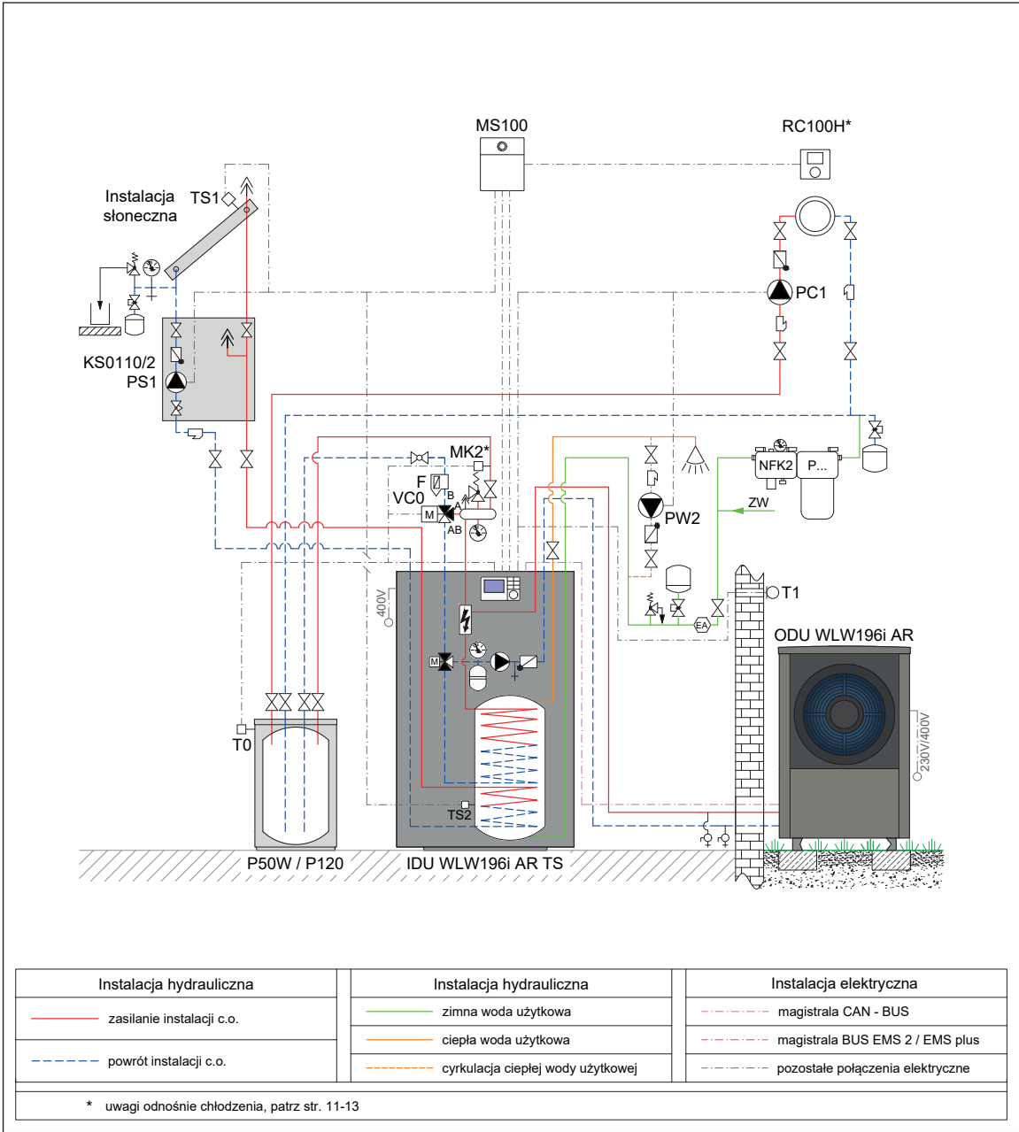
Rys. 79 Schemat hydrauliczny
