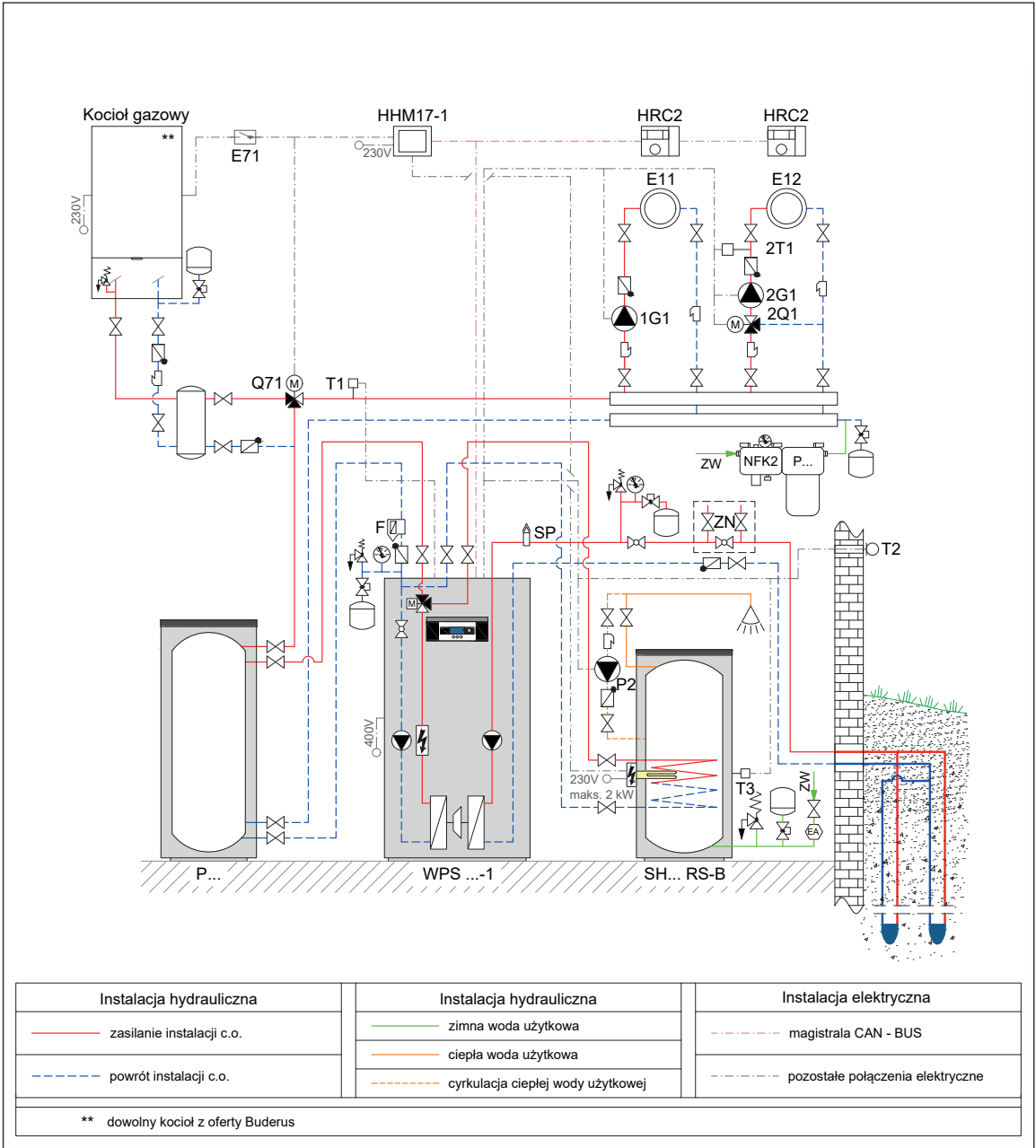
Rys. 161 Schemat hydrauliczny
