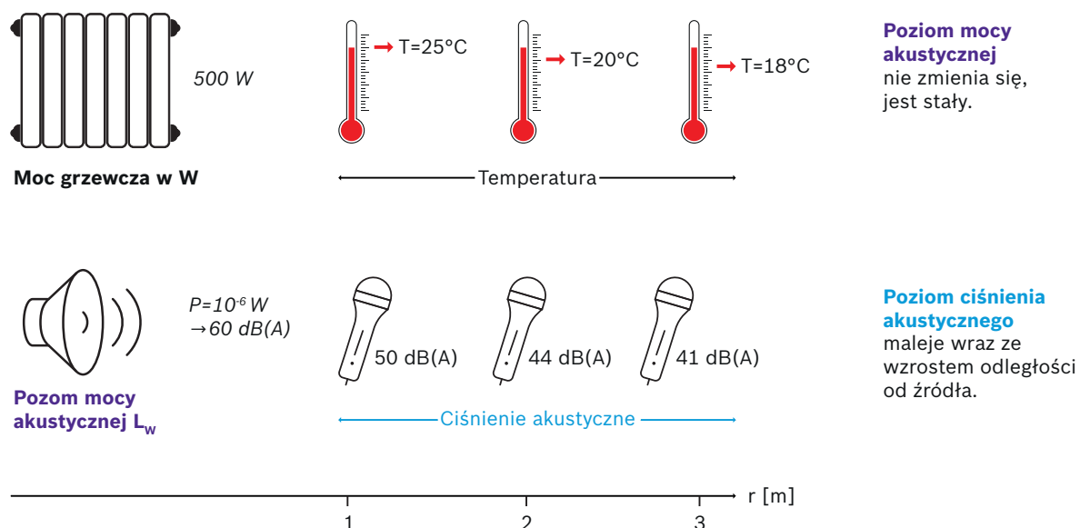
Rys. 12 Różnice w poziomie mocy akustycznej i poziomie ciśnienia akustycznego
