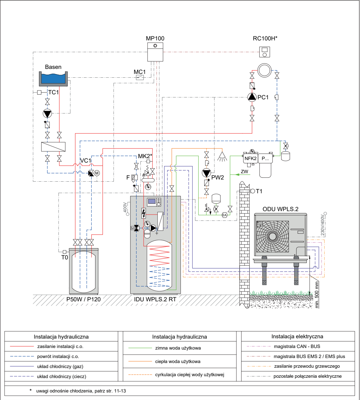
Rys. 131 Schemat hydrauliczny
