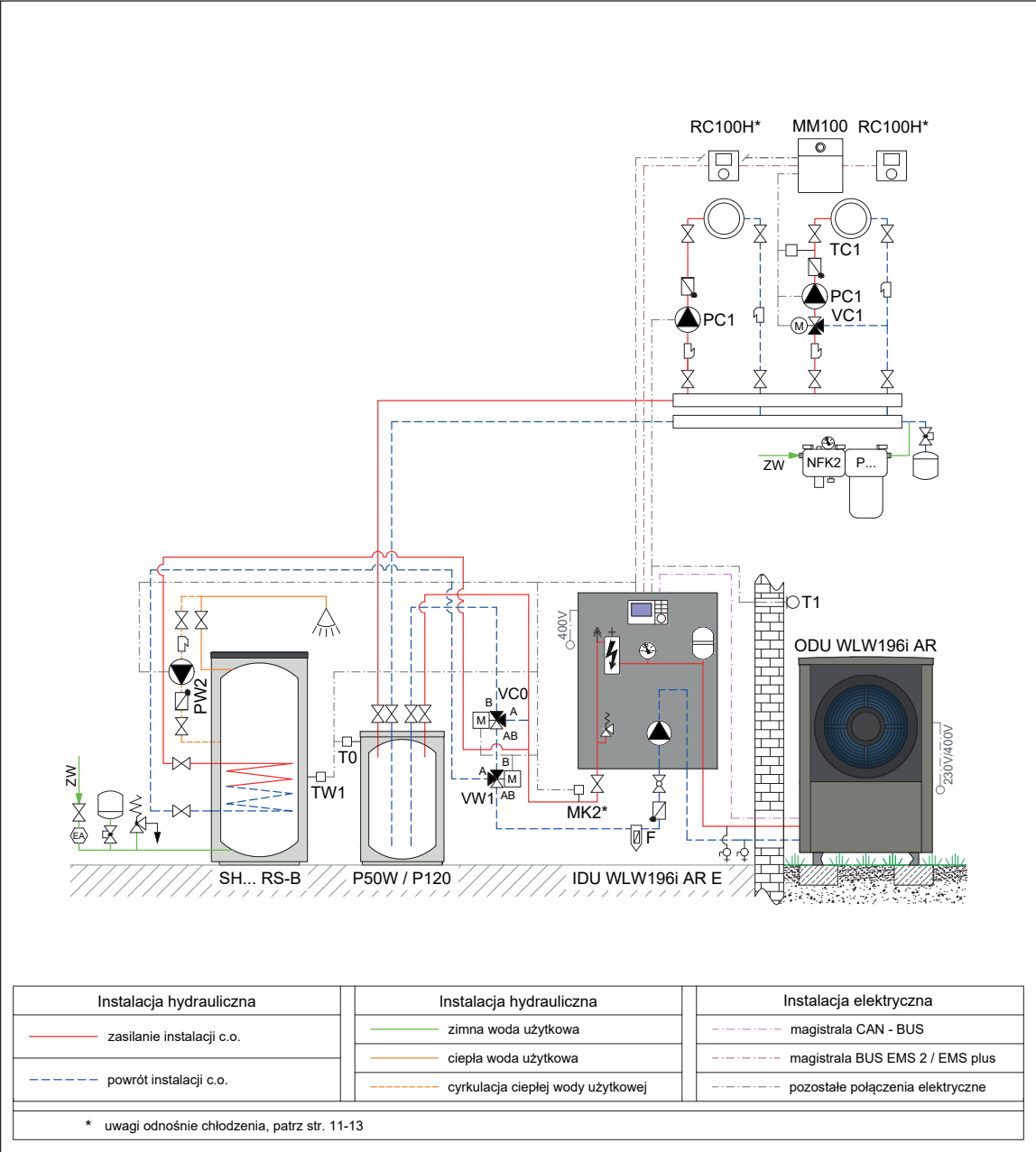
Rys. 39 Schemat hydrauliczny
