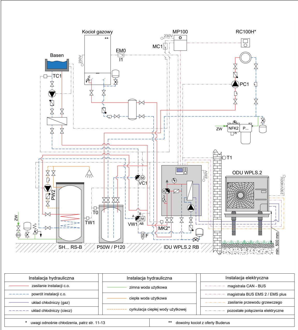
Rys. 117 Schemat hydrauliczny
