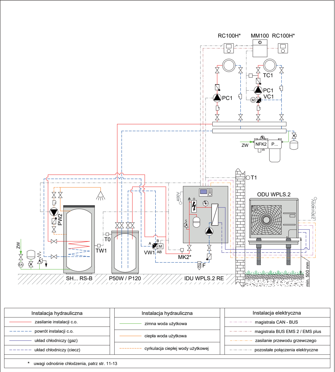
Rys. 93 Schemat hydrauliczny
