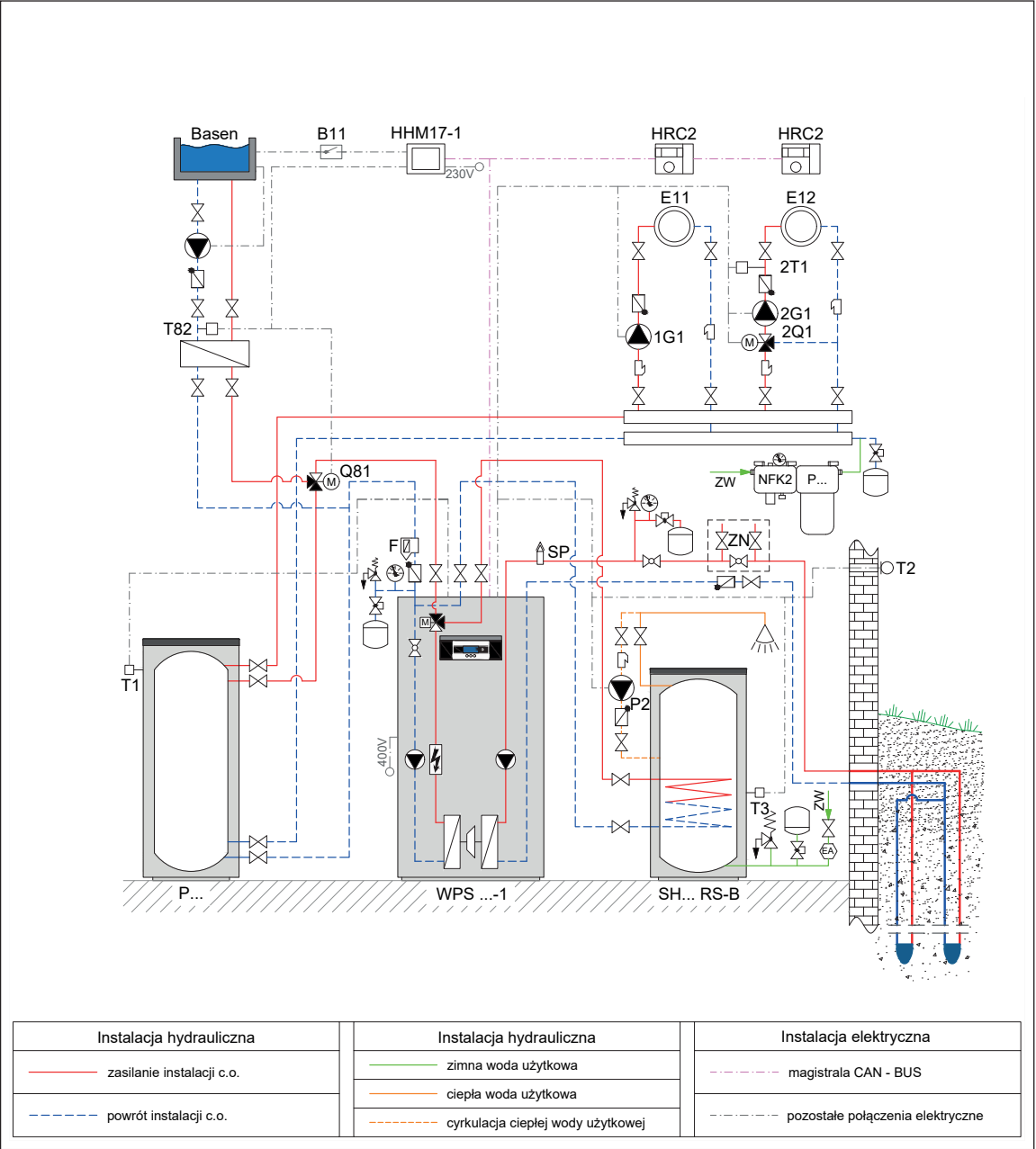
Rys. 163 Schemat hydrauliczny
