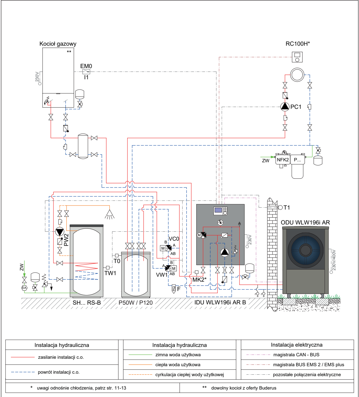
Rys. 57 Schemat hydrauliczny
