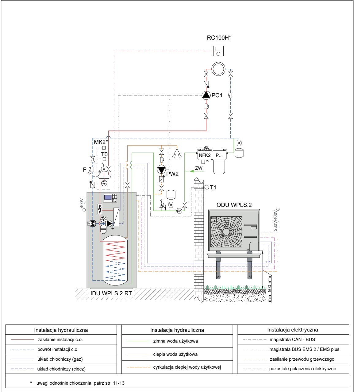
Rys. 123 Schemat hydrauliczny
