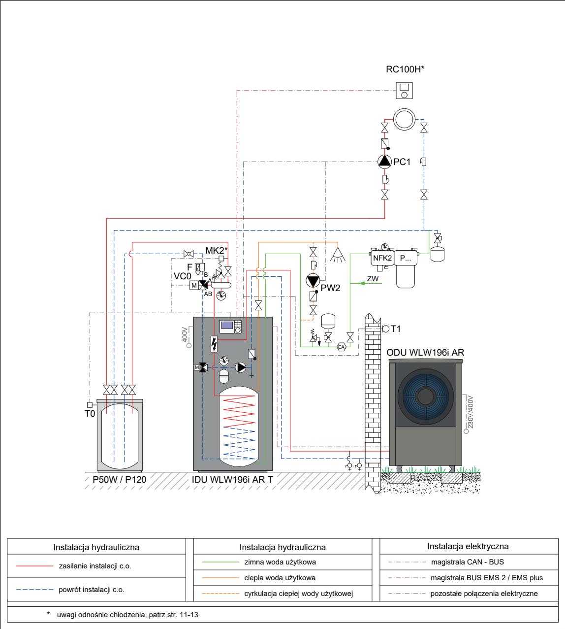
Rys. 69 Schemat hydrauliczny
