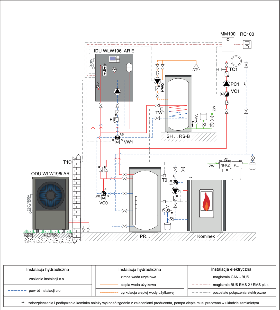
Rys. 43 Schemat hydrauliczny
