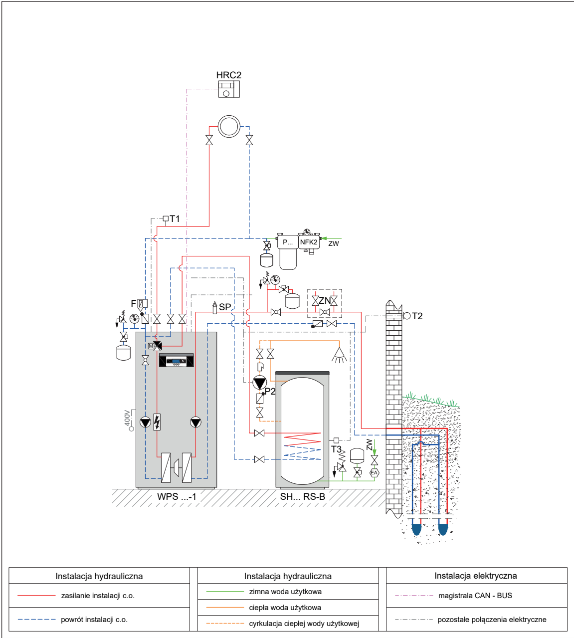
Rys. 153 Schemat hydrauliczny
