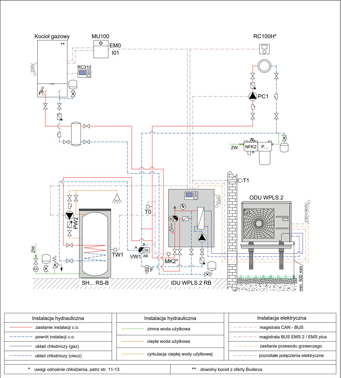
Rys. 109 Schemat hydrauliczny
