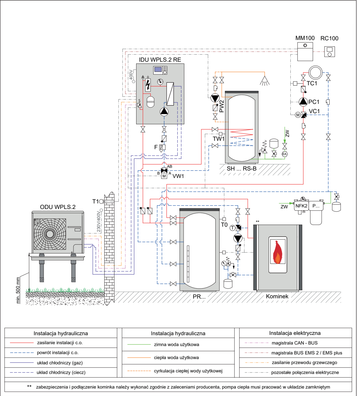
Rys. 97 Schemat hydrauliczny
