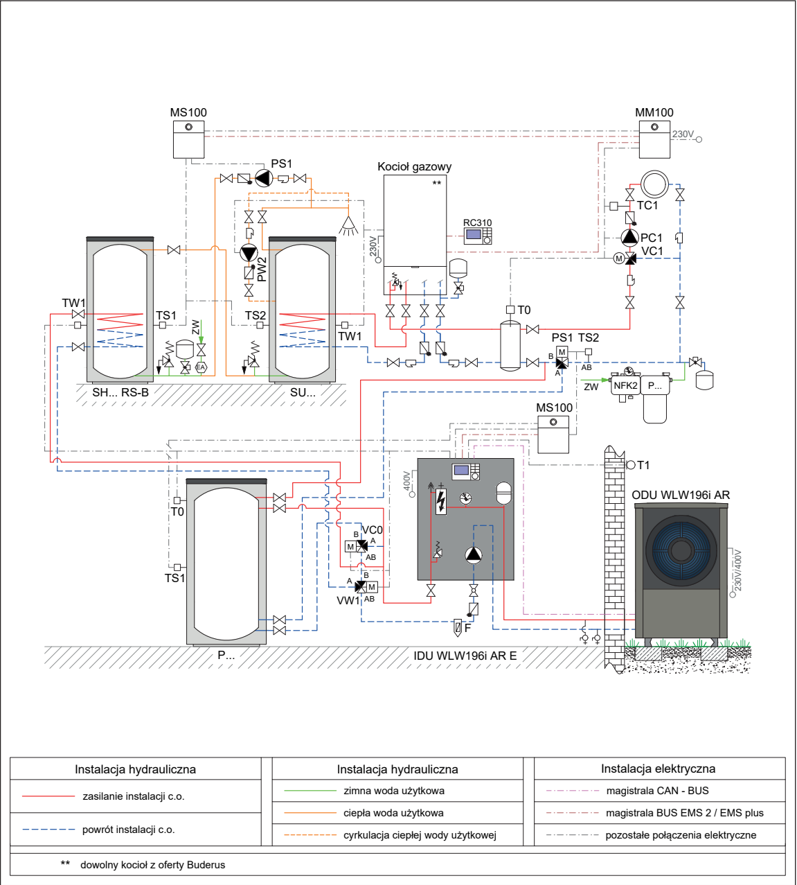
Rys. 49 Schemat hydrauliczny
