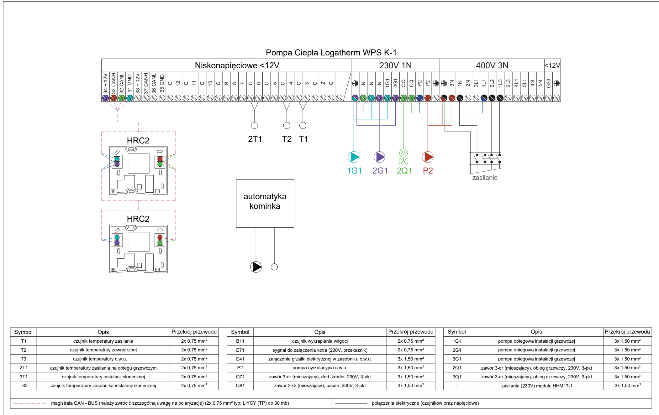
Rys. 152 Schemat elektryczny
