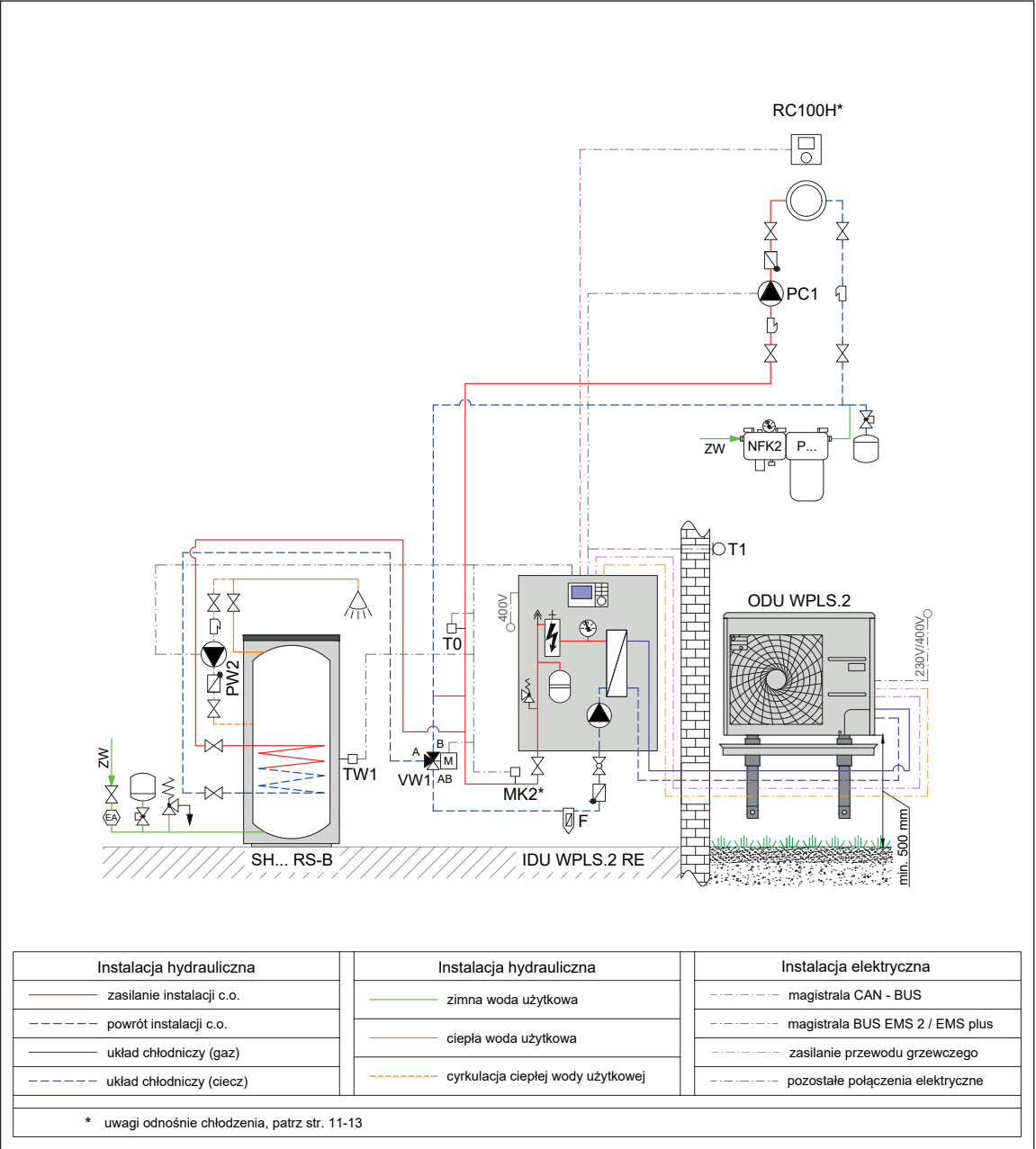
Rys. 87 Schemat hydrauliczny
