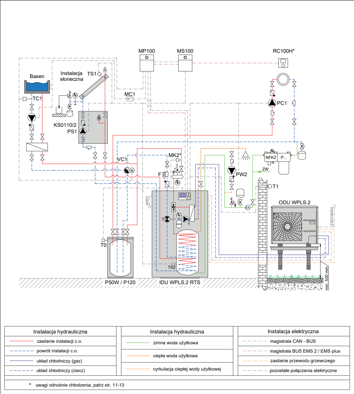
Rys. 143 Schemat hydrauliczny
