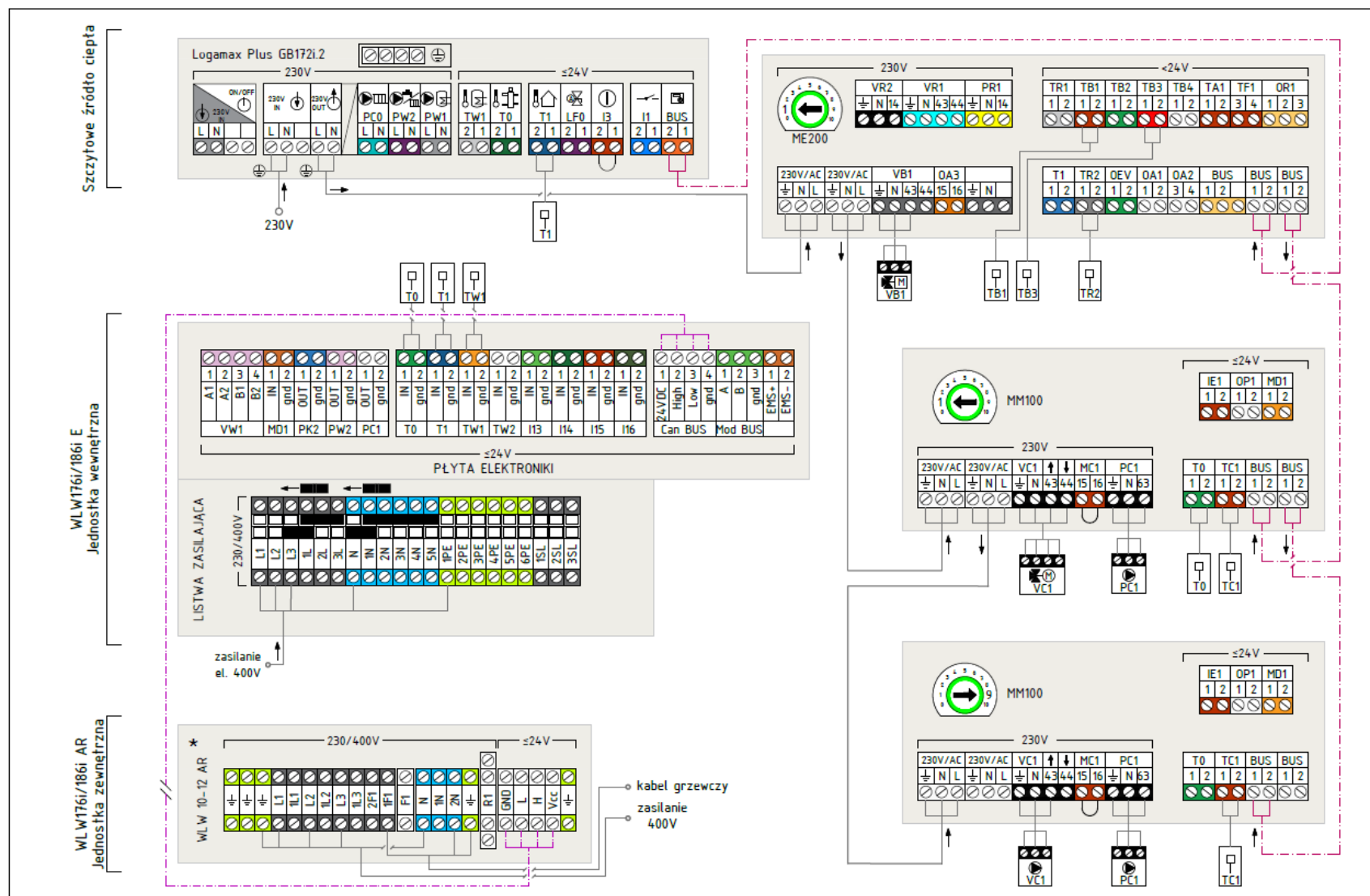
Schemat 1.3: WLW176i/186i AR E - instalacja ze zbiornikiem buforowym, współpraca z kotłem Buderus (moduł ME200), CWU z kotła
