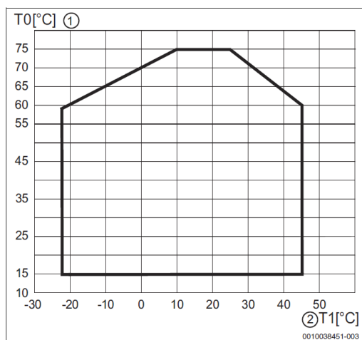
Rys. 7. Pompa ciepła w trybie grzania, bez dogrzewacza.
