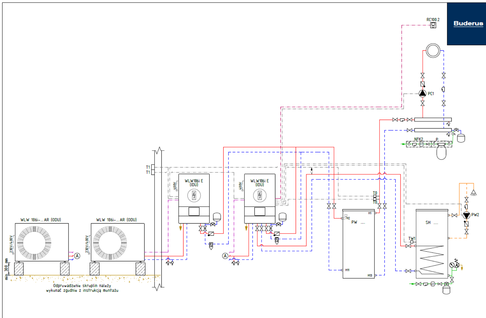
Schemat 1.6: WLW176i/186i AR E – kaskada hydrauliczna ze wspólnym zbiornikiem buforowym, CWU z jednej pompy ciepła
