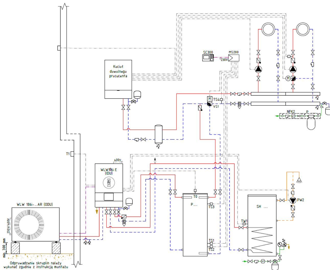
Schemat 1.4: WLW176i/186i AR E - instalacja ze zbiornikiem buforowym, współpraca z obcym kotłem (moduł MS200)
