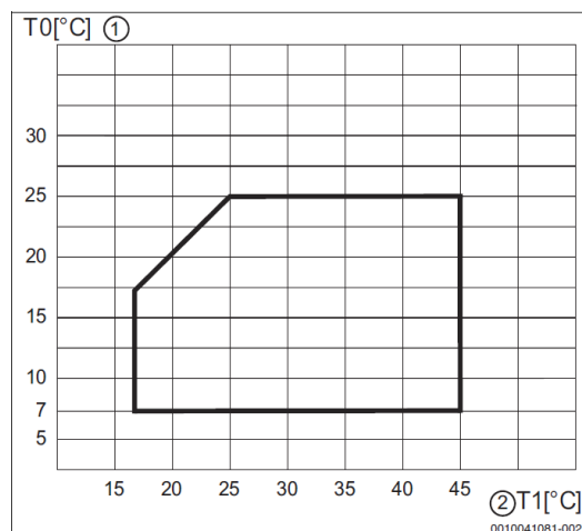
Rys. 8. Pompa ciepła w trybie chłodzenia.
