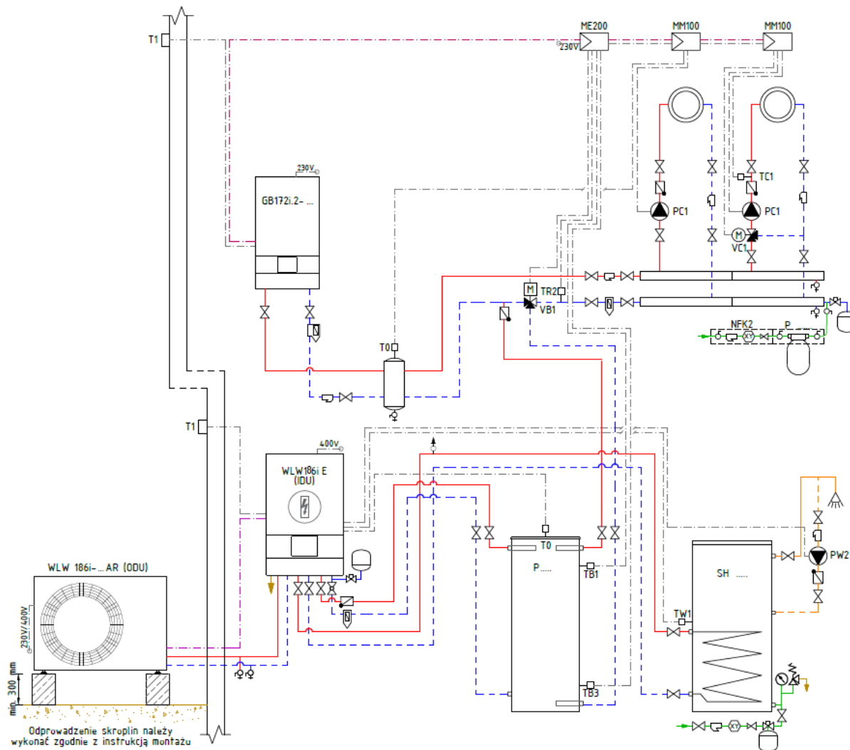
Schemat 1.2: WLW176i/186i AR E - instalacja ze zbiornikiem buforowym, współpraca z kotłem Buderus (moduł ME200), CWU z pompy ciepła
