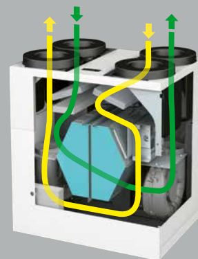
Vysoký komfort vďaka integrovanému letnému bypassu
