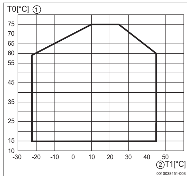
Rys. 45 Pompa ciepła w trybie grzania, bez dogrzewacza
