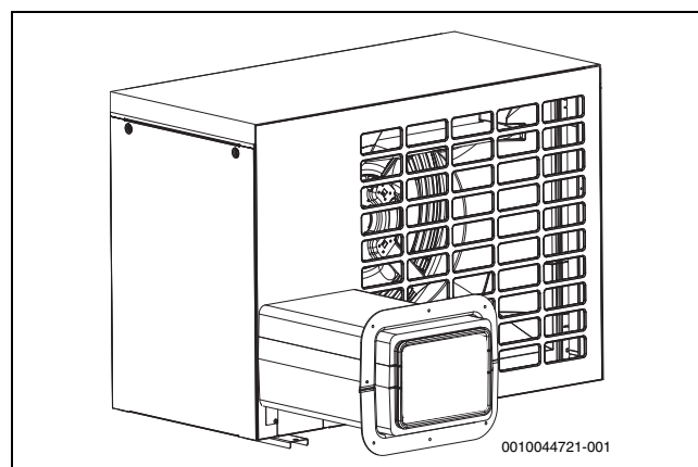
Rys. 24 Zestaw montażowy, zawieszenie na ścianie
