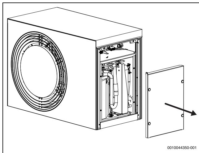
Rys. 34 Pokrywa zbiornika czynnika chłodniczego
