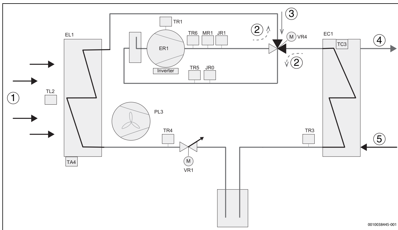
Rys. 47 Obieg czynnika chłodniczego
