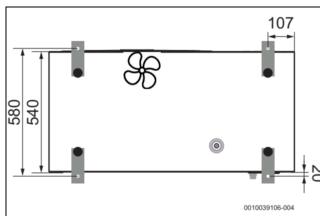
Rys. 5 Wymiary pompy ciepła, górna część
