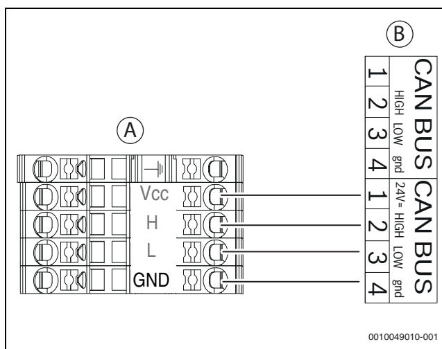
Rys. 36 Magistrala CAN-BUS pompy ciepła – jednostka wewnętrzna
