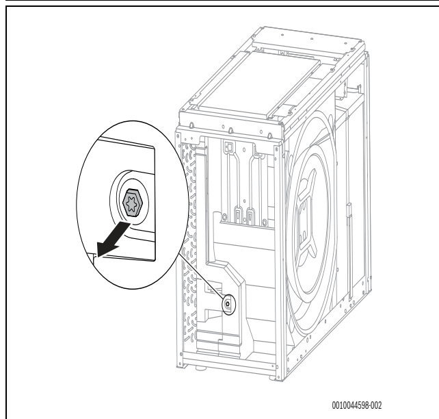
Rys. 42 Odkręcanie
