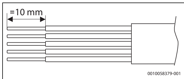
Rys. 40 Usuwanie izolacji z przewodu zasilania sieciowego
