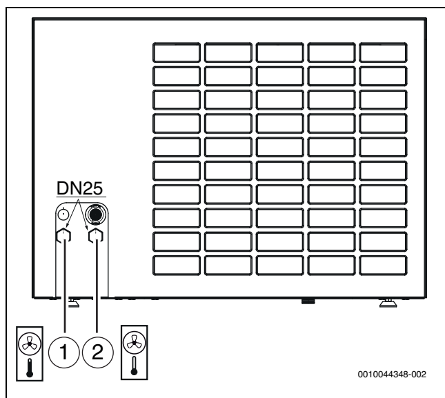
Rys. 32 Łączniki rurowe nośnika ciepła; opis dotyczy wszystkich rozmiarów
