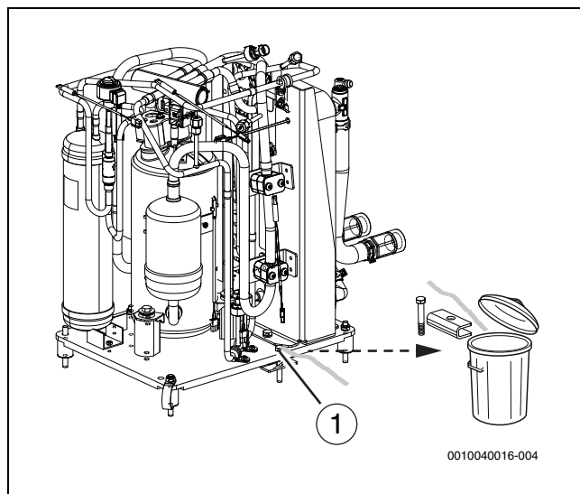
Rys. 35 Śruba transportowa
