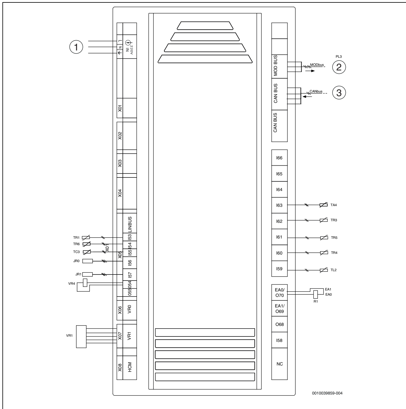
Rys. 49 Schemat elektryczny XCU-SRH (XCU-HP)
