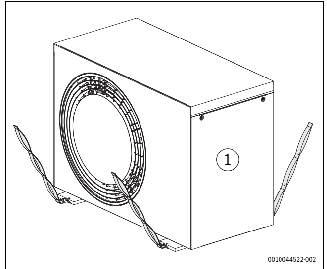
Rys. 11 Używanie pasów do transportu pompy ciepła bez opakowania
