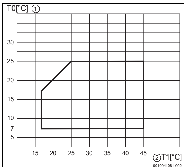
Rys. 46 Pompa ciepła w trybie chłodzenia
