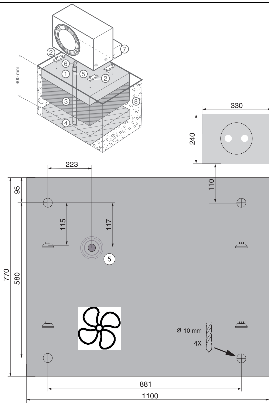
Rys. 31 Plan fundamentów, alternatywa 2
