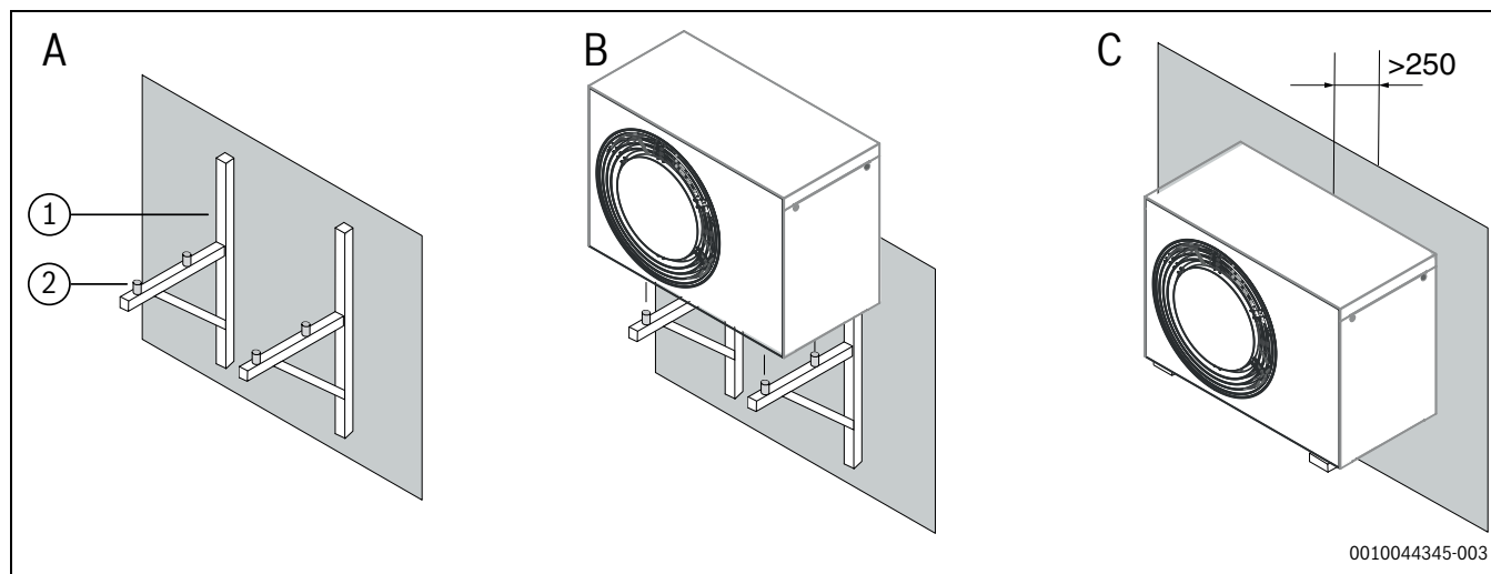
Rys. 25 Jednostka zewnętrzna zamocowana do ściany (mm)
