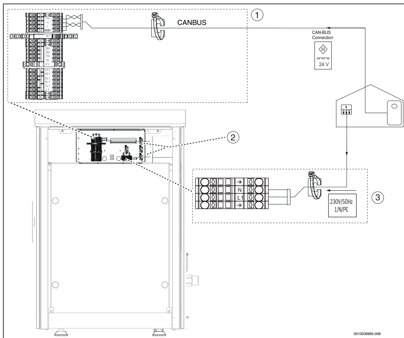
Rys. 39 Skrzynka zaciskowa
