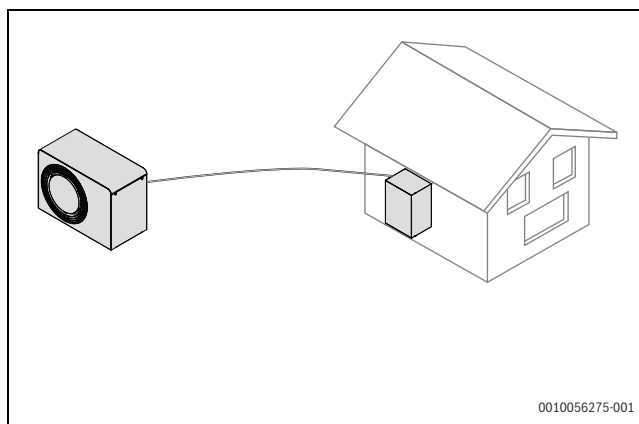
Rys. 37 Połączenie CAN-BUS między jednostką wewnętrzną a jednostką zewnętrzną
