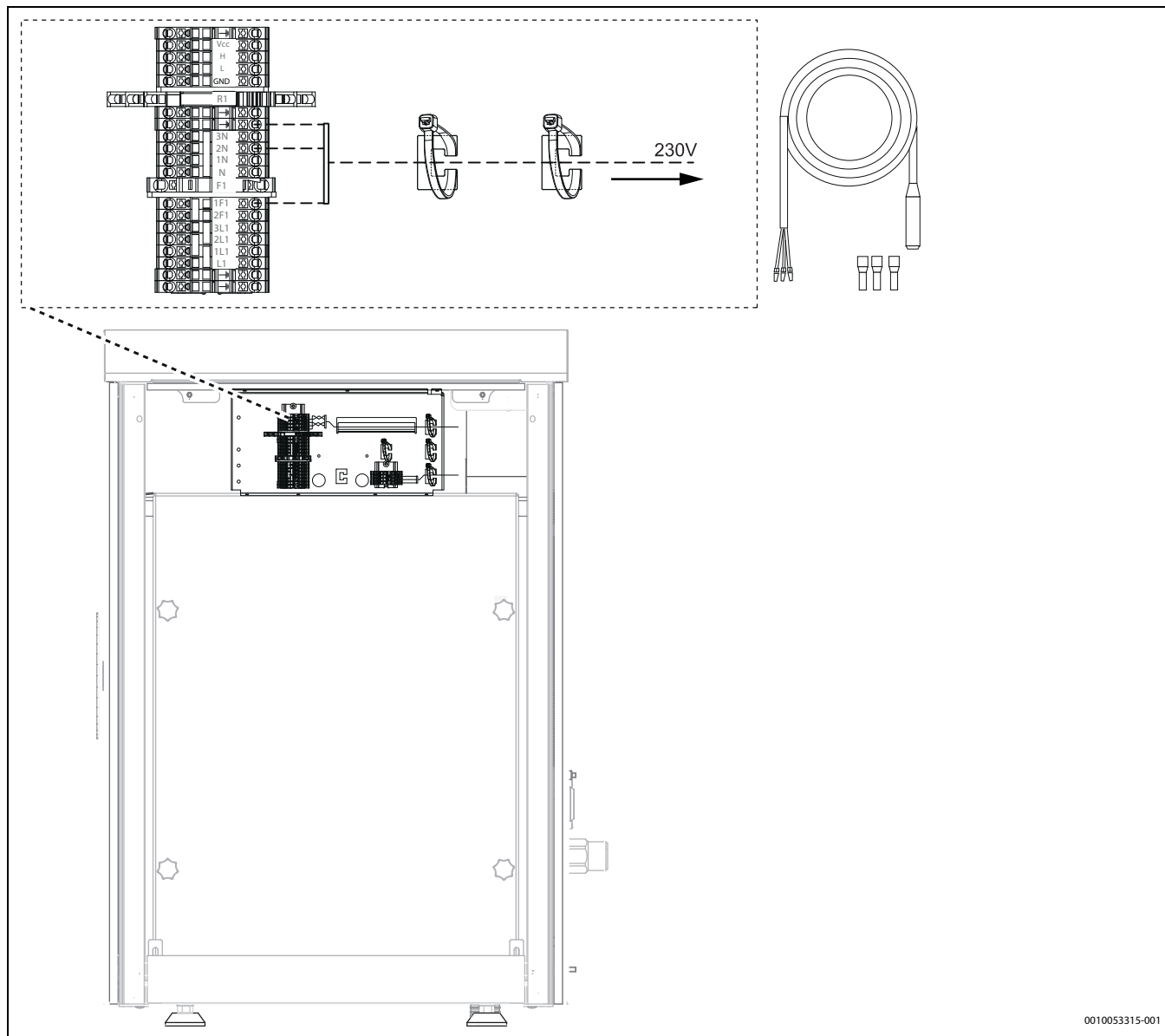
Rys. 41 Przyłącze kabla grzewczego (osprzęt)
