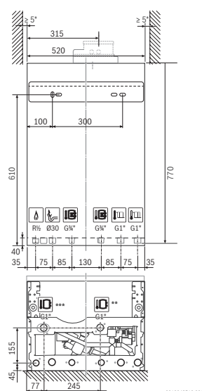
Logamax plus GB192i.2-15 H, GB192i.2-25 H
