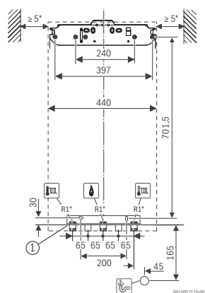
Logamax plus GB182i.2-45 H
