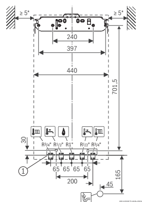
Logamax plus GB182i.2-15 H, GB182i.2-25 H, GB182i.2-30 H
