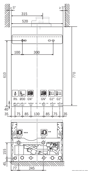
Logamax plus GB192i.2-15 H, GB192i.2-25 H
