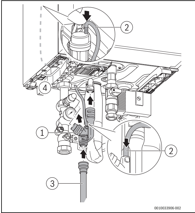
Res. 17 Hava pürjörü hortumunun monte edilmesi
