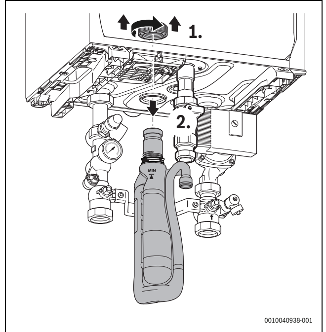
Res. 42 Kazan sifonunun çıkarılması
