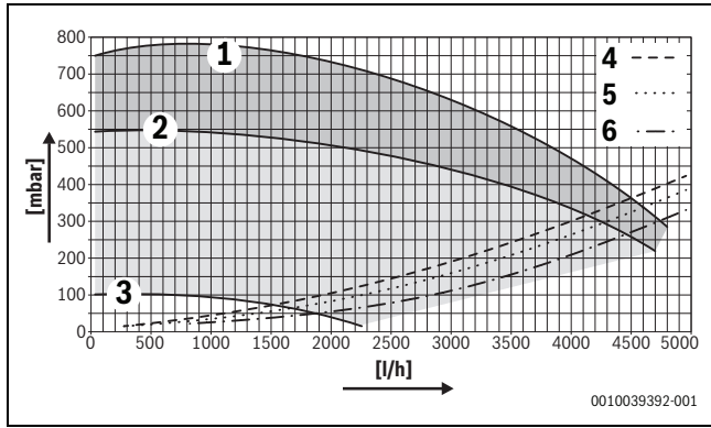
Res. 49 Pompanın kalan pompalama yüksekliği GB272-100
