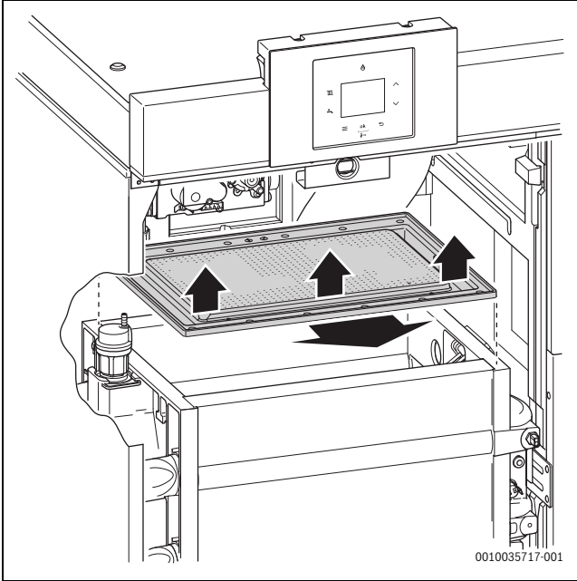
Res. 40 Brülörün çıkarılması
