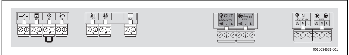
Res. 23 Soket panosuna genel bakış
