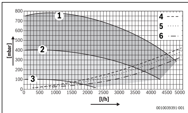
Res. 50 Pompanın kalan pompalama yüksekliği GB272-85
