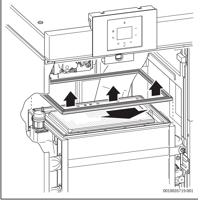
Res. 39 Brülör contasının çıkarılması
