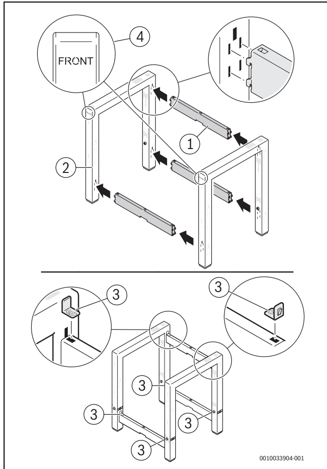
Res. 8 Yer kitinin monte edilmesi
