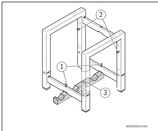
Res. 9 Yer kitinin duvara veya zemine sabitlenmesi
