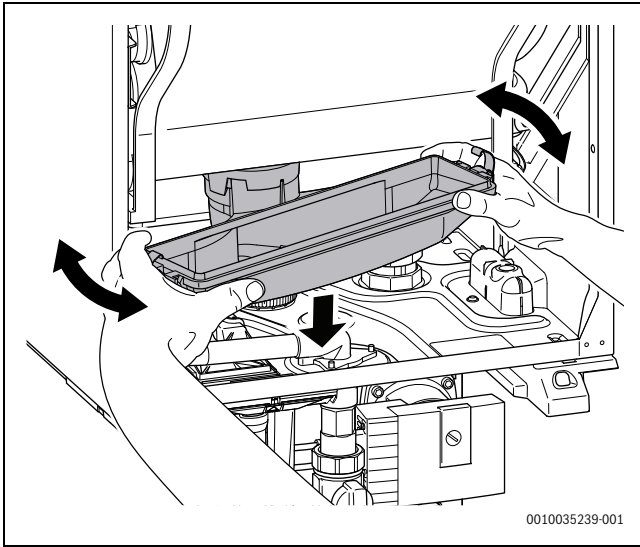
Res. 44 Yoğuşma suyu kabının çıkarılması
