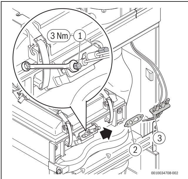
Res. 45 Ateşleme çubuğunun değiştirilmesi
