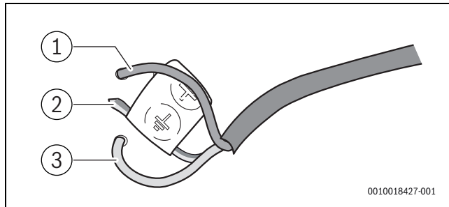
Res. 29 Soketin monte edilmesi
