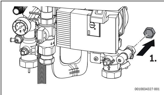
Res. 20 Bir genleşme tankının bağlanması
