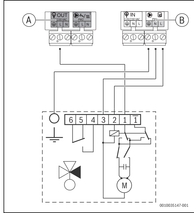
Res. 27 230 V 3 yollu vananın bağlantı planı
