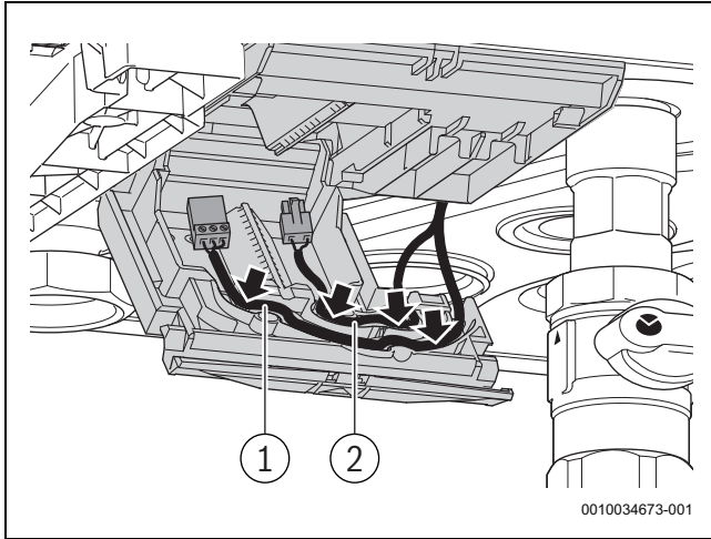
Res. 26 Pompanın bağlanması
