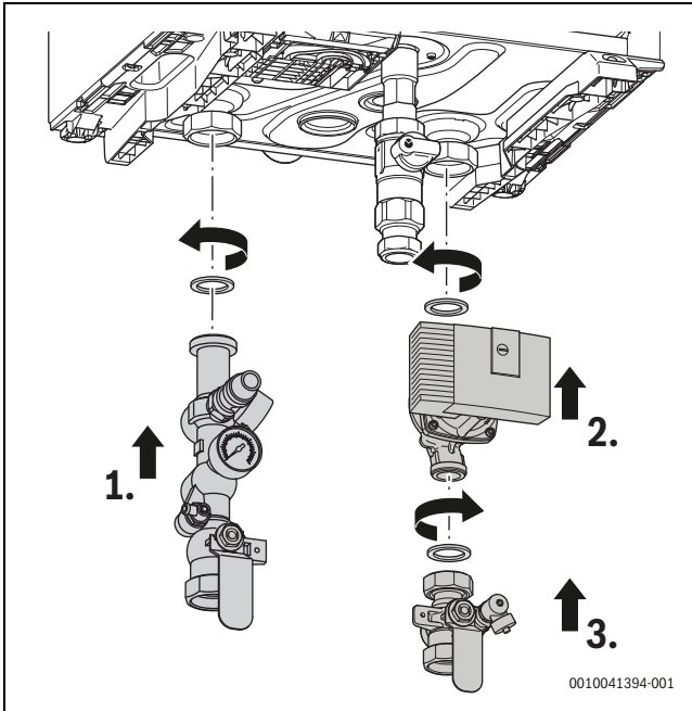
Res. 14 Gidiş suyu ve dönüş suyu bağlantısının monte edilmesi
