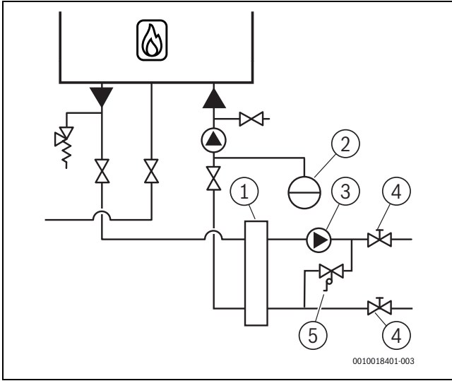
Res. 19 Hidrolik denge kabı ile kurulum
