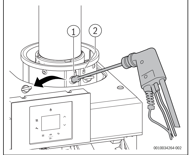
Res. 32 Atık gaz çıkışındaki dübelin çıkarılması
