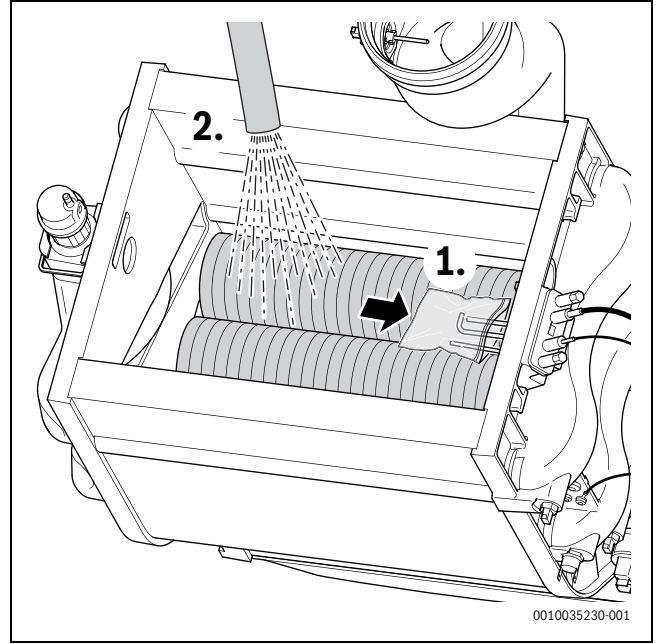
Res. 41 Eşanjörün temizlenmesi
