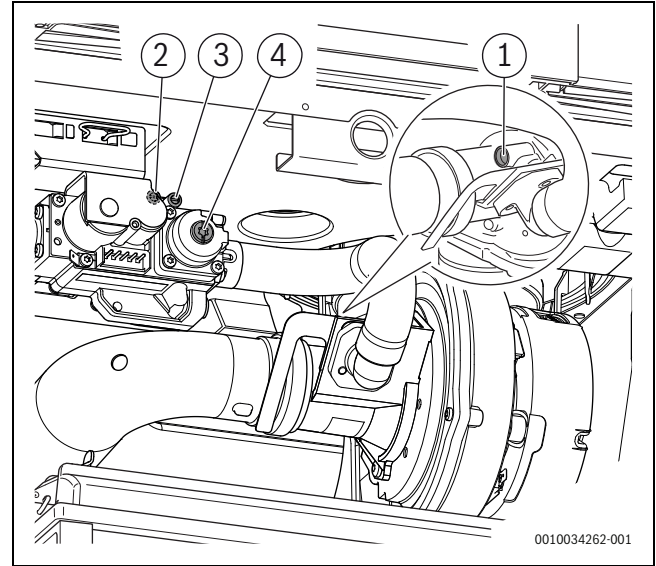
Res. 30 Ölçüm bağlantı ağzlarına ve ≤ 70 kW ayar vidalarına genel bakış
