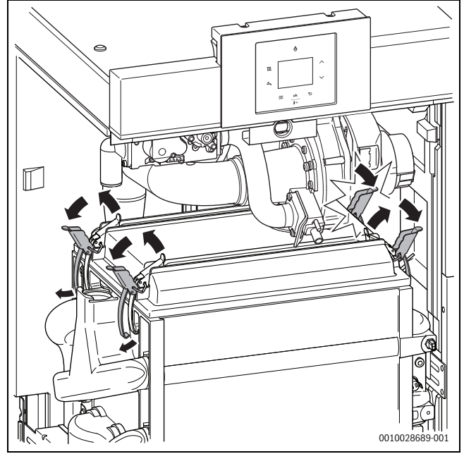
Res. 37 Hızlı kenetlemeli kilitlerin açılması
