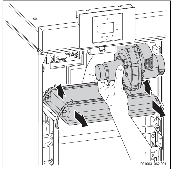
Res. 38 Gaz-hava ünitesini brülör kapağı ile birlikte çıkarın
