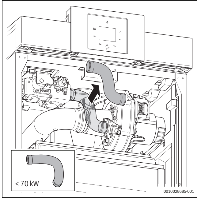
Res. 35 Gaz hortumunun \geq 85 kW çıkarılması
