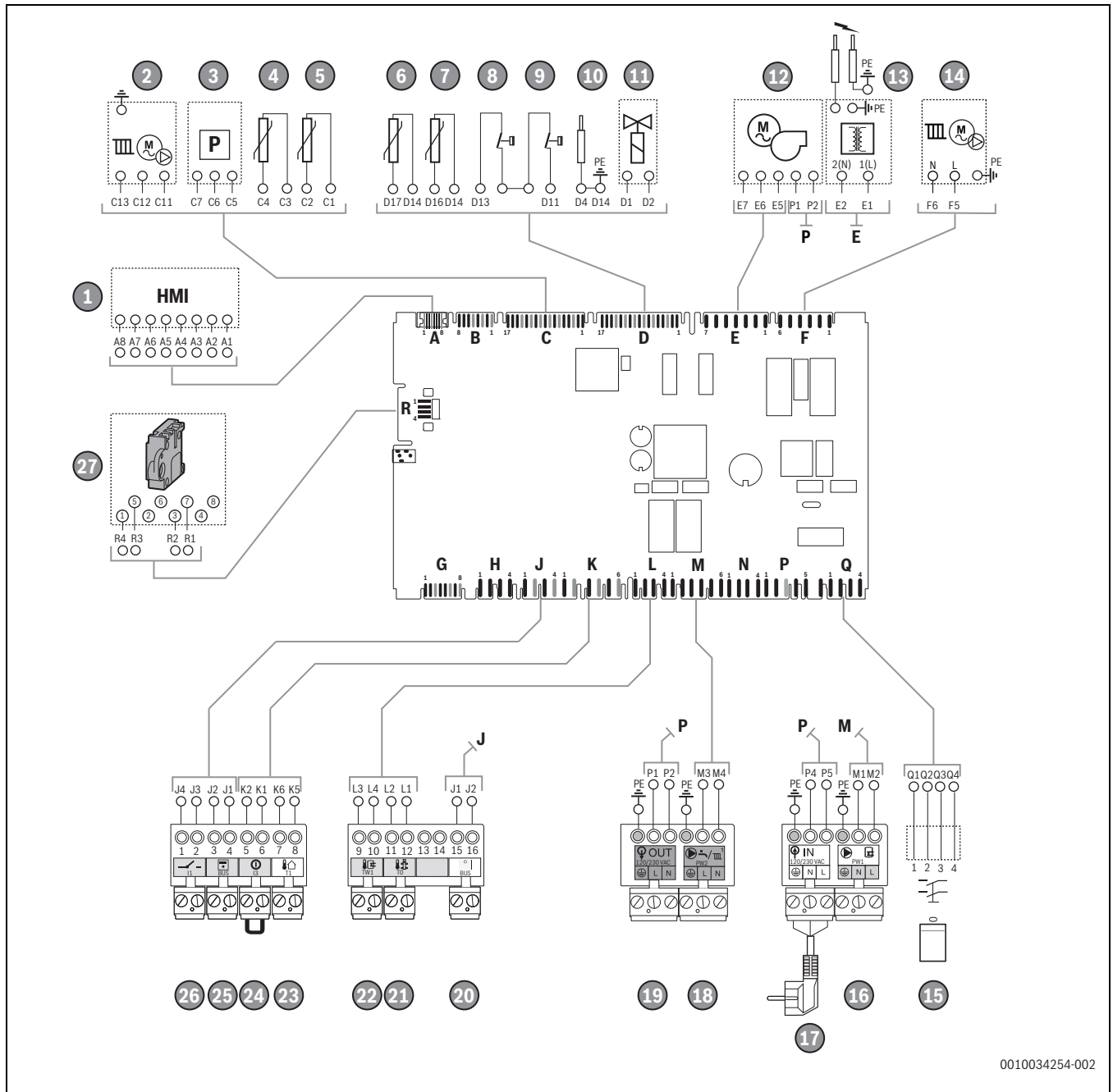
Res. 48 Devre şeması
