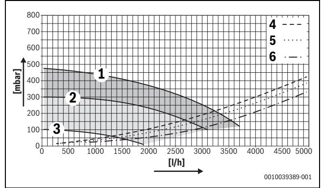
Res. 52 Pompanın kalan pompalama yüksekliği GB272-49
