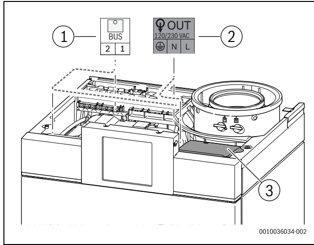
Res. 28 Fonksiyon modülünün monte edilmesi
