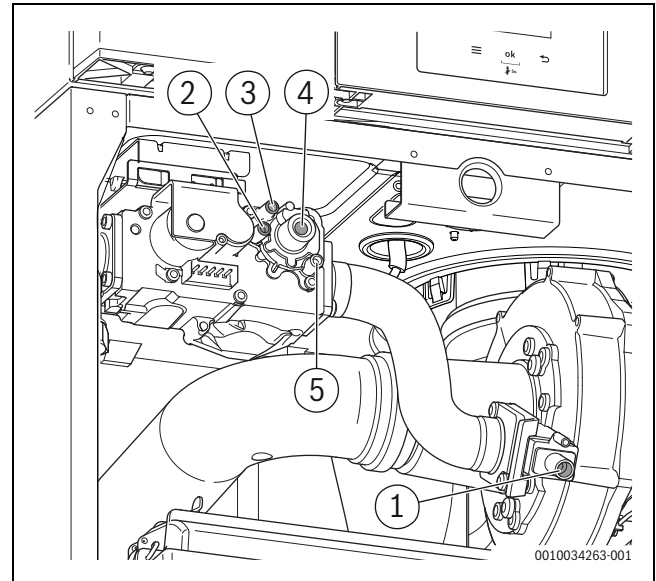
Res. 31 Ölçüm bağlantı ağzlarına ve ≥ 85 kW ayar vidalarına genel bakış
