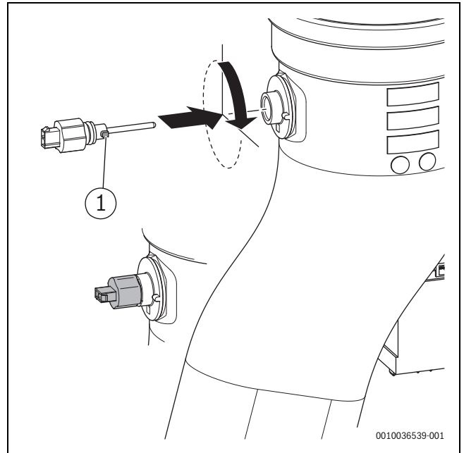
Res. 46 Atık gaz sıcaklık sensörünün değiştirilmesi
