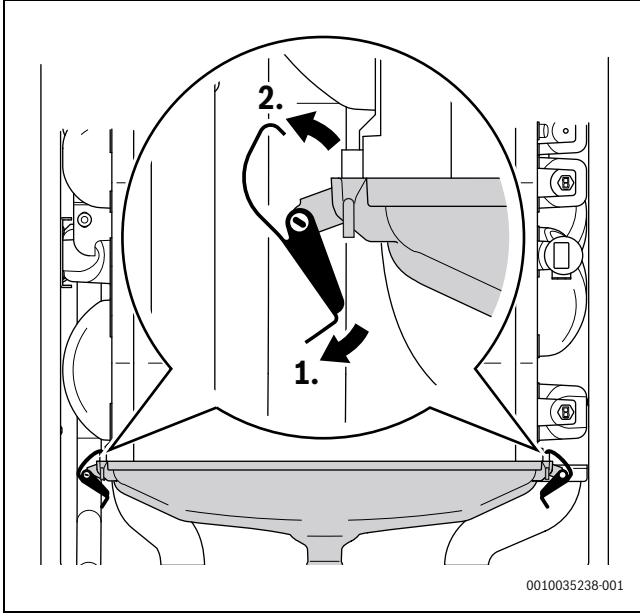
Res. 43 Yoğuşma suyu kabının hızlı kenetlemeli kilitlerinin açılması
