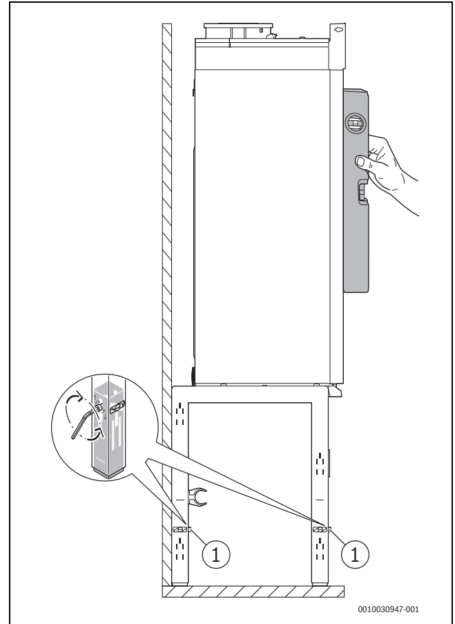
Res. 10 Isıtma kazanının yer kiti üzerinde hizalanması
