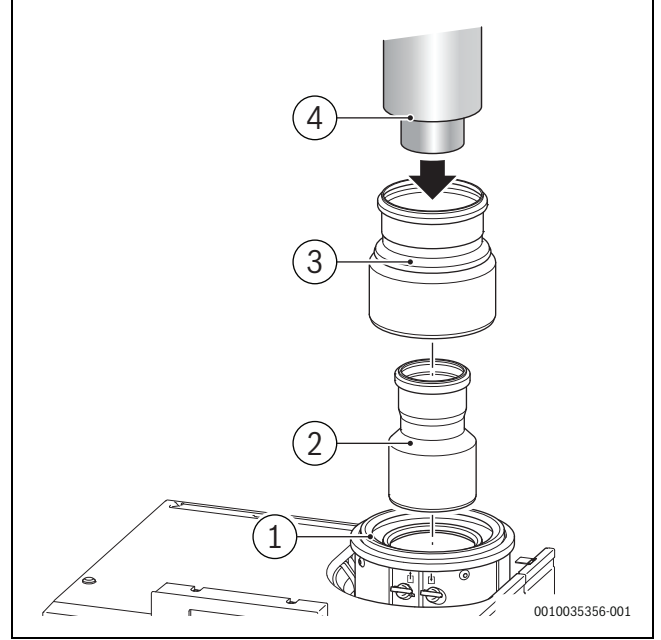
Res. 3 Atık gaz adaptörünün Ø 80/125 monte edilmesi
