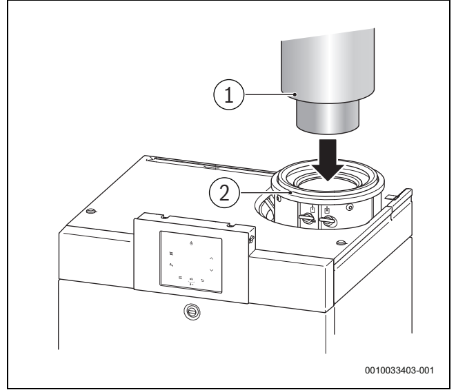
Res. 1 Konsantrik boru (oda havasından bağımsız)
