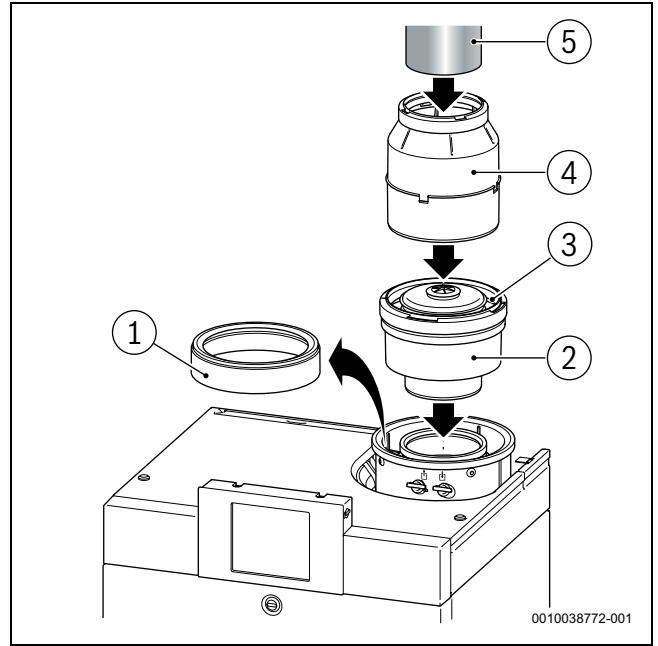
Res. 5 Harici atık gaz çekvalfini monte edilmesi
