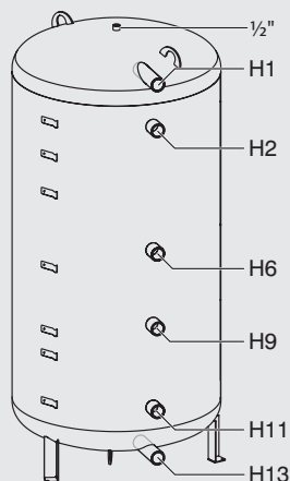
P 500, 750, 1000.6 (W)
