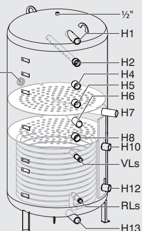
PNRZ 750, 1000.6 E(W)
