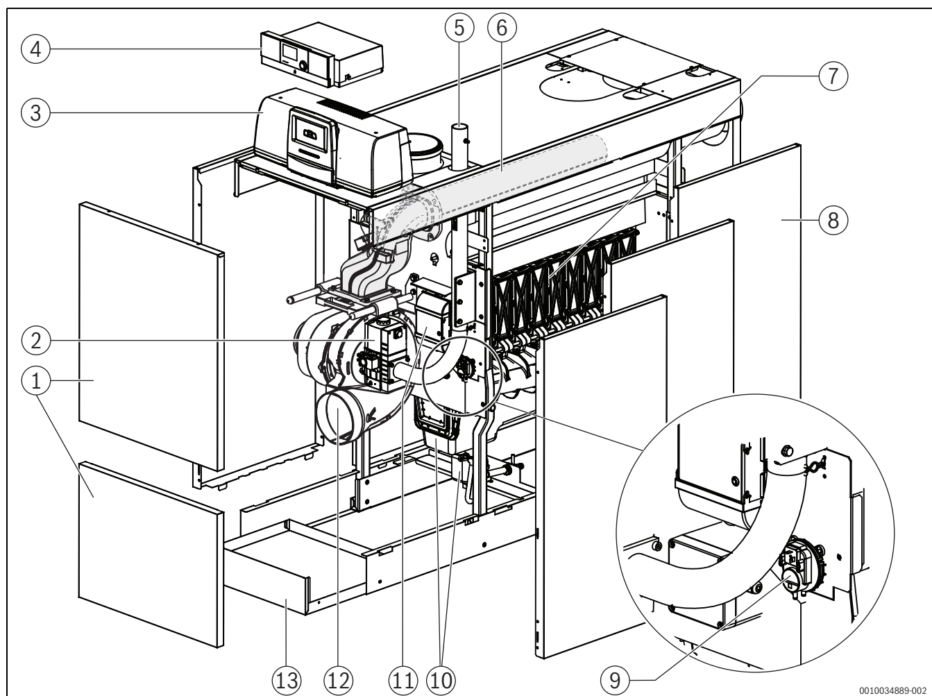
Fig. 1 Componenti principali Logano plus KB472, 350...620 kW (in figura: versione destra; il coperchio di pulizia e mandata e ritorno si trovano a destra)
