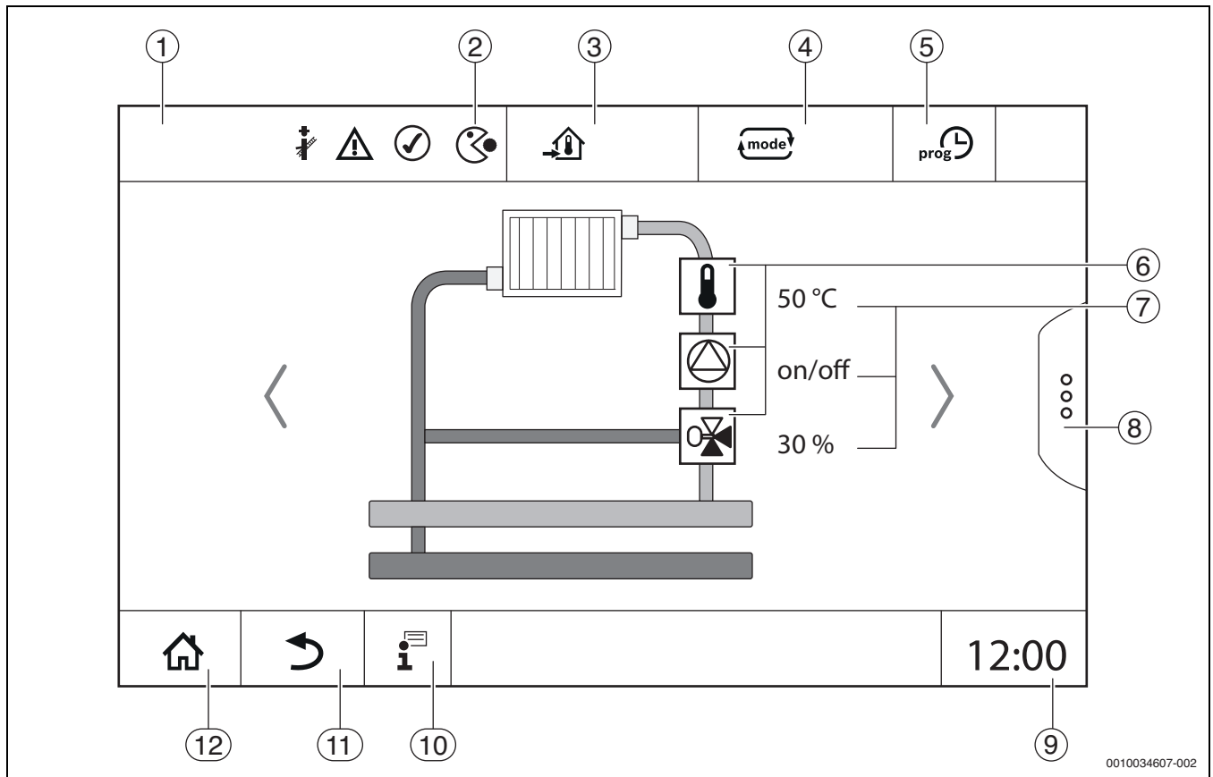
Fig. 13 Elementi di comando e visualizzazione (esempio)
