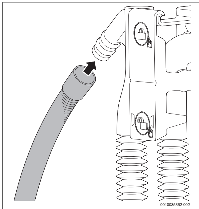
Fig. 36 Montarea furtunului pentru condensat la sifonul pentru condensat
