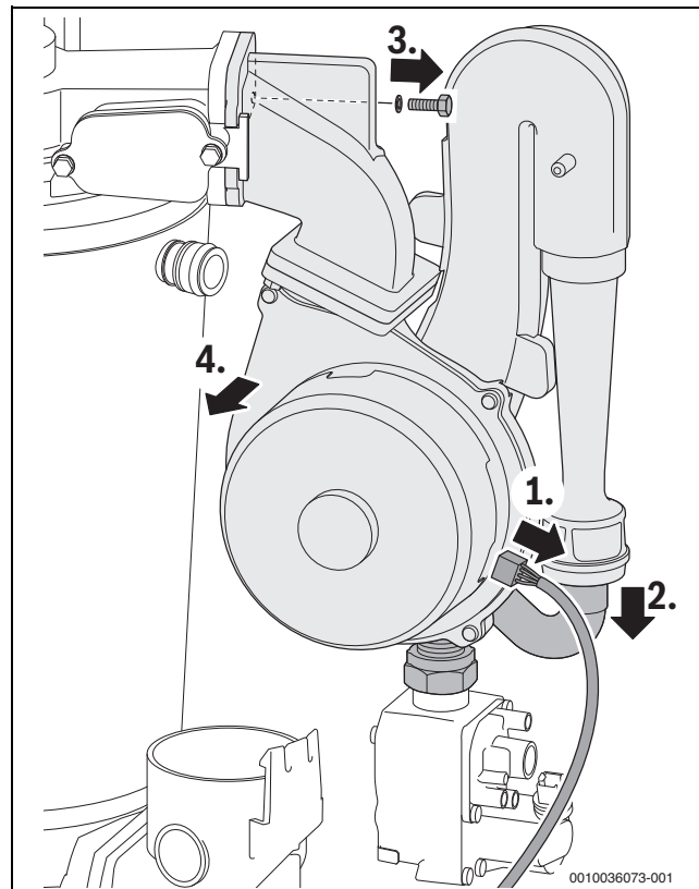
Fig. 57 Demontarea suflantei și a dispozitivului de amestecare
