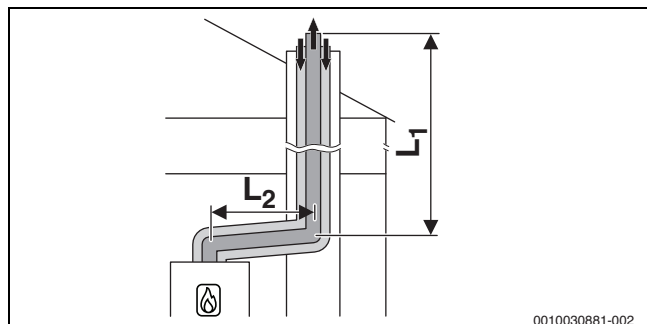
Fig. 10 Ghidarea concentrică a aerului/gazelor arse în puț conform C 33x
