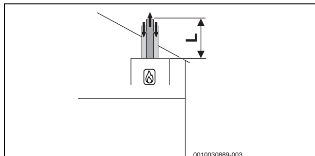
Fig. 11 Ghidarea verticală, concentrică a aerului/gazelor arse conform C 33x
