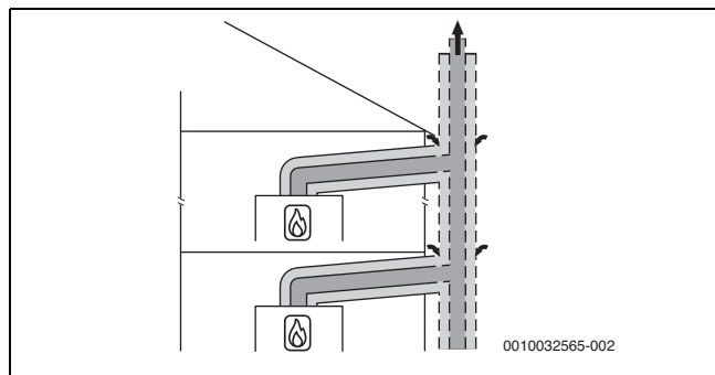
Fig. 23 Acoperire multiplă conform C_{(12)3x} cu ghidarea concentrică a aerului/gazelor arse în încăperea centralei termice
