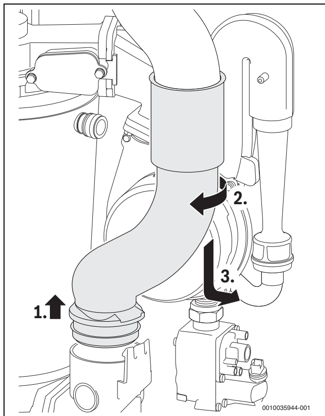
Fig. 56 Demontați tubulatura evacuare gaze arse
