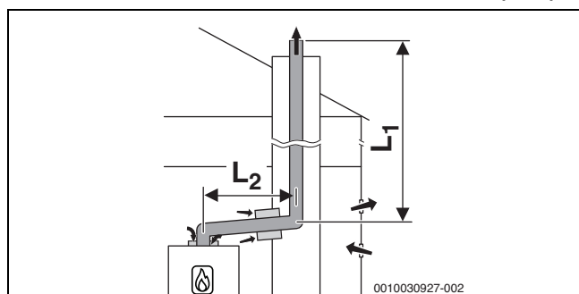
Fig. 19 Ghidarea rigidă a gazelor arse în puț conform B 23p /B 53p cu alimentare cu aer dependentă de aerul din încălă la nivelul aparatului și elementului de legătură concentric dintre încăperea centralei termice și puț
