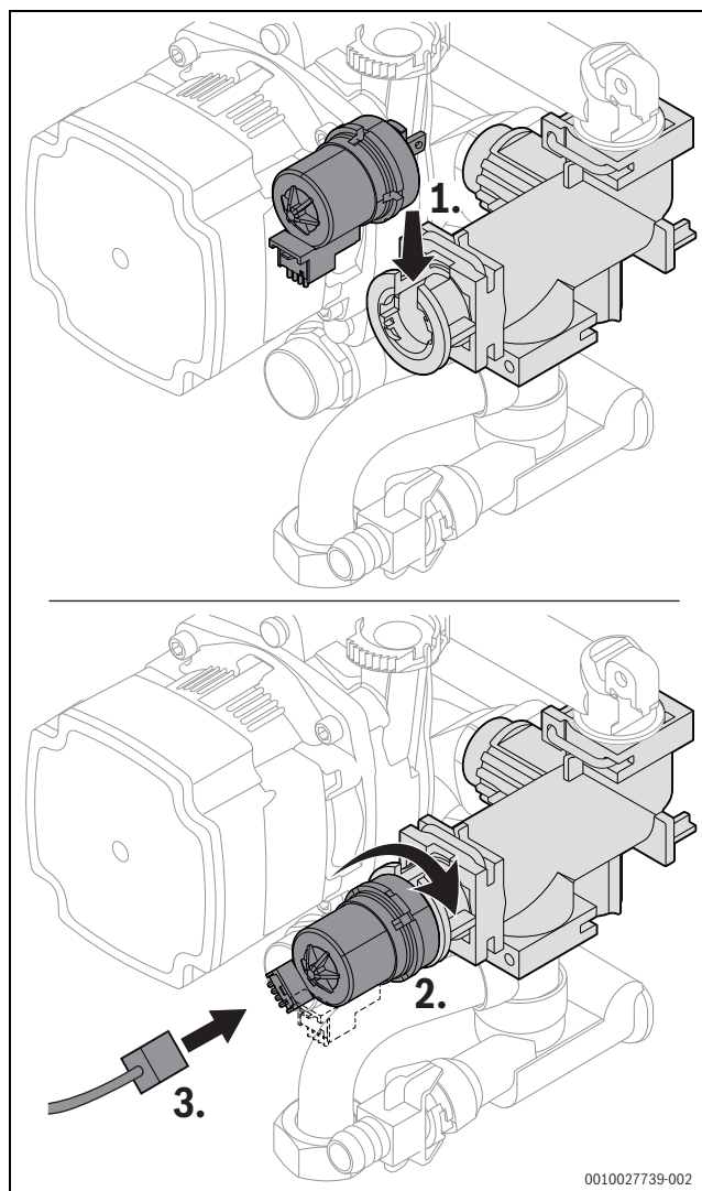
Fig. 85 Montați motorul vanei cu 3 căi (variante fără șuruburi)
