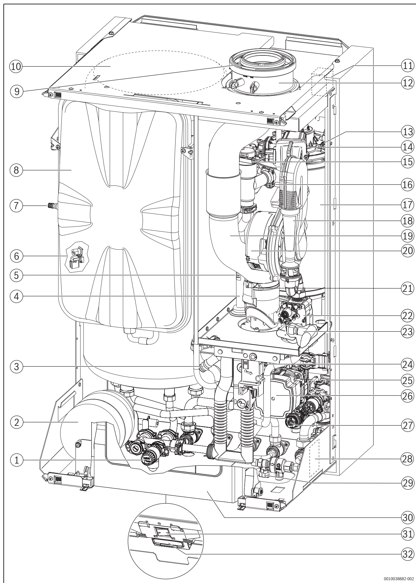
Fig. 5 Structura echipamentului
