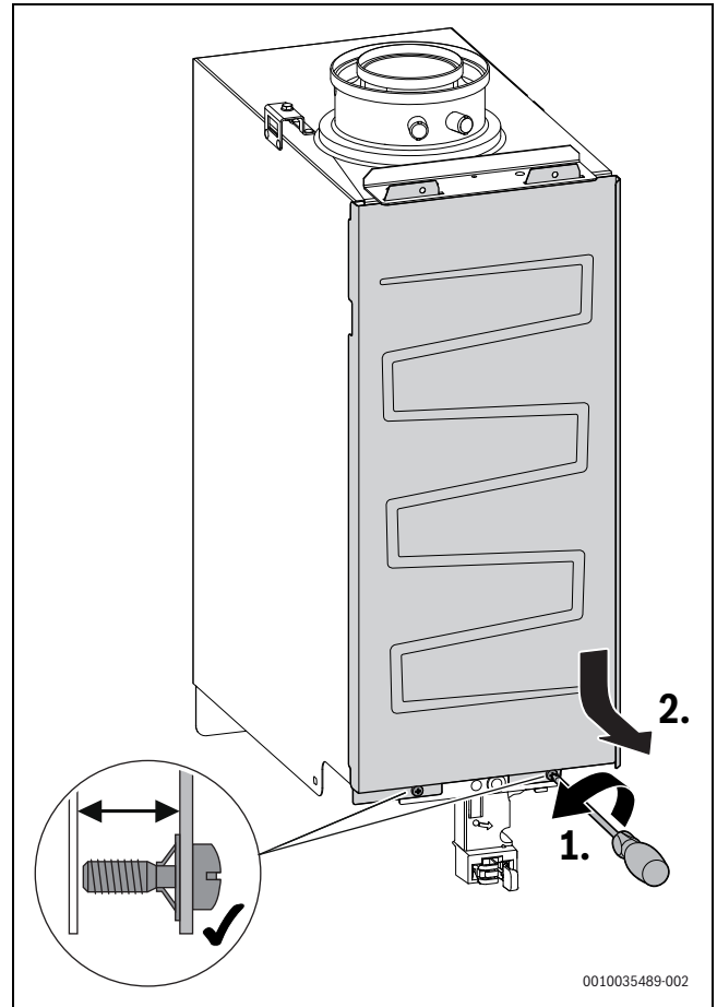
Fig. 49 Scoaterea ajutorului de arzător
