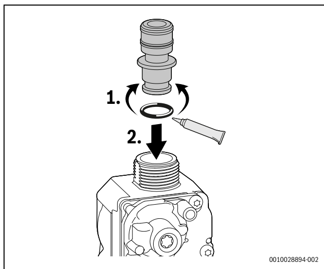
Fig. 82 Introducerea ajutorului de strângare pentru gaz
