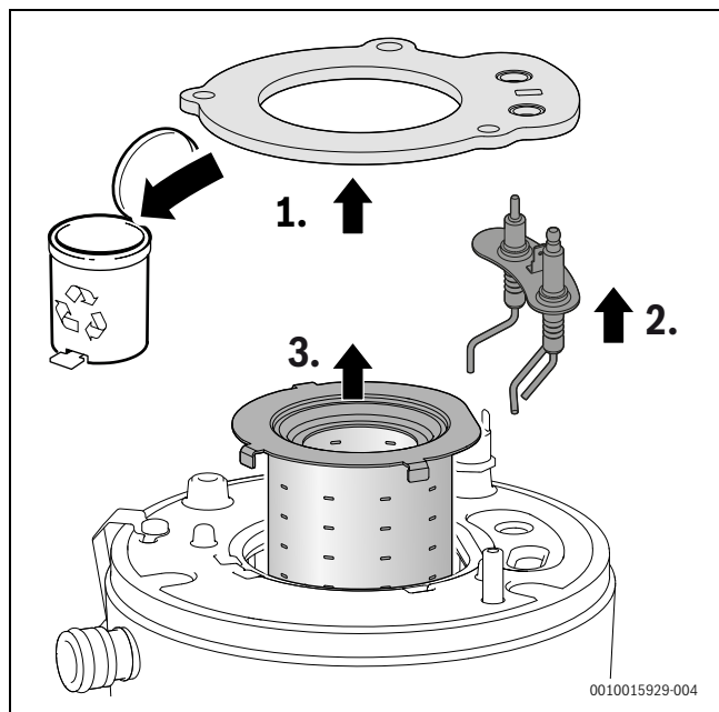
Fig. 60 Scoateți arzătorul
