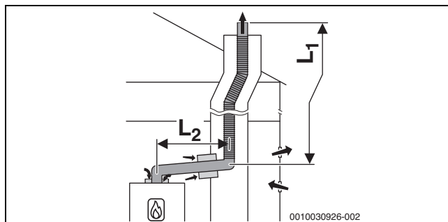
Fig. 20 Ghidarea flexibilă a gazelor arse în puț conform B 23p /B 53p cu alimentare cu aer dependentă de aerul din încălă la nivelul aparatului și elementului de legătură concentric dintre încăperea centralei termice și puț
