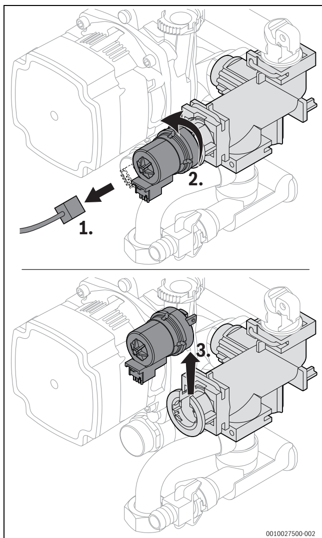
Fig. 84 Demontați motorul vanei cu 3 căi (variante fără șuruburi)
