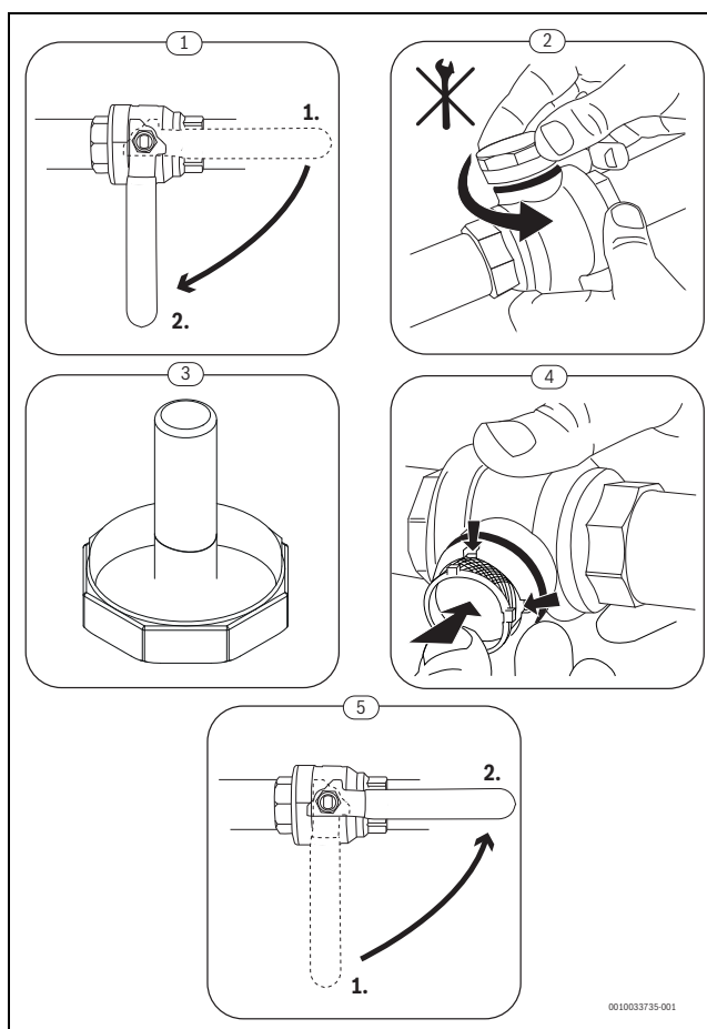
Afb. 5 Filterreiniging
