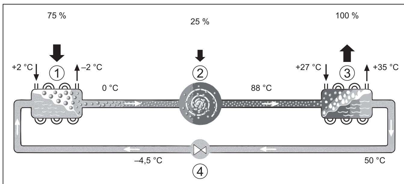
Afb. 1 Werkingsprincipe van het koelmiddelcircuit in de warmtepomp
