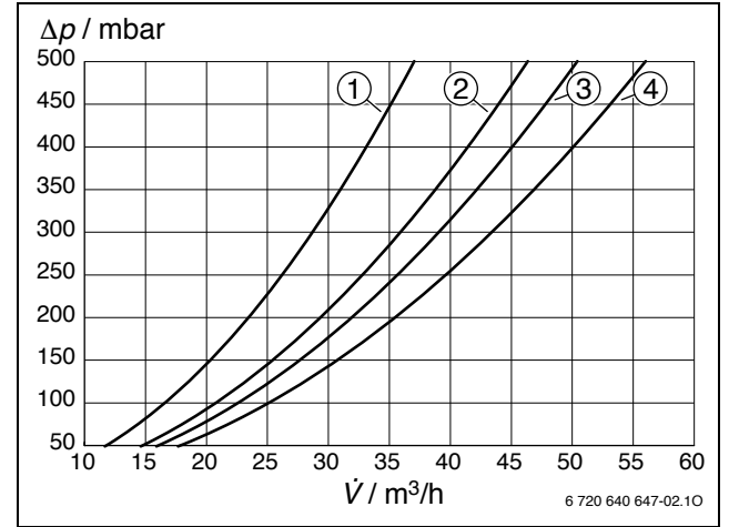
Su tarafında basınç kaybı Logano plus GB402
