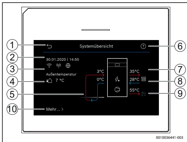
Bild 7 Systemübersicht
