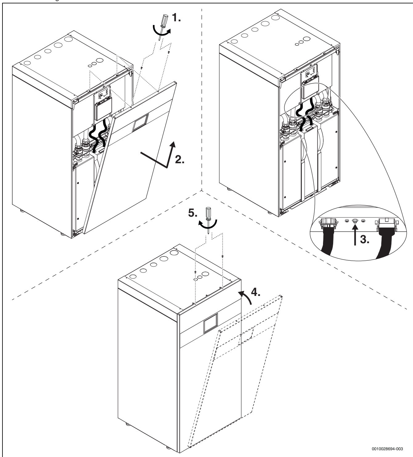
Bild 9 Zurücksetzen des Überhitzungsschutzes
