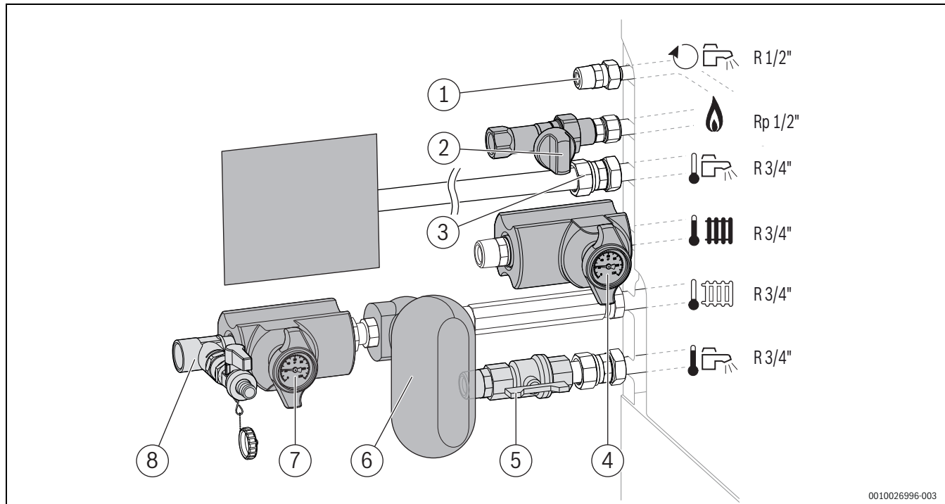
Rys. 4 Przykład: przyłącze po stronie gazu i wody z zestawem przyłączeniowym zaworów (osprzęt dodatkowy CS 28-1) po lewej stronie
