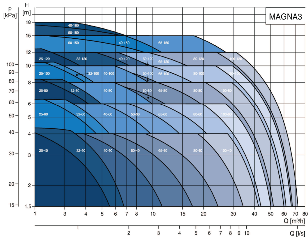
Abb. 3 Leistungsbereich der Einzelpumpen MAGNA3
