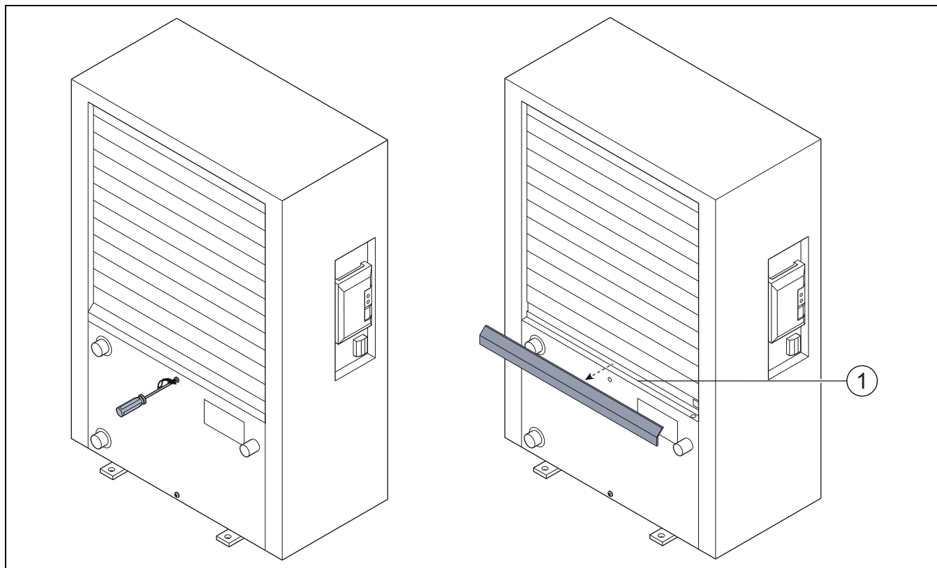
Obr. 9 Vana na kondenzát tepelného čerpadla
