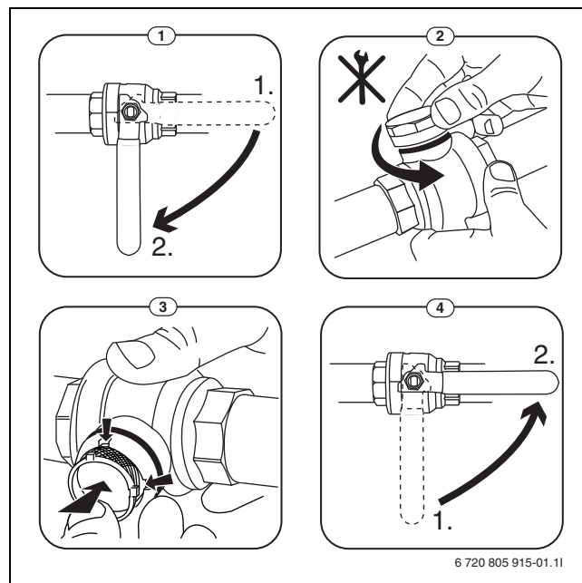
Rys. 7 Czyszczenie sitka
