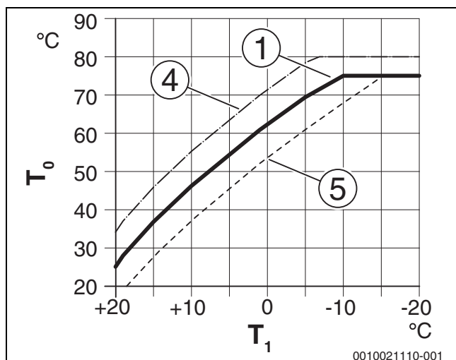
Obr. 5 Nastavení ekvitemní křivky pro otopná tělesa Paralelní posun podle Ofset teploty prostoru nebo požadované teploty prostoru
