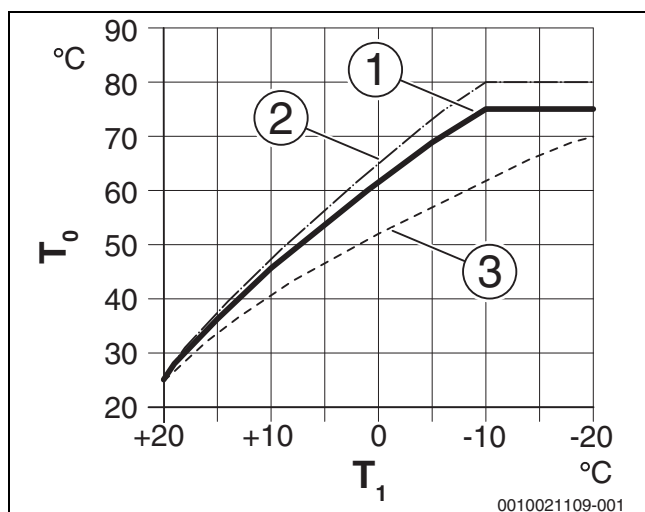
Obr. 4 Nastavení ekvitemní křivky pro otopná tělesa Sklon podle návrhové teploty T_0 a minimální venkovní teploty T_{1,min}
