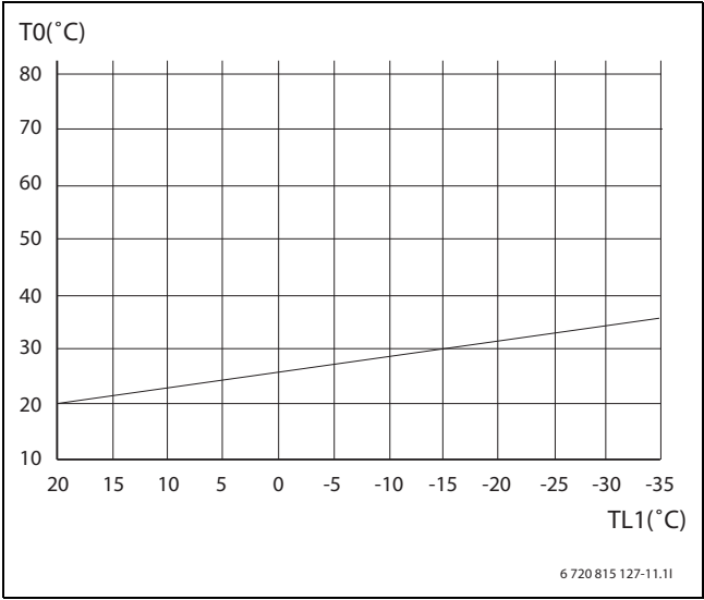
Rys. 3 Ogrzewanie podłogowe
