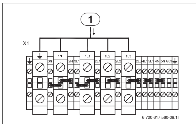
Rys. 43 Wersja standardowa, WPS 13-1 - 17-1
