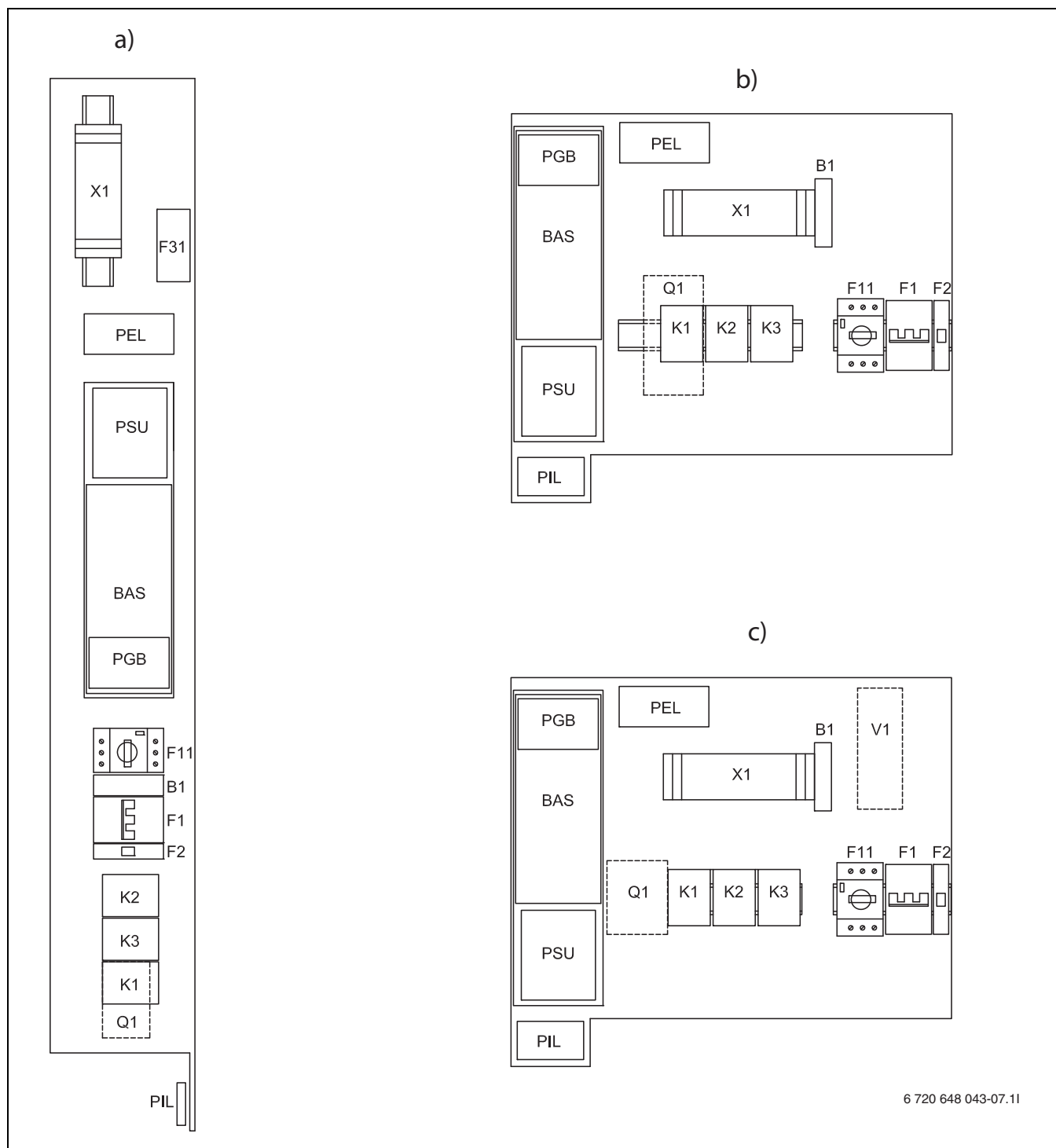
Rys. 34 Płyta główna – przegląd
