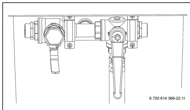
Rys. 26 Stacja napełniania w pozycji mieszania
