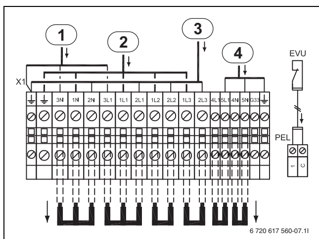
Rys. 42 Alternatywa C, WPS 6-1 - 10-1 i WPS 6K-1 - 10K-1
