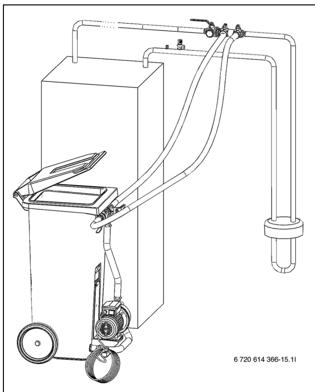
Rys. 24 Napełnianie przy użyciu stacji napełniania
