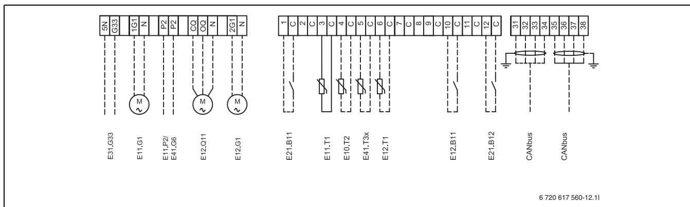
Rys. 47 Podłączenia zewnętrzne
