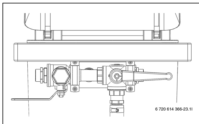
Rys. 27 Stacja napełniania w pozycji napełniania
