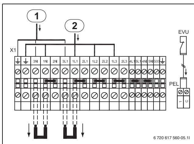
Rys. 40 Alternatywa A, WPS 6-1 - 10-1 i WPS 6K-1 - 10K-1
