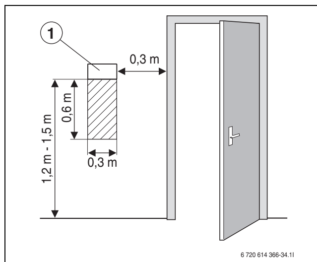
Rys. 21 Zalecane miejsce montażu czujnika pokojowego T5
