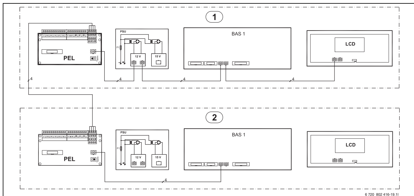
Rys. 74 Schemat magistrali CAN-BUS z dwiema pompami ciepła (6–17 kW)
