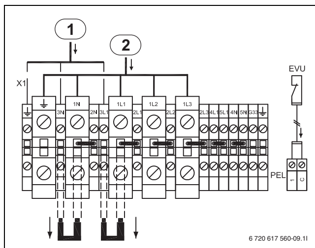
Rys. 44 Alternatywa A, WPS 13-1 - 17-1
