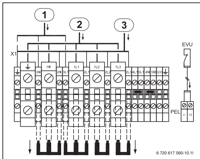
Rys. 45 Alternatywa B, WPS 13-1 - 17-1
