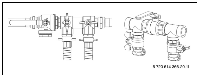
Rys. 28 Urządzenia napełniające w pozycji zwiększania ciśnienia
