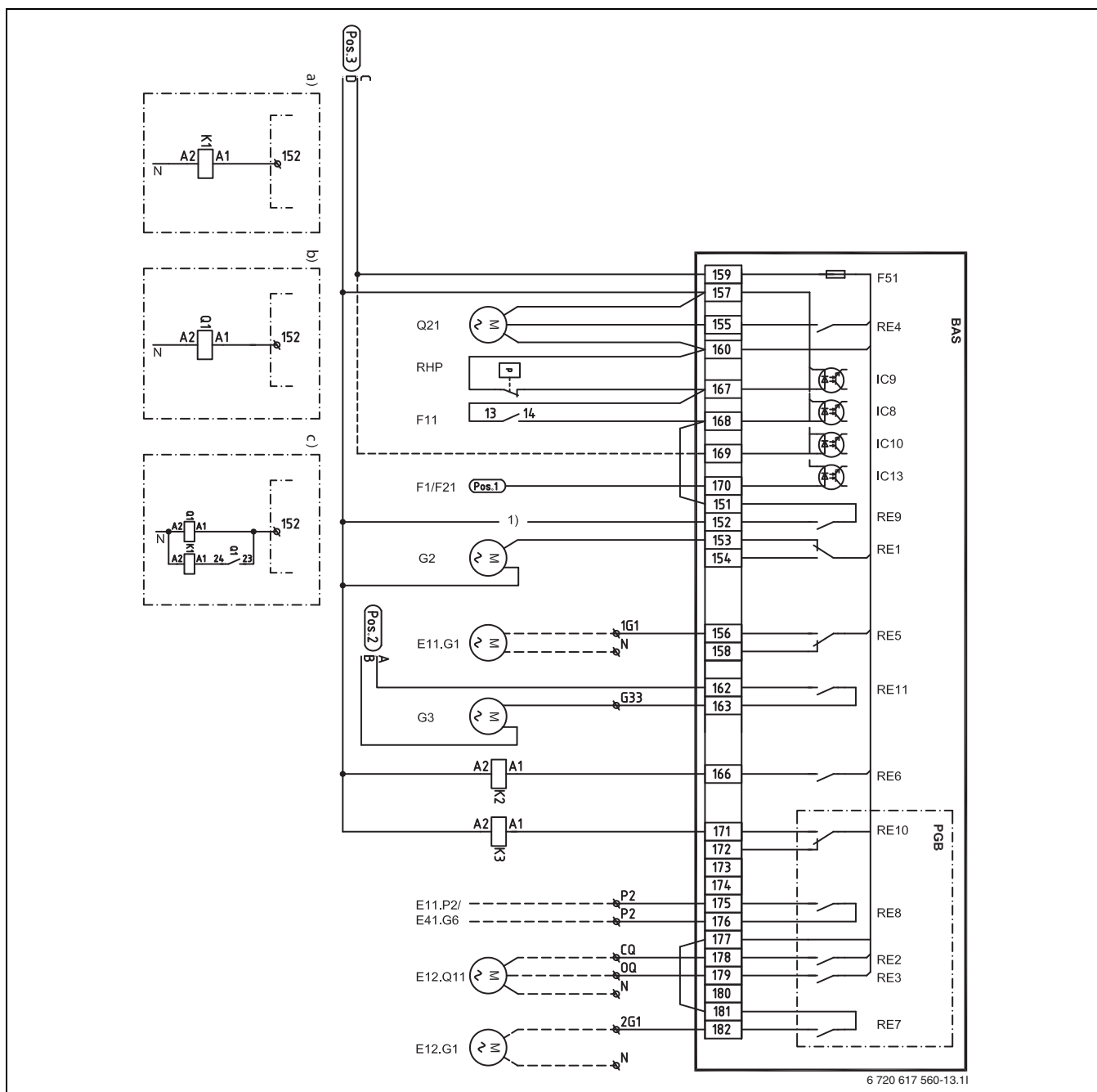
Rys. 50 Kompletny schemat przyłączeniowy (230 V)
