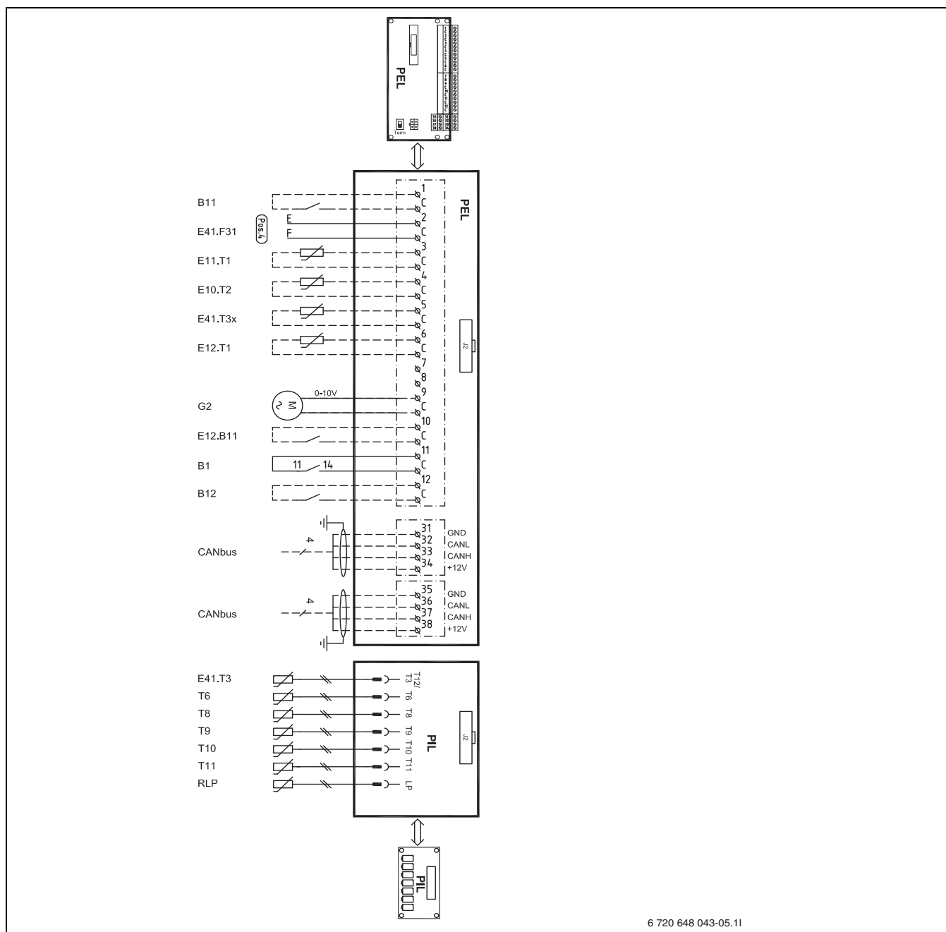
Rys. 51 Kompletny schemat przyłączeniowy (niskie napięcie)
