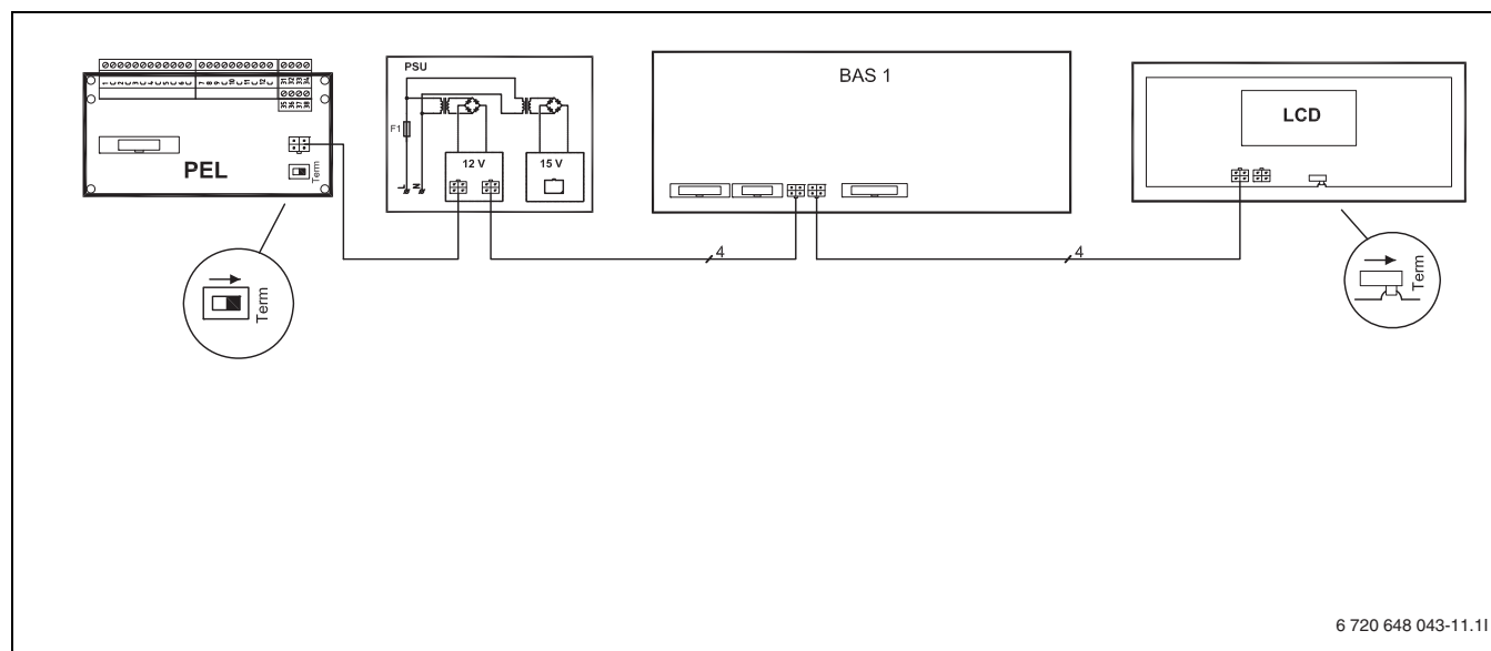
Rys. 35 CAN-BUS – przegląd
