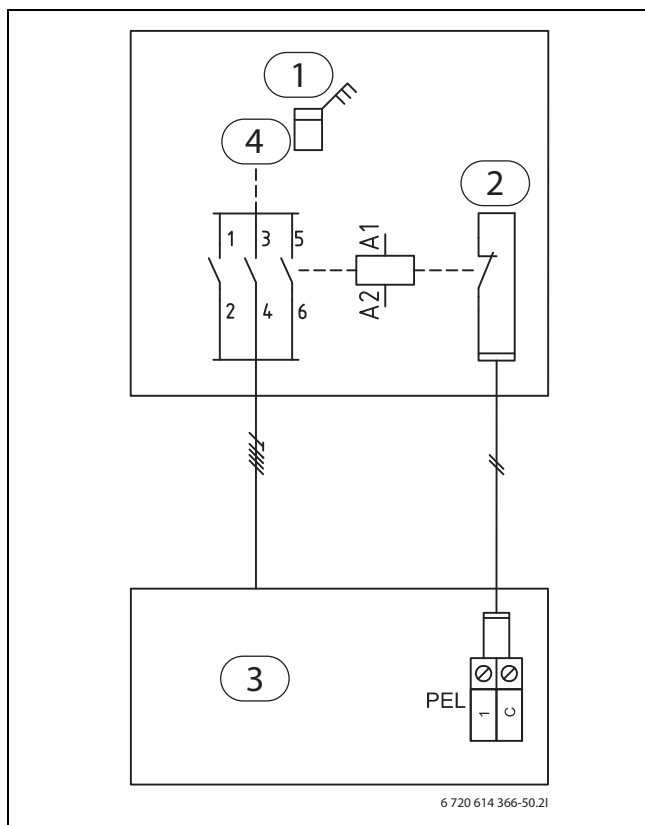
Rys. 37 Okres blokady aktywny
