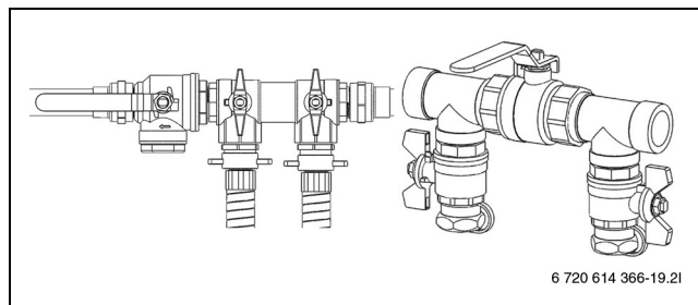
Rys. 25 Urządzenia napełniające w pozycji napełniania.
