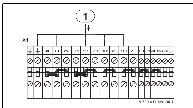
Rys. 39 Wersja standardowa, WPS 6-1 - 10-1 i WPS 6K-1 - 10K-1
