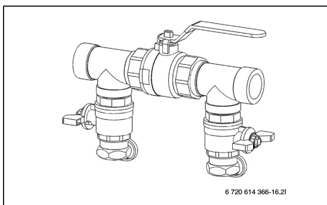
Rys. 23 Urządzenie napełniające WPS 13-1...17-1
