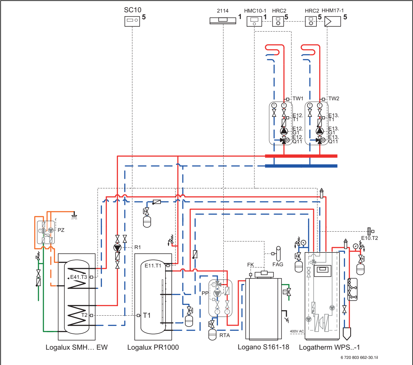
Rys. 15 Biwalentny obieg grzewczy bez mieszania z zasobnikiem buforowym i kotłem na paliwo stałe
