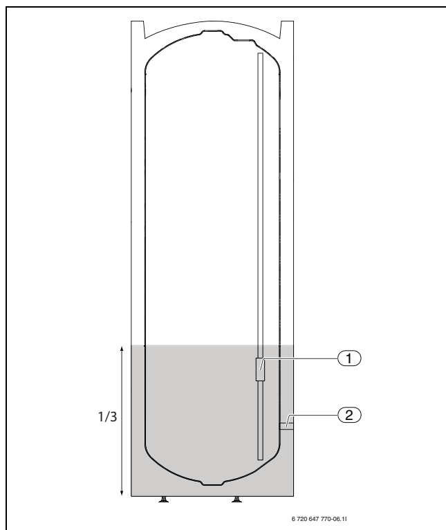
Rys. 20 Montaż czujników temperatury
