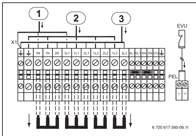
Rys. 41 Alternatywa B, WPS 6-1 - 10-1 i WPS 6K-1 - 10K-1
