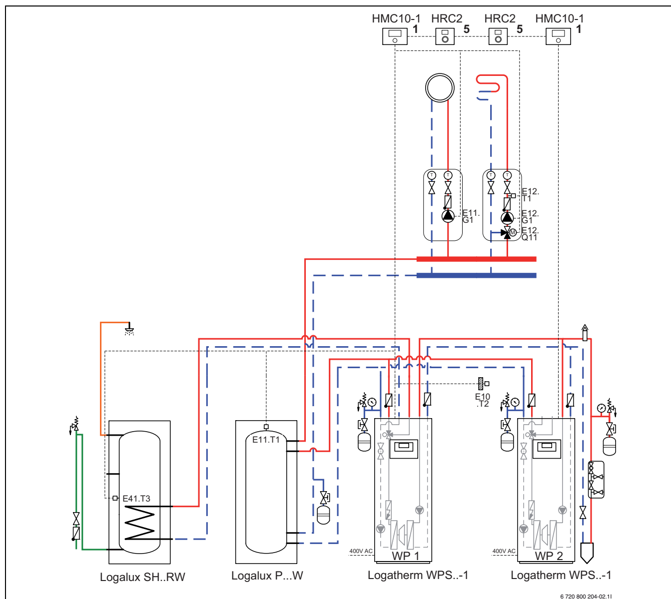
Rys. 73 Dwie pompy ciepła (połączone kaskadowo) z obiegiem grzewczym bez zaworu mieszającego i z zaworem mieszającym, ze zbiornikiem roboczym i zewnętrznym podgrzewaczem CWU.
