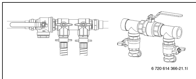
Rys. 29 Urządzenia napełniające w pozycji normalnej
