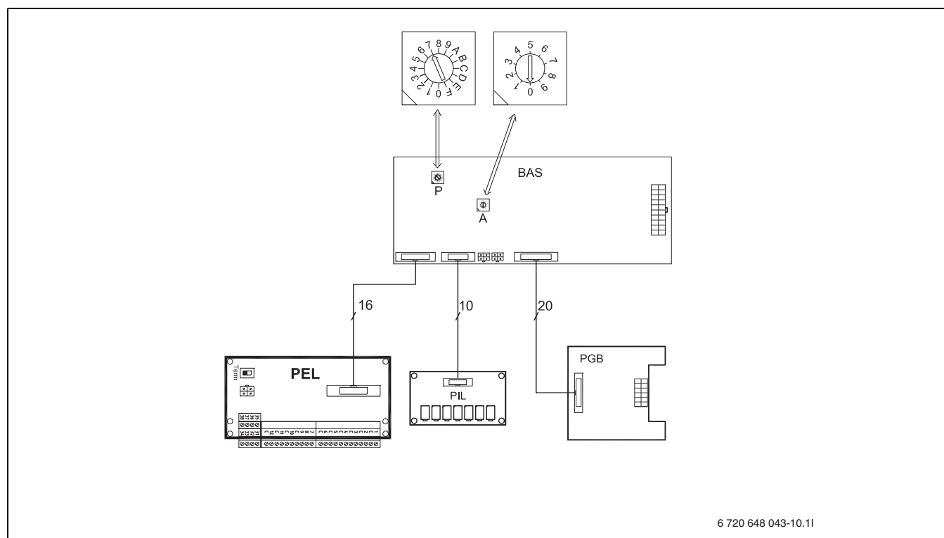
Rys. 36 Połączenia płyty głównej
