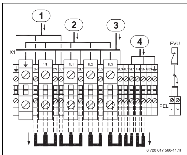
Rys. 46 Alternatywa C, WPS 13-1 - 17-1
