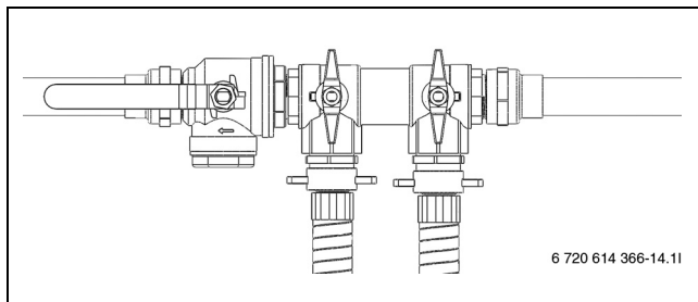
Rys. 22 Urządzenie napełniające WPS 6-1...10-1, WPS 6K-1...10 K-1
