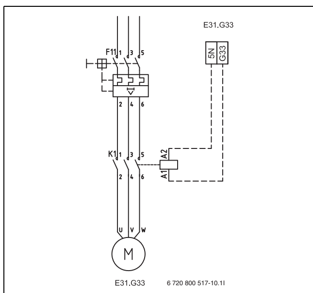
Rys. 48 Przyłącze pompy wody gruntowej
