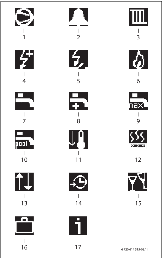
Obr. 18 Provozní symboly
