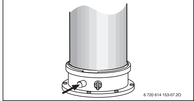
Res. 37 Atık gaz ölçüm ağızı
