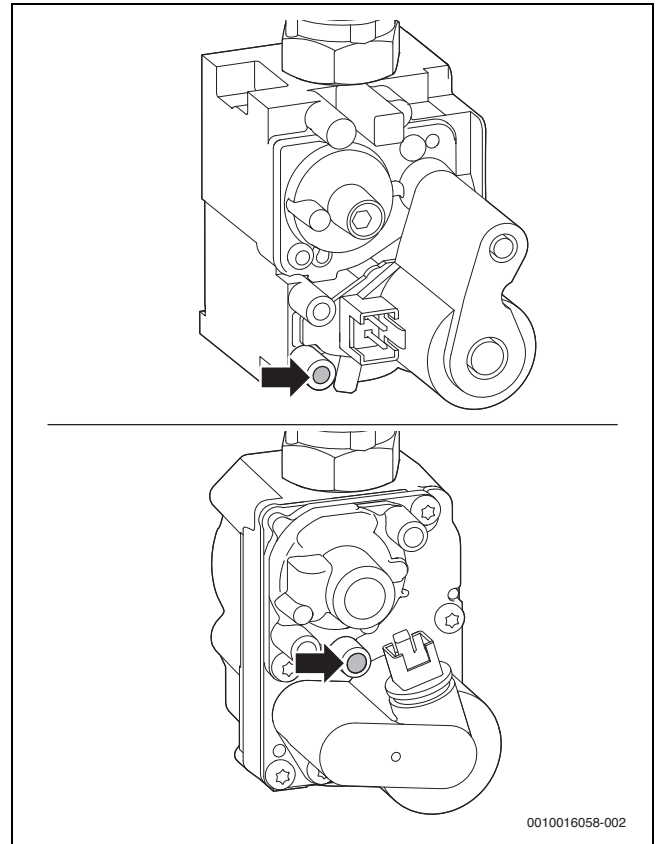
Res. 40 Gaz bağlantı basıncı için ölçüm ağızı
