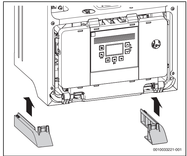
Res. 71 Yan plastik çıtaların takılması
