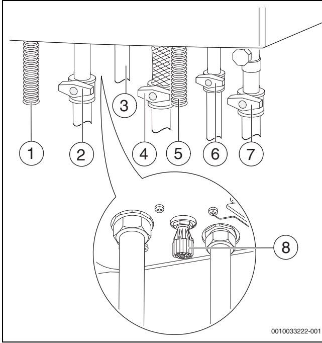
Res. 26 Gaz ve su tarafı bağlantıları (aksesuar)
