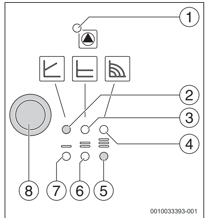
Рис. 86 Обзор
