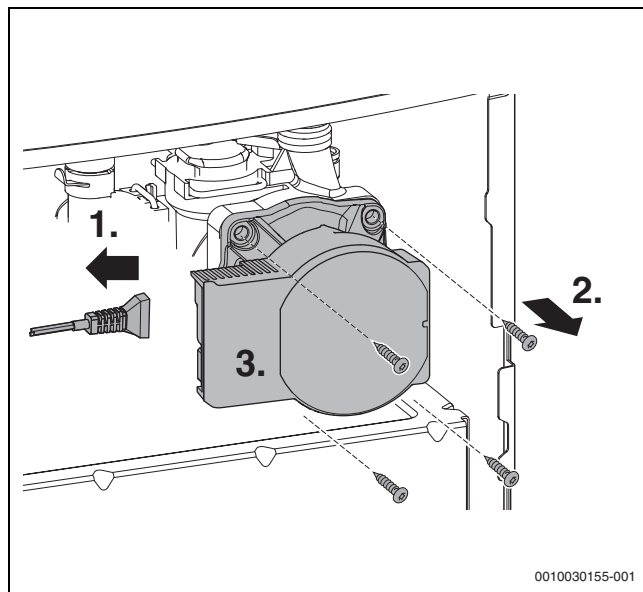
Рис. 111 Демонтаж насоса отопительного контура
