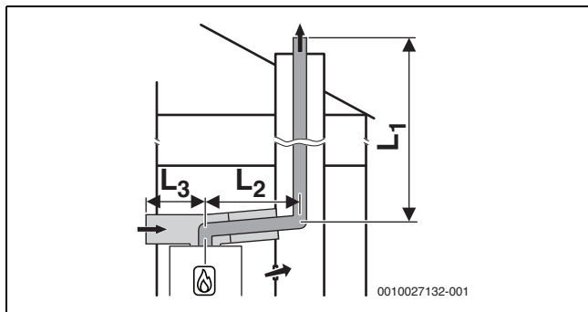
Рис. 19 Схема жесткого отвода дымовых газов согласно C_{53x} в шахте и схема подачи воздуха/отвода дымовых газов с отдельной линией подвода воздуха и концентрической линией отвода дымовых газов в помещении для установки
