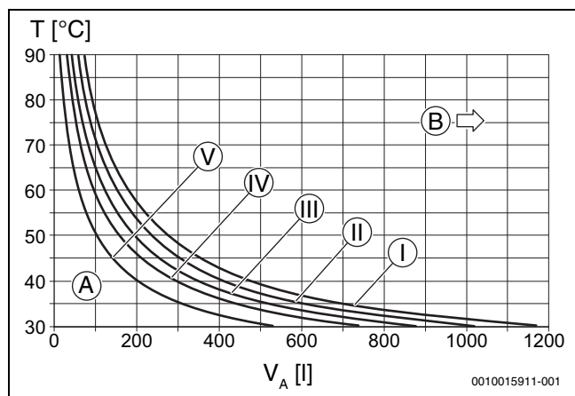
Рис. 82 Характеристики расширительного бака
