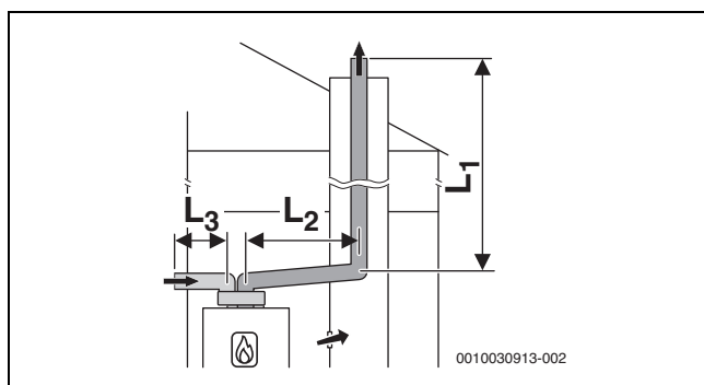
Рис. 16 Схема жесткого отвода дымовых газов согласно C_{53} в шахте и схема подачи воздуха/отвода дымовых газов с раздельными трубами для линии подвода воздуха и линии отвода дымовых газов в помещении для установки
