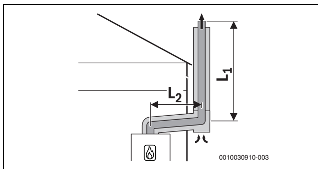
Рис. 56 Концентрическая схема подачи воздуха/отвода дымовых газов согласно C_{53x} по наружной стене
