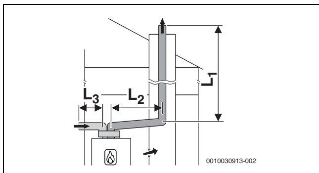
Рис. 20 Схема жесткого отвода дымовых газов согласно C_{53} в шахте и схема подачи воздуха/отвода дымовых газов с отдельными трубами для линии подвода воздуха и линии отвода дымовых газов в помещении для установки
