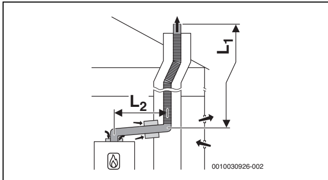
Рис. 69 Схема гибкого отвода дымовых газов в шахте согласно В 23р /В 53р с забором воздуха из помещения топочной для подвода воздуха и с концентрическим соединительным участком между помещением для установки и шахтой
