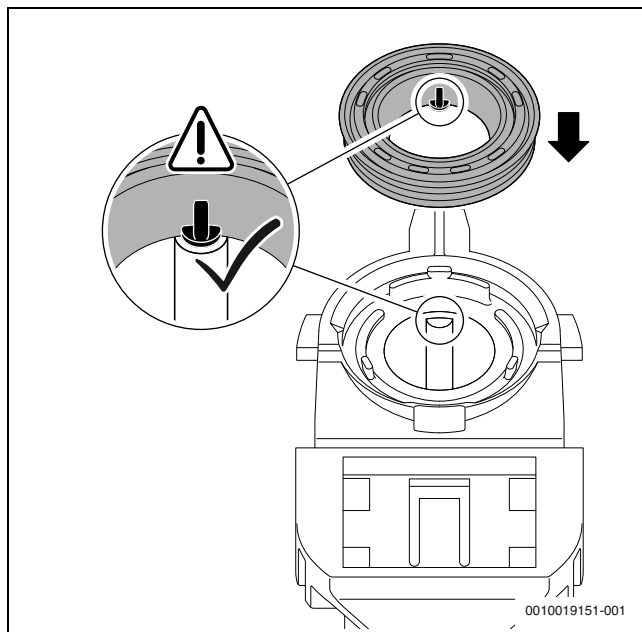
Рис. 103 Выравнивание нового уплотнения на сифоне для отвода конденсата
