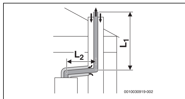
Рис. 62 Схема жесткого отвода дымовых газов согласно C_{93x} в шахте и концентрический подвод воздуха/отвод дымовых газов в помещении для установки
