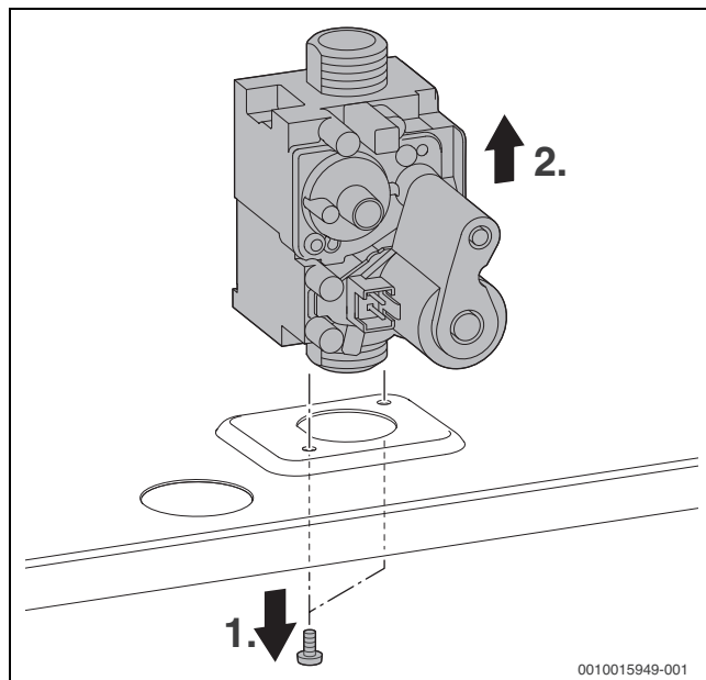
Рис. 110 Демонтаж газовой арматуры
