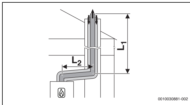
Рис. 49 Концентрическая схема подачи воздуха/отвода дымовых газов согласно C 33x в шахте
