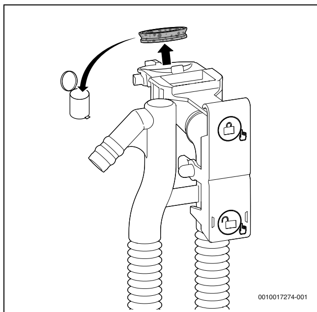
Рис. 102 Замена уплотнения сверху на сифоне для отвода конденсата
