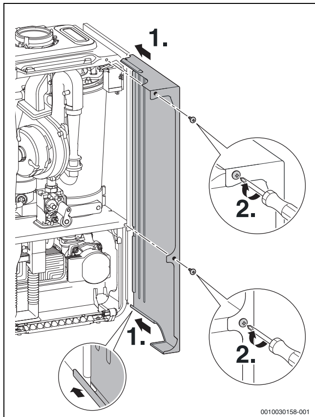
Рис. 116 Повторная установка боковой облицовки
