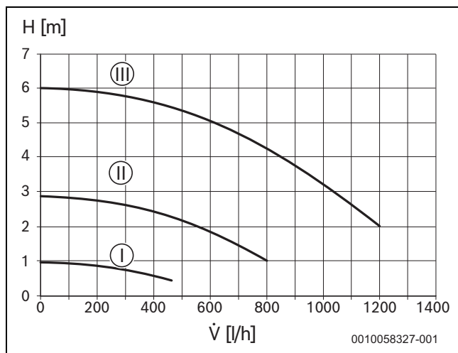
Рис. 88 Характеристическая кривая насоса отопительного контура (постоянное давление)
