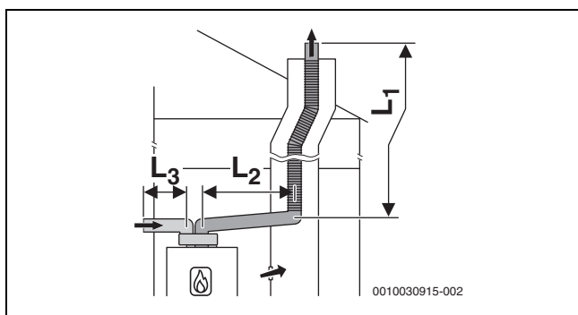
Рис. 55 Схема гибкого отвода дымовых газов согласно C_{53} в шахте и схема подачи воздуха/отвода дымовых газов с отдельными трубами для линии подвода воздуха и линии отвода дымовых газов в помещении для установки
