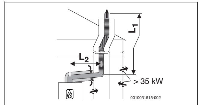
Рис. 71 Схема гибкого отвода дымовых газов в шахте согласно В 33 с забором воздуха из помещения через концентрический подвод воздуха/отвод дымовых газов в помещении для установки
