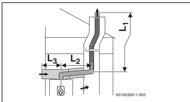
Рис. 21 Схема гибкого отвода дымовых газов согласно C_{53x} в шахте и схема подачи воздуха/отвода дымовых газов с отдельной линией подвода воздуха и концентрической линией отвода дымовых газов в помещении для установки
