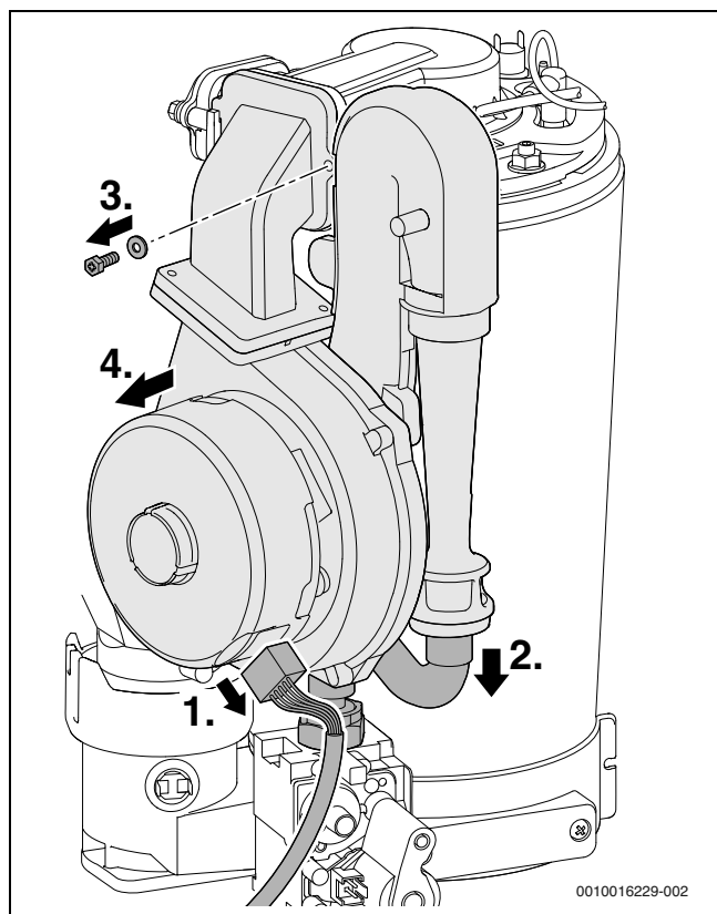
Рис. 91 Демонтаж вентилятор со смесительным устройством
