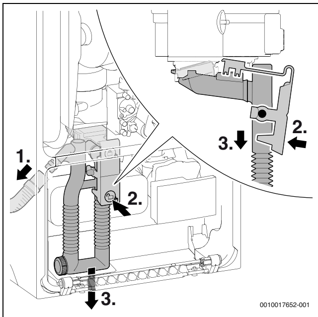
Рис. 100 Демонтаж конденсатного сифона
