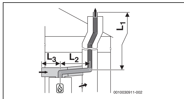
Рис. 53 Схема гибкого отвода дымовых газов согласно C 53x в шахте и схема подачи воздуха/отвода дымовых газов с отдельной линией подвода воздуха и концентрической линией отвода дымовых газов в помещении для установки
