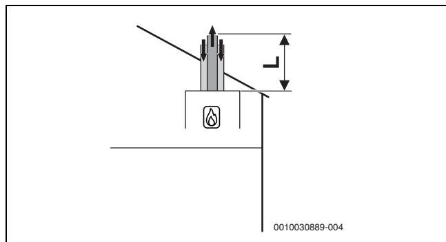
Рис. 48 Вертикальная концентрическая схема подачи воздуха/отвода дымовых газов согласно C 33x
