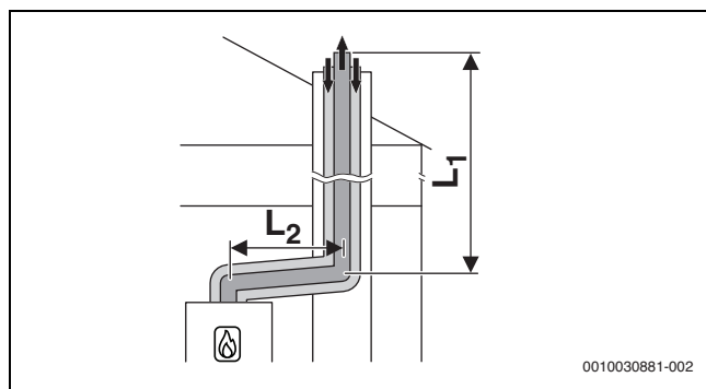
Рис. 9 Концентрическая схема подачи воздуха/отвода дымовых газов согласно C_{33x} в шахте
