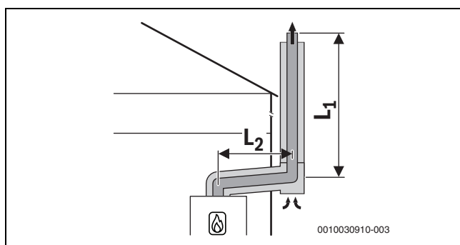
Рис. 61 Концентрическая схема подачи воздуха/отвода дымовых газов согласно C_{53x} по наружной стене
