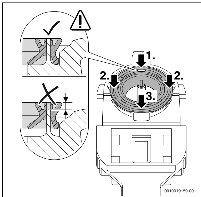
Рис. 104 Прижатие уплотнения
