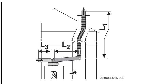
Рис. 22 Схема гибкого отвода дымовых газов согласно C_{53} в шахте и схема подачи воздуха/отвода дымовых газов отдельными трубами для линии подвода воздуха и линии отвода дымовых газов в помещении для установки
