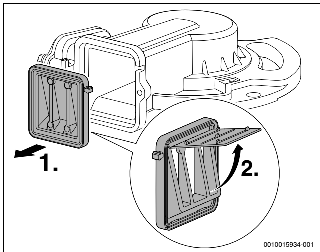
Рис. 93 Обратный клапан в смесительном устройстве
