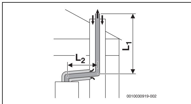
Рис. 24 Схема жесткого отвода дымовых газов согласно C_{93x} в шахте и концентрический подвод воздуха/отвод дымовых газов в помещении для установки
