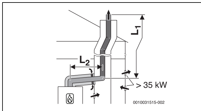
Рис. 33 Схема гибкого отвода дымовых газов в шахте согласно В 33 с забором воздуха из помещения через концентрический подвод воздуха/отвод дымовых газов в помещении для установки
