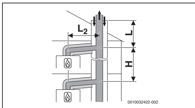
Рис. 37 Подключение нескольких котлов к одному дымоходу согласно C_{(14)3x} с коллективным жестким подводом воздуха/отводом дымовых газов в помещении для установки
