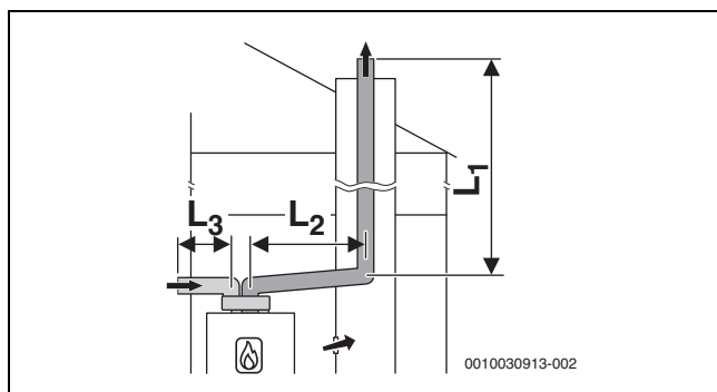
Рис. 58 Схема жесткого отвода дымовых газов согласно C_{53} в шахте и схема подачи воздуха/отвода дымовых газов с отдельными трубами для линии подвода воздуха и линии отвода дымовых газов в помещении для установки
