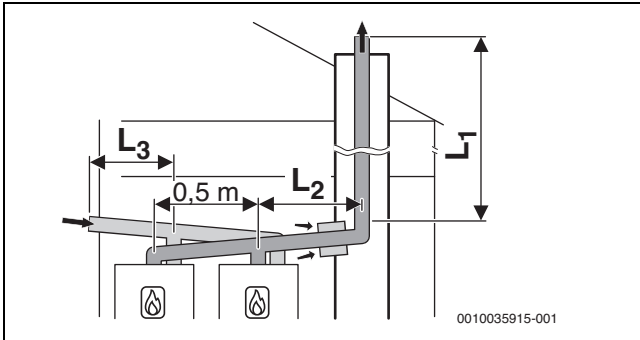
Рис. 78 Схема каскада с 2 котлами Схема жесткого отвода дымовых газов согласно C_{53} в шахте и схема подачи воздуха/отвода дымовых газов с отдельными трубами для линии подвода воздуха и линии отвода дымовых газов в помещении для установки
