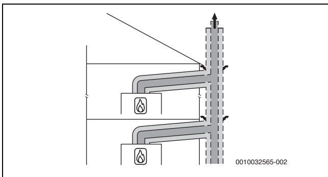
Рис. 73 Подключение нескольких котлов к одному дымоходу согласно C_{(12)3x} с концентрическим подводом воздуха/отводом дымовых газов вне помещения для установки
