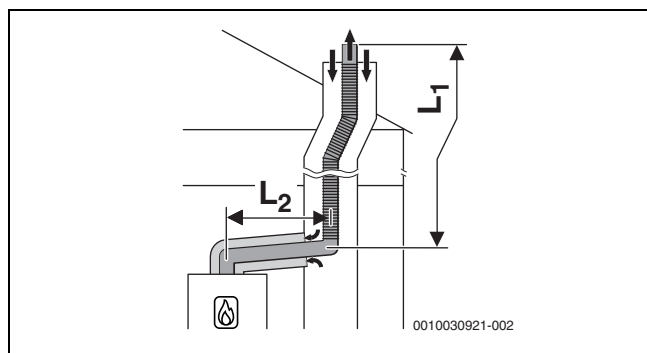
Рис. 63 Схема гибкого отвода дымовых газов согласно C 93x в шахте и концентрический подвод воздуха/отвод дымовых газов в помещении для установки
