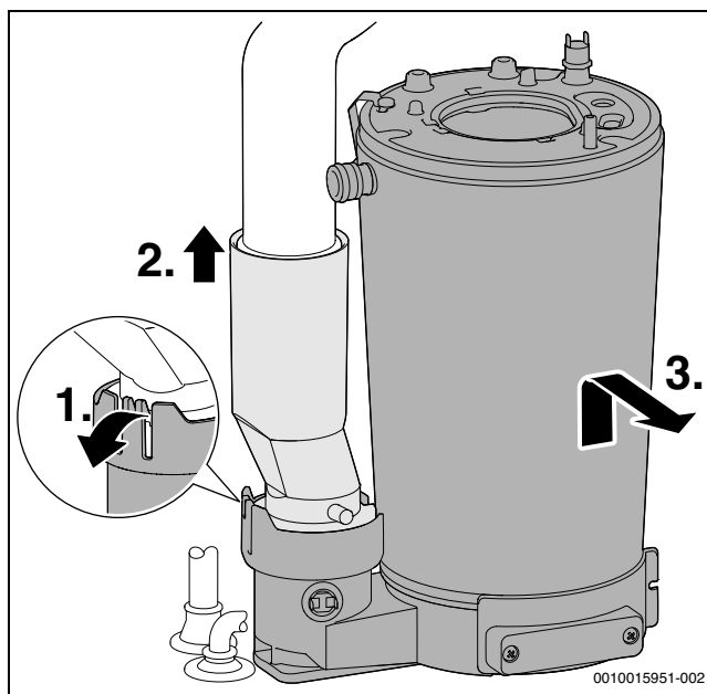
Рис. 115 Демонтаж теплообменника
