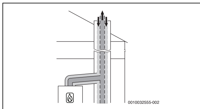
Рис. 51 Концентрическая схема подачи воздуха/отвода дымовых газов согласно C 43x в помещении для установки
