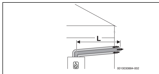
Рис. 46 Горизонтальная концентрическая схема подачи воздуха/отвода дымовых газов согласно C 13x через наружную стену
