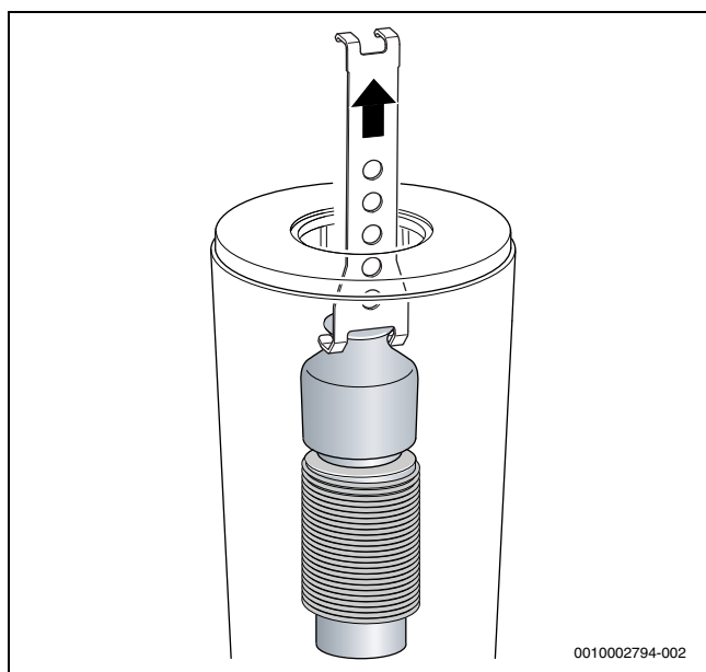
Рис. 95 Выньте верхний рассекатель
