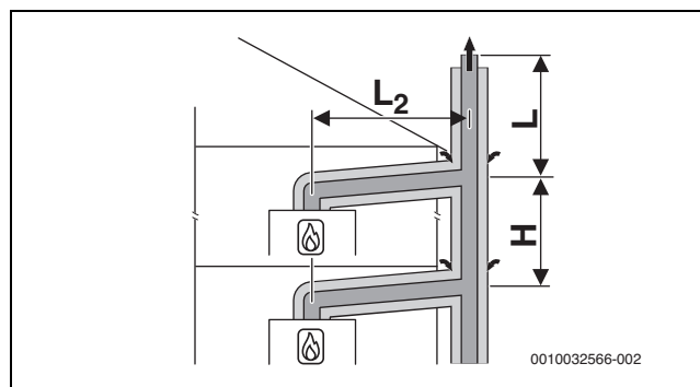
Рис. 36 Подключение нескольких котлов к одному дымоходу согласно C_{(13)3x} с концентрическим подводом воздуха/отводом дымовых газов по наружной стене и в помещении для установки
