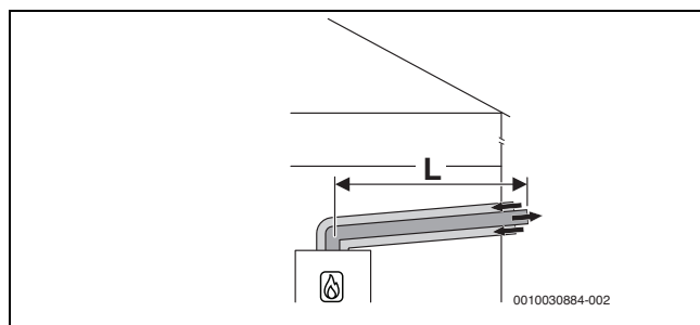
Рис. 44 Горизонтальная концентрическая схема подачи воздуха/отвода дымовых газов согласно C 13x через наружную стену
