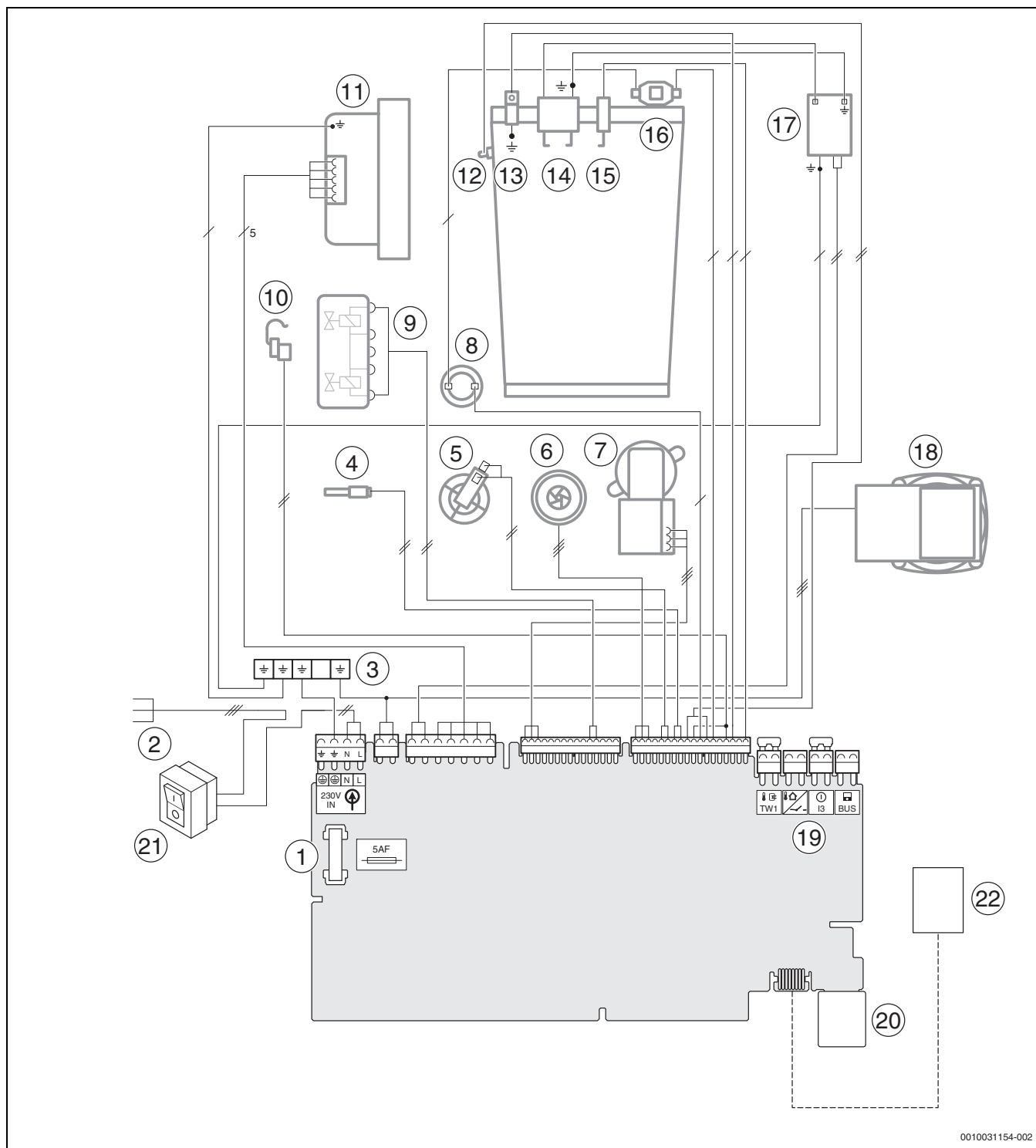
Рис. 119 Электрические соединения
