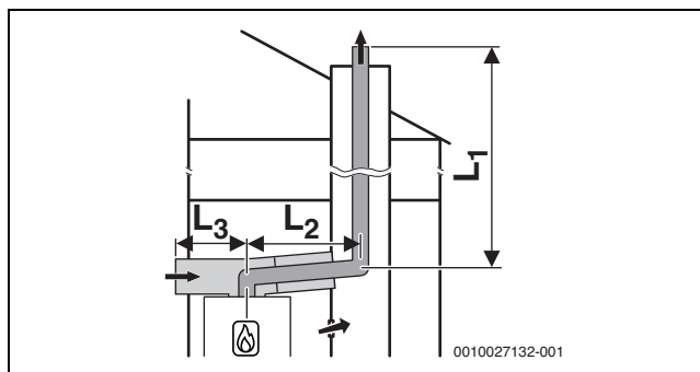
Рис. 14 Схема жесткого отвода дымовых газов согласно C_{53x} в шахте и схема подачи воздуха/отвода дымовых газов с отдельной линией подвода воздуха и концентрической линией отвода дымовых газов в помещении для установки
