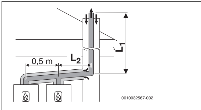
Рис. 41 Схема каскада с 2 котлами: Схема жесткого отвода дымовых газов согласно C 93x в шахте и концентрический подвод воздуха/отвод дымовых газов в помещении для установки
