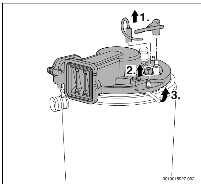
Рис. 92 Снятие крышки горелки
