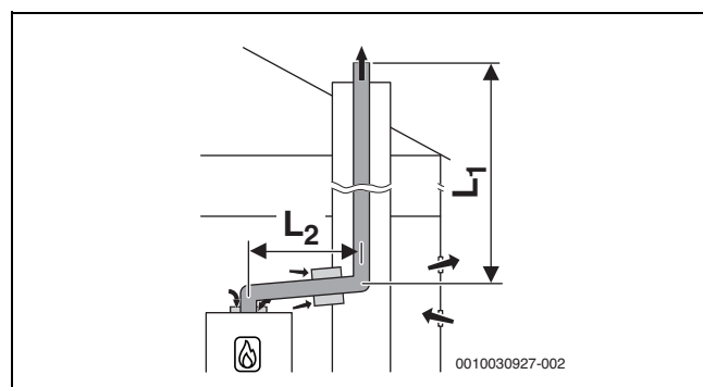
Рис. 68 Жёсткий отвод дымовых газов в шахте по B_{23p}/B_{53p} с забором воздуха из помещения и с концентрическим соединительным элементом между помещением установки котла и шахтой
