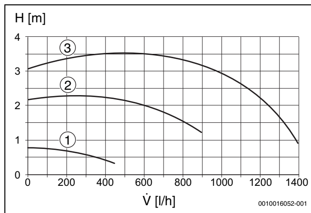
Рис. 89 Характеристическая кривая насоса отопительного контура (пропорциональное давление)
