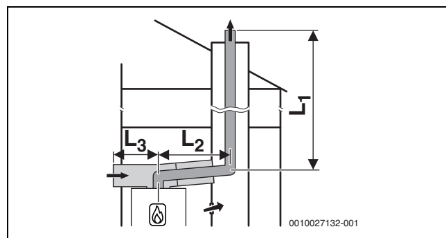
Рис. 52 Схема жесткого отвода дымовых газов согласно C 53x в шахте и схема подачи воздуха/отвода дымовых газов с отдельной линией подвода воздуха и концентрической линией отвода дымовых газов в помещении для установки
