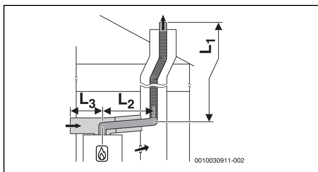
Рис. 59 Схема гибкого отвода дымовых газов согласно C_{53x} в шахте и схема подачи воздуха/отвода дымовых газов с отдельной линией подвода воздуха и концентрической линией отвода дымовых газов в помещении для установки
