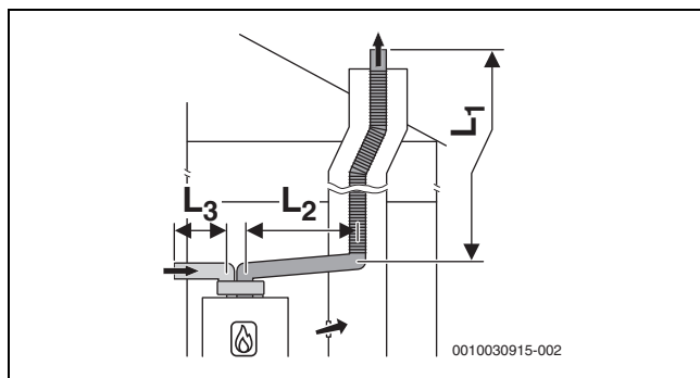
Рис. 17 Схема гибкого отвода дымовых газов согласно C_{53} в шахте и схема подачи воздуха/отвода дымовых газов раздельными трубами для линии подвода воздуха и линии отвода дымовых газов в помещении для установки
