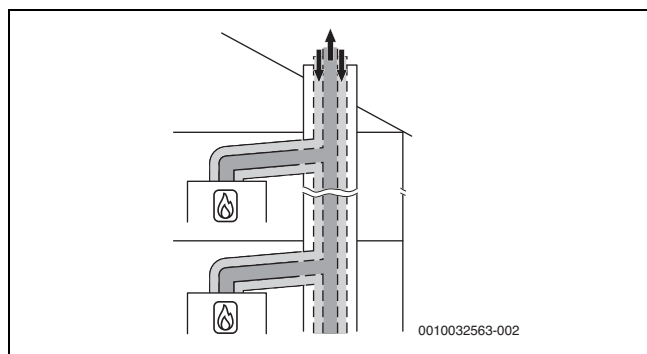
Рис. 72 Подключение нескольких котлов к одному дымоходу согласно C_{(10)3x} с концентрическим подводом воздуха/отводом дымовых газов вне помещения для установки
