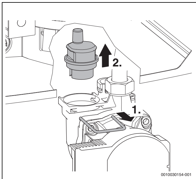
Рис. 112 Демонтаж автоматического воздухоотводчика
