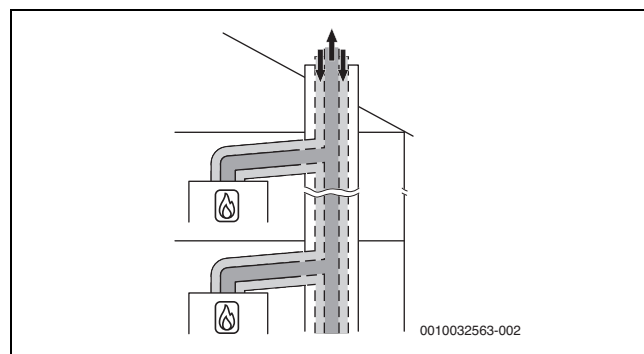
Рис. 34 Подключение нескольких котлов к одному дымоходу согласно C (10)3x с концентрическим подводом воздуха/отводом дымовых газов вне помещения для установки
