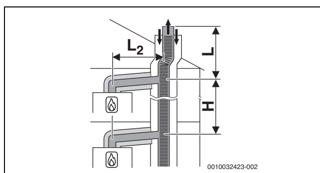
Рис. 76 Подключение нескольких котлов к одной дымовой трубе по C_{(14)3x} с коллективным гибким отводом дымовых газов и концентрическим подводом воздуха/отводом дымовых газов в помещении установки оборудования
