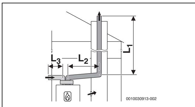
Рис. 54 Схема жесткого отвода дымовых газов согласно C_{53} в шахте и схема подачи воздуха/отвода дымовых газов с отдельными трубами для линии подвода воздуха и линии отвода дымовых газов в помещении для установки
