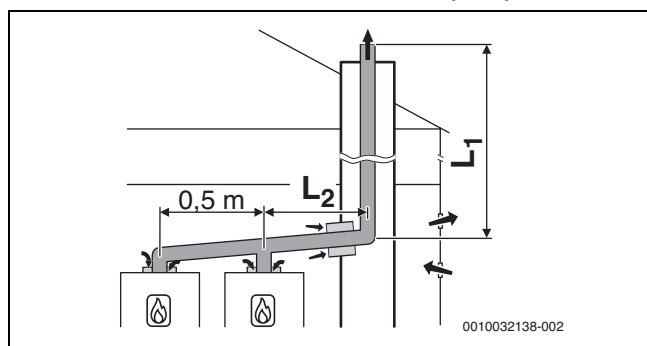
Рис. 77 Схема каскада с 2 котлами: жесткий отвод дымовых газов в шахте согласно B_{23}/B_{53p} с забором воздуха из помещения топочной для подвода воздуха
