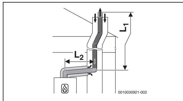
Рис. 25 Схема гибкого отвода дымовых газов согласно C_{93x} в шахте и концентрический подвод воздуха/отвод дымовых газов в помещении для установки
