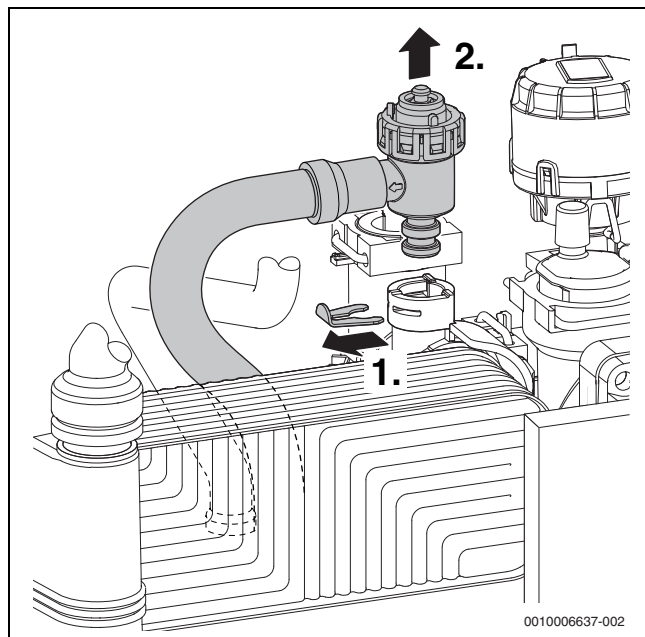
Рис. 106 Демонтаж предохранительного клапана (отопительного контура)
