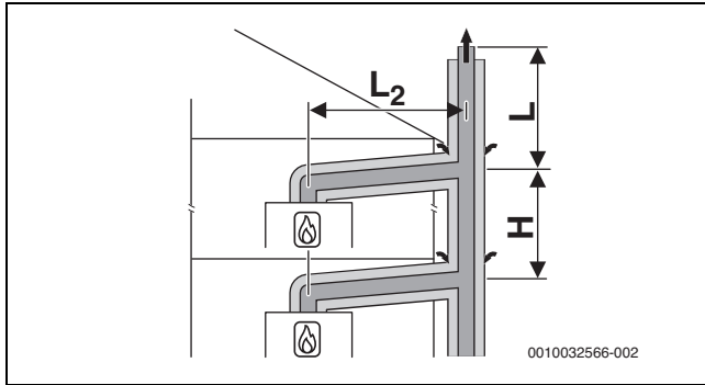
Рис. 74 Подключение нескольких котлов к одному дымоходу согласно C_{(13)3x} с концентрическим подводом воздуха/отводом дымовых газов по наружной стене и в помещении для установки
