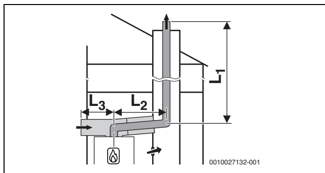
Рис. 57 Схема жесткого отвода дымовых газов согласно C_{53x} в шахте и схема подачи воздуха/отвода дымовых газов с отдельной линией подвода воздуха и концентрической линией отвода дымовых газов в помещении для установки
