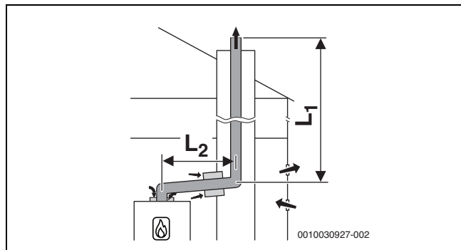
Рис. 66 Жёсткий отвод дымовых газов в шахте по B_{23p}/B_{53p} с забором воздуха из помещения и с концентрическим соединительным элементом между помещением установки котла и шахтой
