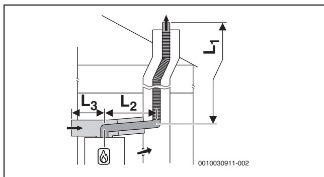
Рис. 15 Схема гибкого отвода дымовых газов согласно C_{53x} в шахте и схема подачи воздуха/отвода дымовых газов с отдельной линией подвода воздуха и концентрической линией отвода дымовых газов в помещении для установки
