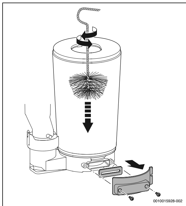
Рис. 97 Чистка теплообменника
