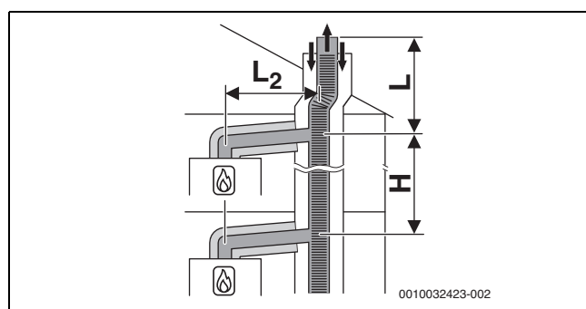
Рис. 38 Подключение нескольких котлов к одной дымовой трубе по C (14)3x с коллективным гибким отводом дымовых газов и концентрическим подводом воздуха/отводом дымовых газов в помещении установки оборудования
