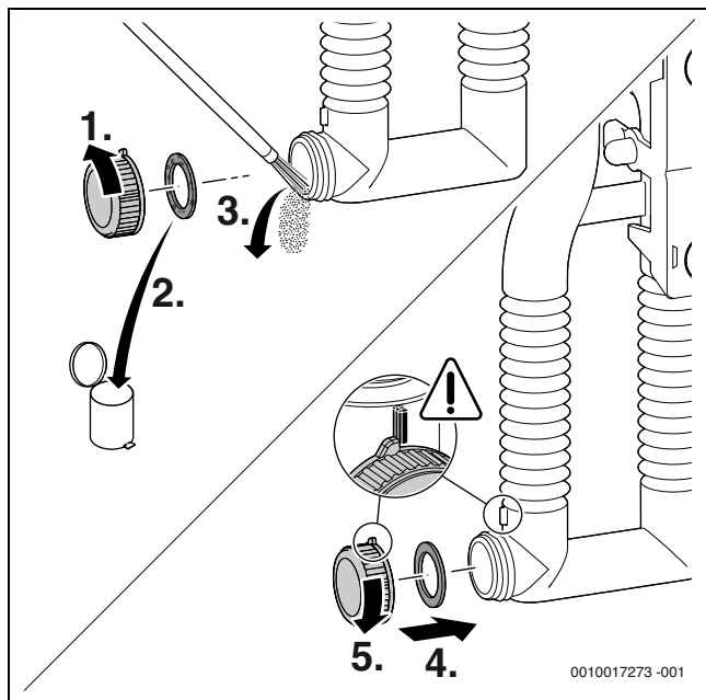
Рис. 101 Чистка конденсатного сифона
