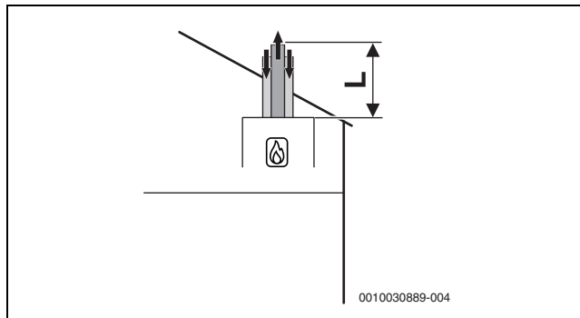
Рис. 50 Вертикальная концентрическая схема подачи воздуха/отвода дымовых газов согласно C 33x
