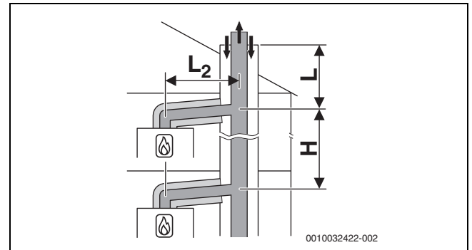
Рис. 75 Подключение нескольких котлов к одному дымоходу согласно C_{(14)3x} с коллективным жестким подводом воздуха/отводом дымовых газов в помещении для установки
