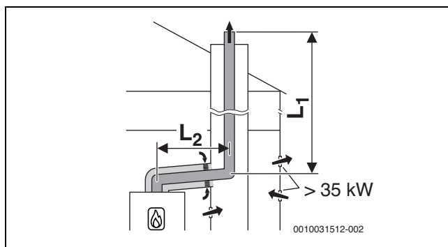
Рис. 32 Схема жесткого отвода дымовых газов в шахте согласно B 33 с забором воздуха из помещения через концентрический подвод воздуха/отвод дымовых газов в помещении для установки
