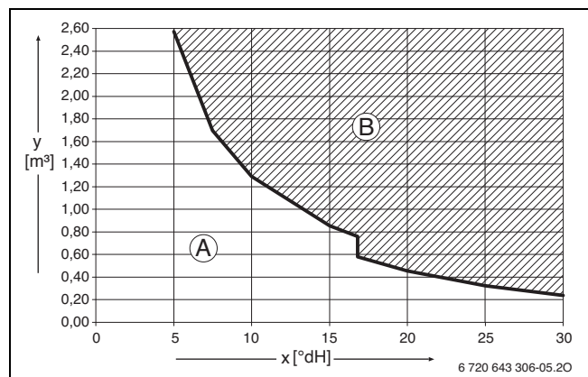
Рис. 80 Требования к воде для заполнения и подпитки в °dH для котлов < 50 кВт
