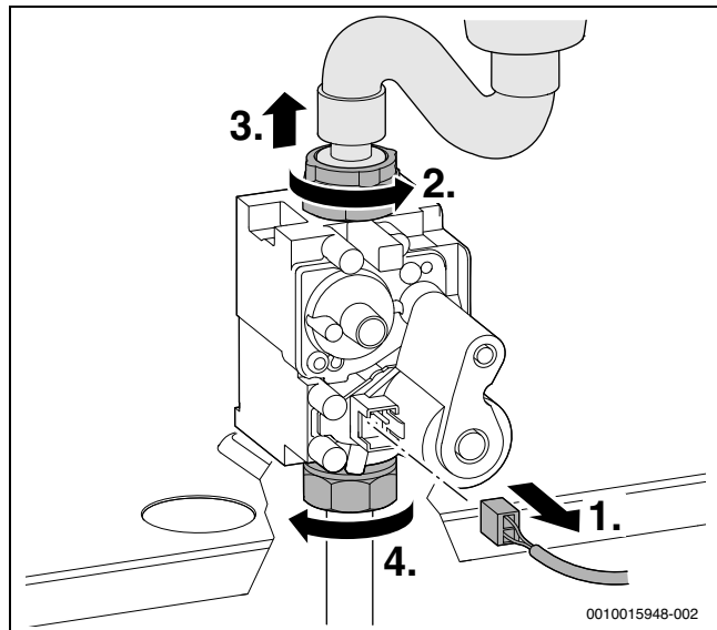
Рис. 109 Извлечение штекера и отвинчивание накидных гаек
