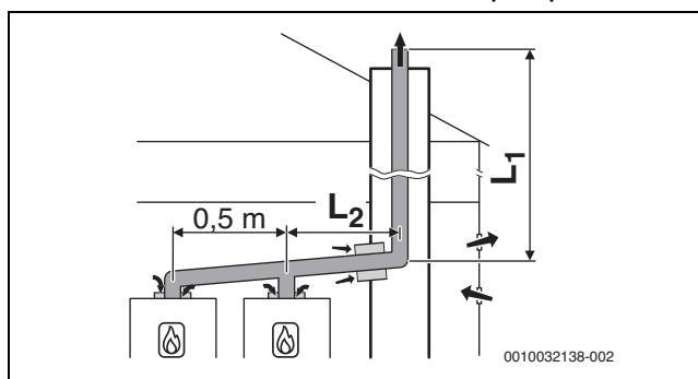
Рис. 39 Схема каскада с 2 котлами:
