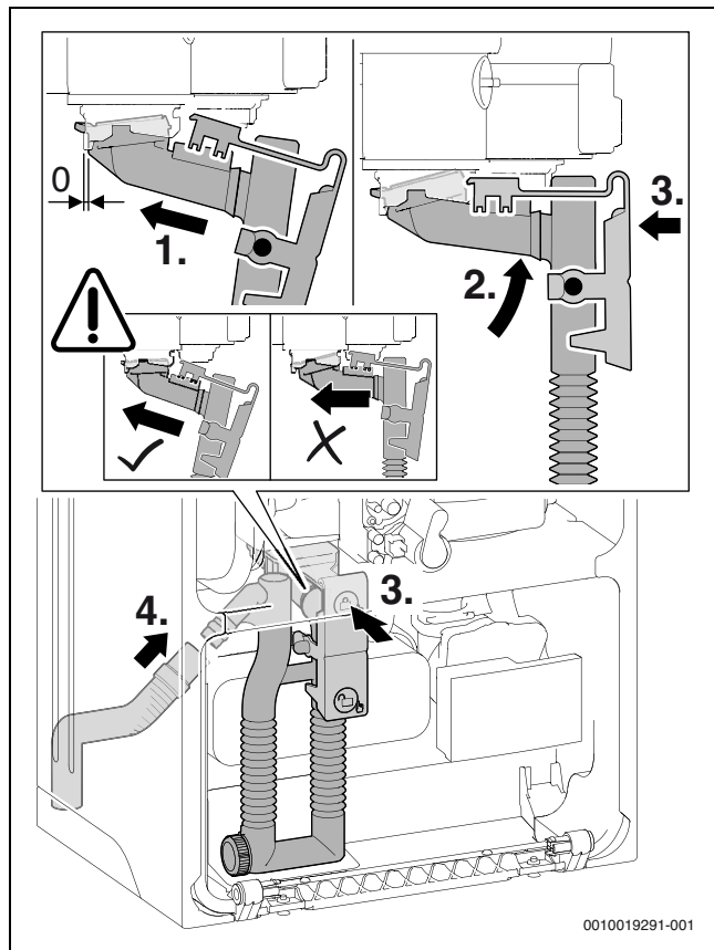
Рис. 105 Установка сифона для отвода конденсата
