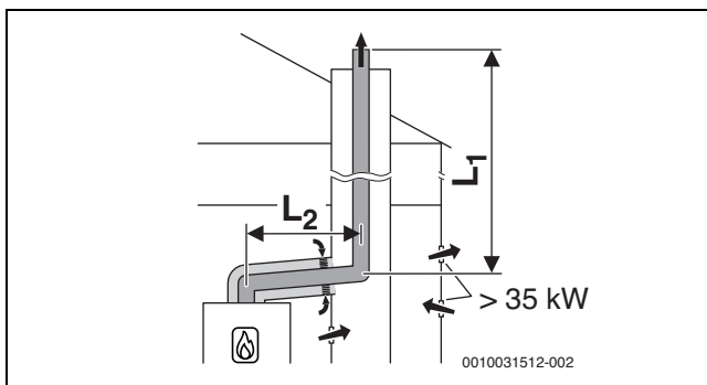
Рис. 70 Схема жесткого отвода дымовых газов в шахте согласно В 33 с забором воздуха из помещения через концентрический подвод воздуха/отвод дымовых газов в помещении для установки
