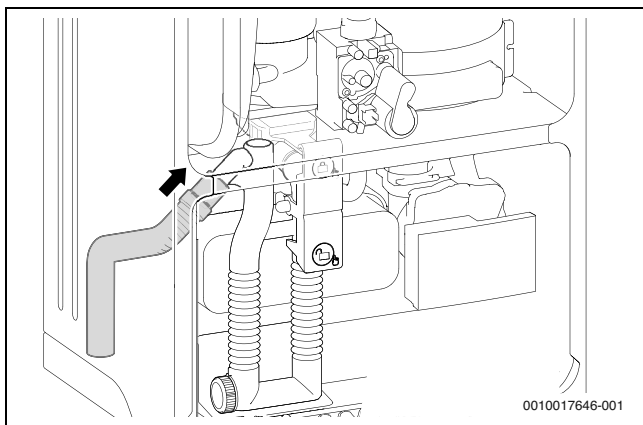
Рис. 85 Подсоединение шланга к сифону для отвода конденсата
