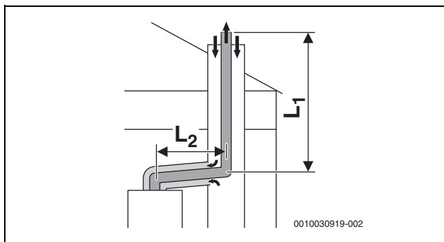
Рис. 26 Схема жесткого отвода дымовых газов согласно C_{93x} в шахте и концентрический подвод воздуха/отвод дымовых газов в помещении для установки
