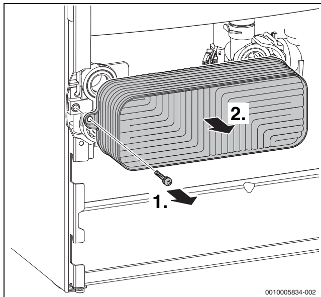
Рис. 108 Демонтаж пластинчатого теплообменника
