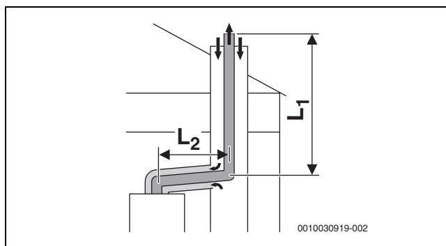
Рис. 64 Схема жесткого отвода дымовых газов согласно C 93x в шахте и концентрический подвод воздуха/отвод дымовых газов в помещении для установки
