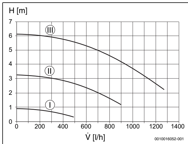
Рис. 87 Характеристическая кривая насоса отопительного контура (постоянная частота вращения)
