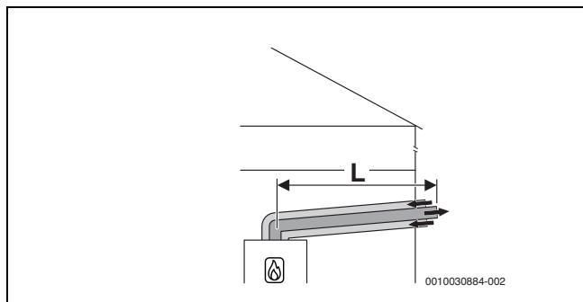
Рис. 8 Горизонтальная концентрическая схема подачи воздуха/отвода дымовых газов согласно C 13x через наружную стену
