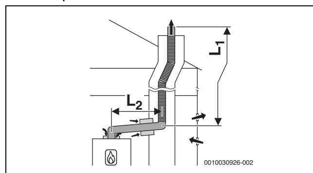
Рис. 29 Схема гибкого отвода дымовых газов в шахте согласно B_{23p}/B_{53p} с забором воздуха из помещения топочной для подвода воздуха и с концентрическим соединительным участком между помещением для установки и шахтой
