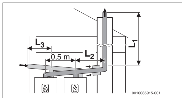
Рис. 40 Схема каскада с 2 котлами
