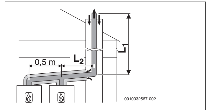
Рис. 79 Схема каскада с 2 котлами: Схема жесткого отвода дымовых газов согласно C_{93x} в шахте и концентрический подвод воздуха/отвод дымовых газов в помещении для установки
