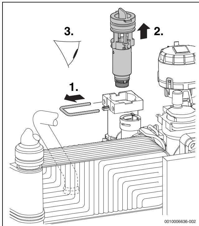
Рис. 107 Проверка сетчатого фильтра в трубе холодной воды
