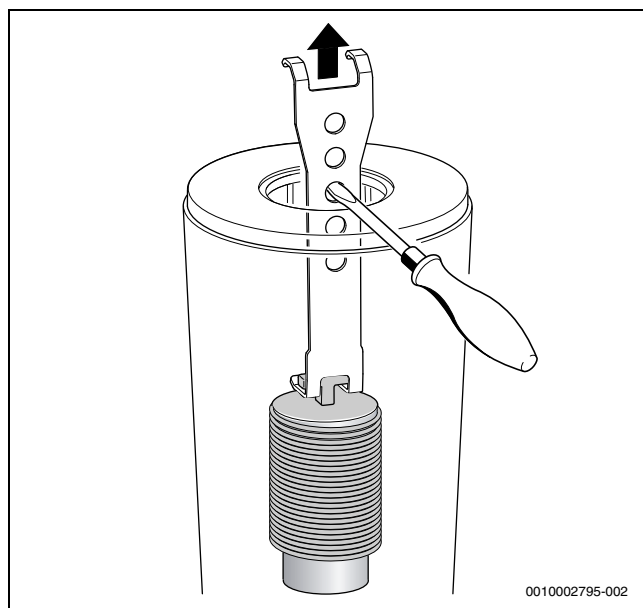
Рис. 96 Выньте нижний рассекатель
