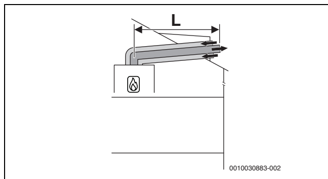
Рис. 45 Горизонтальная концентрическая схема подачи воздуха/отвода дымовых газов согласно C 13x через крышу
