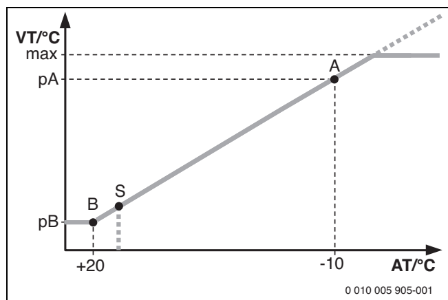
Рис. 120 Отопительная кривая
