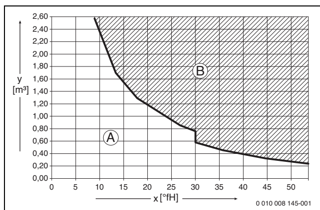
Рис. 81 Требования к воде для заполнения и подпитки в °fH для котлов < 50 кВт
