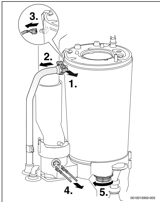
Рис. 114 Отсоедините трубу подающей линии и провода
