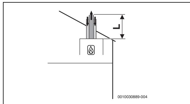
Рис. 10 Вертикальная концентрическая схема подачи воздуха/отвода дымовых газов согласно C_{33x}
