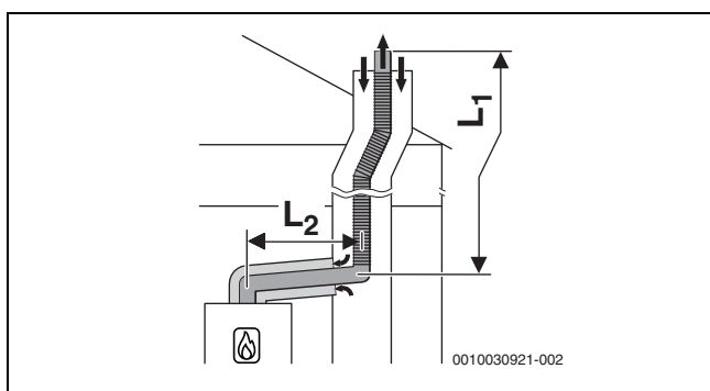
Рис. 27 Схема гибкого отвода дымовых газов согласно C_{93x} в шахте и концентрический подвод воздуха/отвод дымовых газов в помещении для установки
