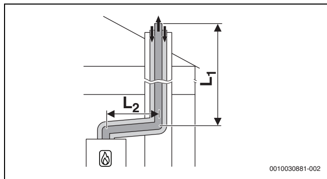
Рис. 11 Концентрическая схема подачи воздуха/отвода дымовых газов согласно C_{33x} в шахте
