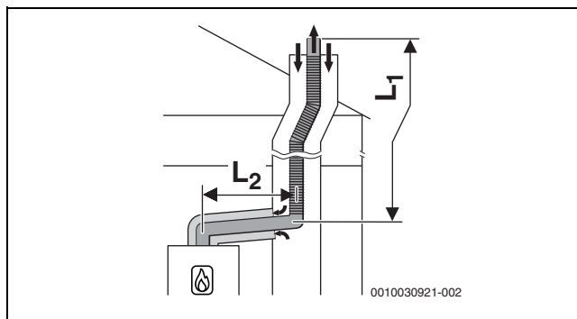
Рис. 65 Схема гибкого отвода дымовых газов согласно C 93x в шахте и концентрический подвод воздуха/отвод дымовых газов в помещении для установки
