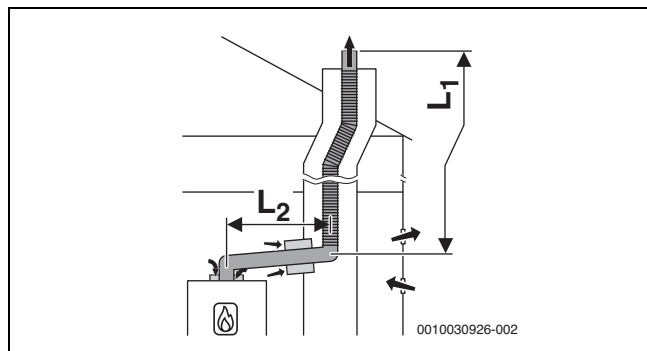
Рис. 31 Схема гибкого отвода дымовых газов в шахте согласно B 23p /B 53p с забором воздуха из помещения топочной для подвода воздуха и с концентрическим соединительным участком между помещением для установки и шахтой
