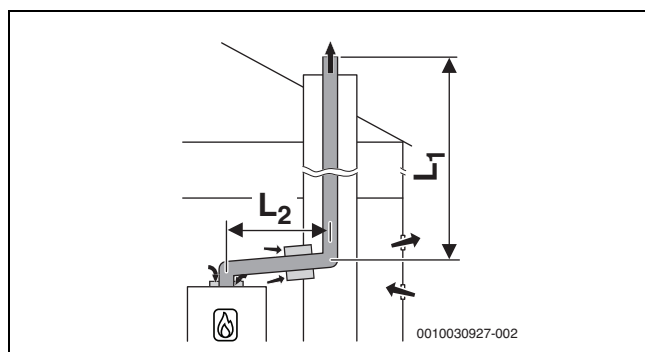
Рис. 28 Жёсткий отвод дымовых газов в шахте по B_{23p}/B_{53p} с забором воздуха из помещения и с концентрическим соединительным элементом между помещением установки котла и шахтой
