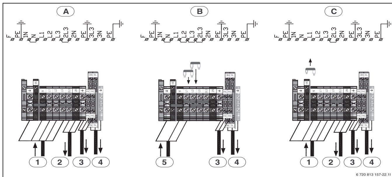
Rys. 31 Zaciski przyłączeniowe
