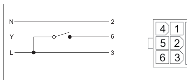
Rys. 22 wtyczka Molex
