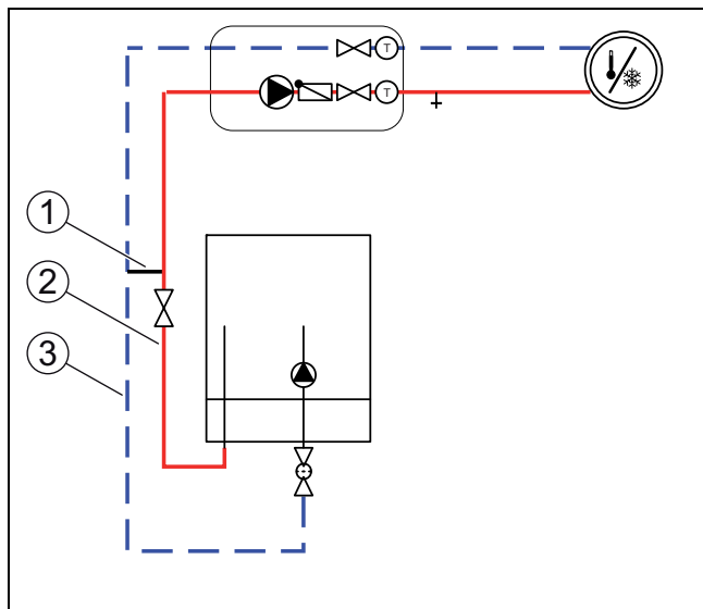
Rys. 24 Jednostka wewnętrzna z obiegiem grzewczym i obejściem
