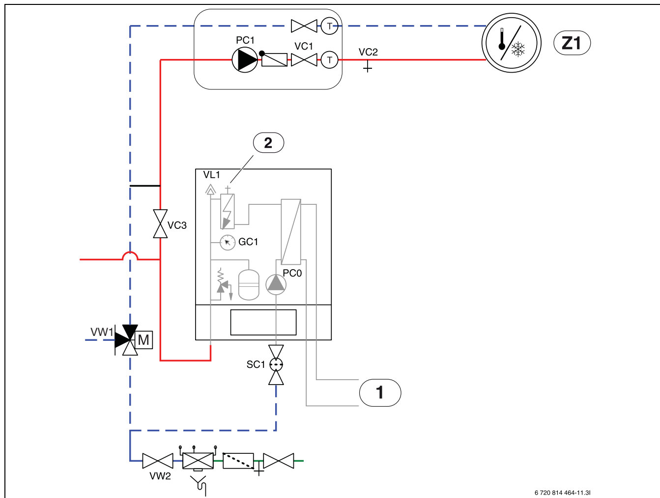
Rys. 14 Jednostka wewnętrzną ze zintegrowaną grzałką elektryczną i instalacją ogrzewczą
