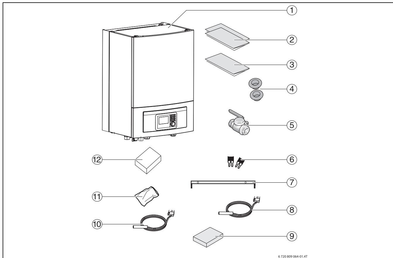
Rys. 1 Zakres dostawy
