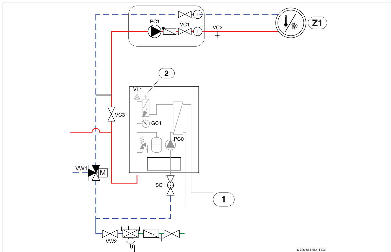
Rys. 8 Jednostka wewnętrzną ze zintegrowaną grzałką elektryczną i system grzewczy
