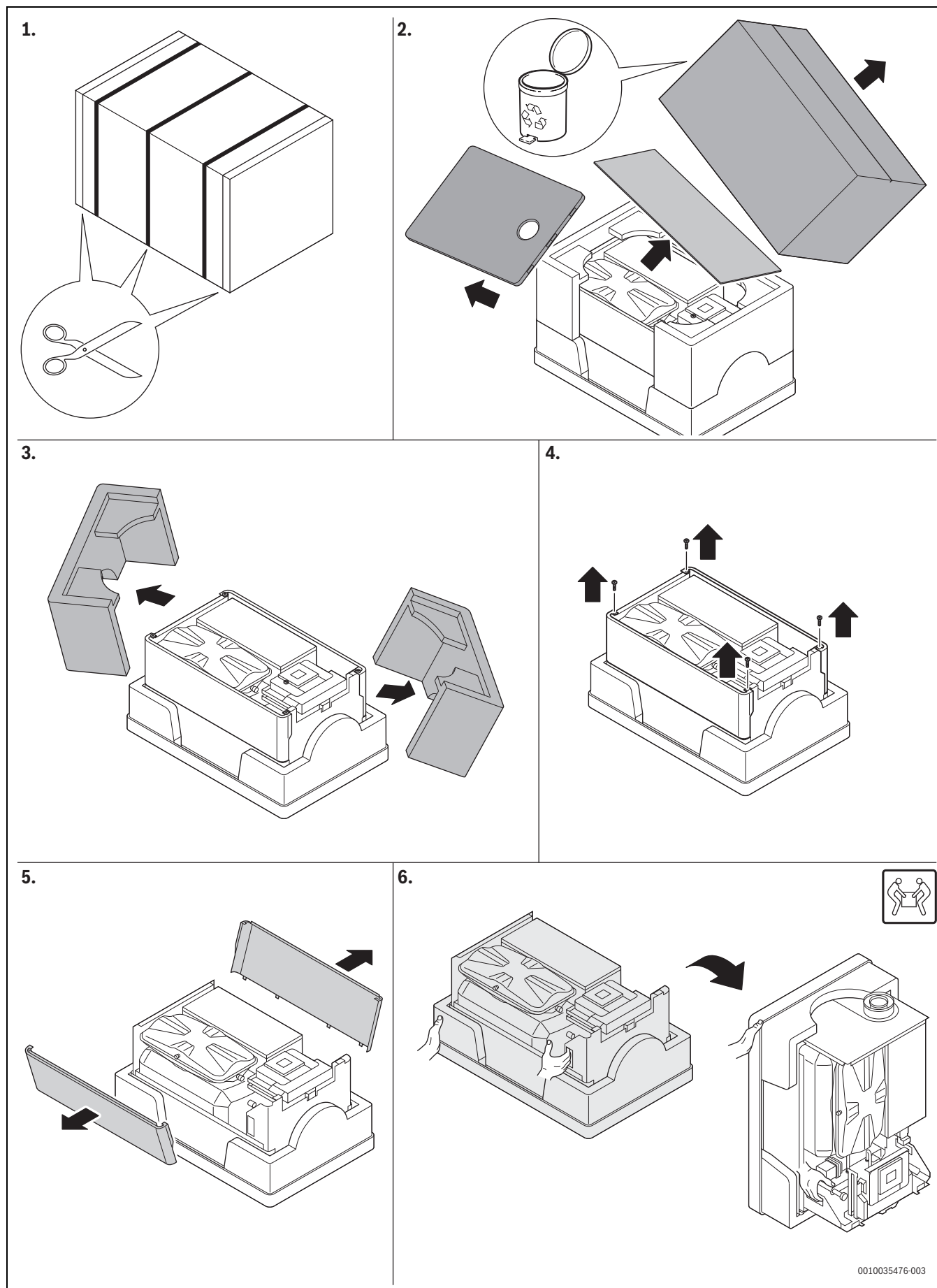
Rys. 32 Instrukcja rozpakowywania
