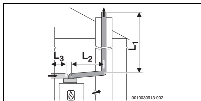
Rys. 15 Sztywne odprowadzenie spalin wg C 53 w szachcie i instalacja powietrzno-spalinowa z odesparowanymi rurami dla dopływu powietrza i odprowadzenia spalin w pomieszczeniu zainstalowania
