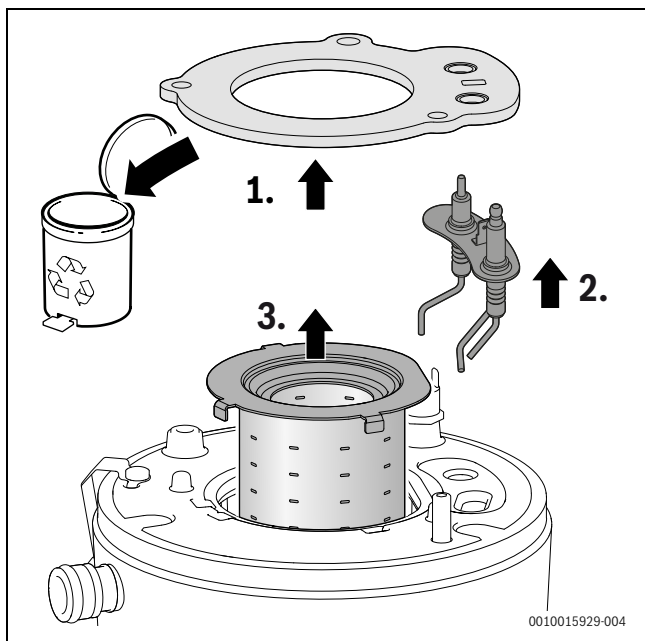
Rys. 62 Wyjmowanie palnika
