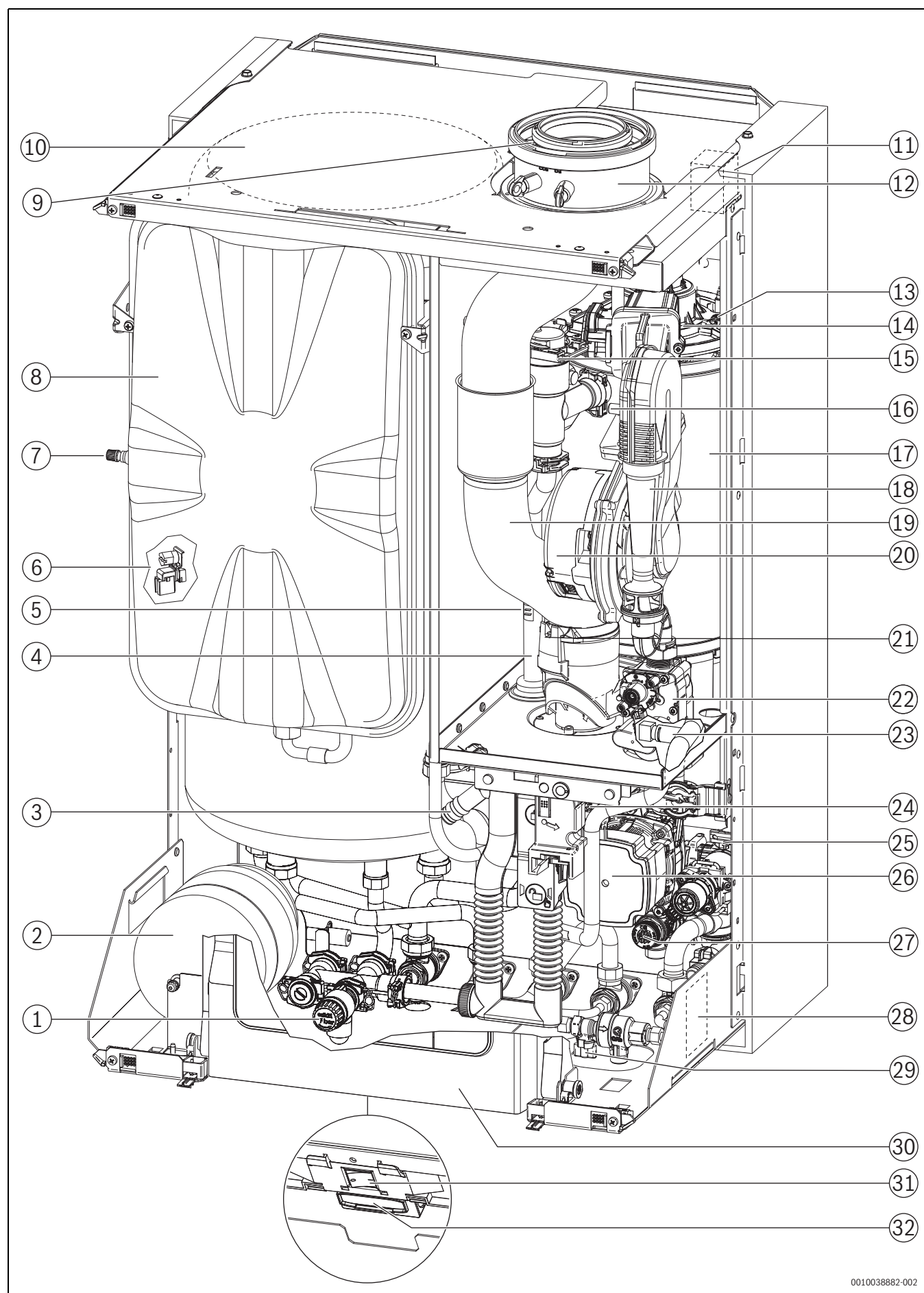
Rys. 5 Przegląd produktu
