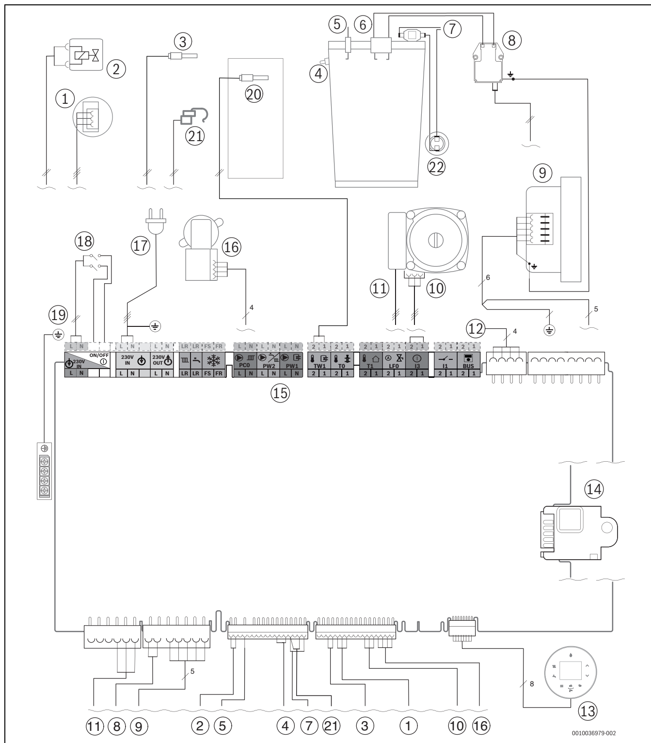
Rys. 91 Okablowanie elektryczne
