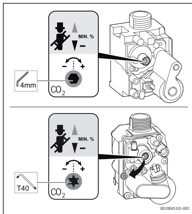
Rys. 55 Ustawianie stężenia \text{CO}_2/\text{O}_2 dla minimalnej znamionowej mocy cieplnej
