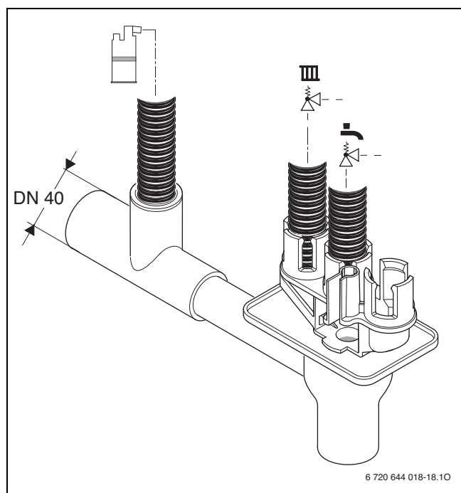
Rys. 39 Montaż węża kondensatu i węży zaworów bezpieczeństwa na syfonie
