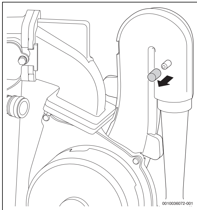
Rys. 57 Króciec pomiarowy na zespole mieszającym
