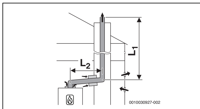
Rys. 20 Sztynne odprowadzenie spalin w szachcie wg B 23p /B 53p z zależnym od powietrza w pomieszczeniu doprowadzeniem powietrza do urządzenia i koncentryczną złączką między pomieszczeniem zainstalowania a szachtem
