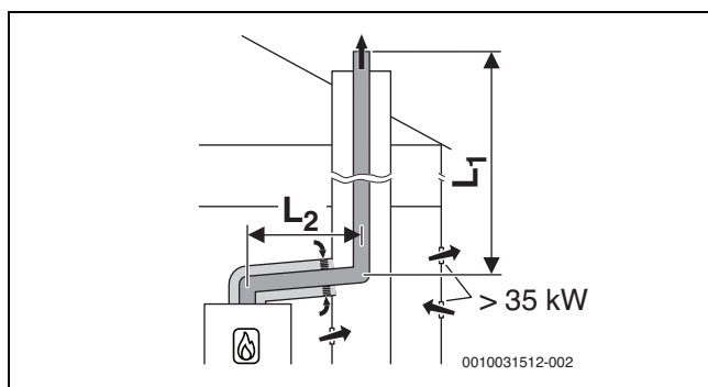
Rys. 22 Szttywne odprowadzenie spalin w szachcie wg B 33 z zależnym od powietrza w pomieszczeniu doprowadzeniem powietrza przez koncentryczną instalację powietrzno-spalinową w pomieszczeniu zainstalowania
