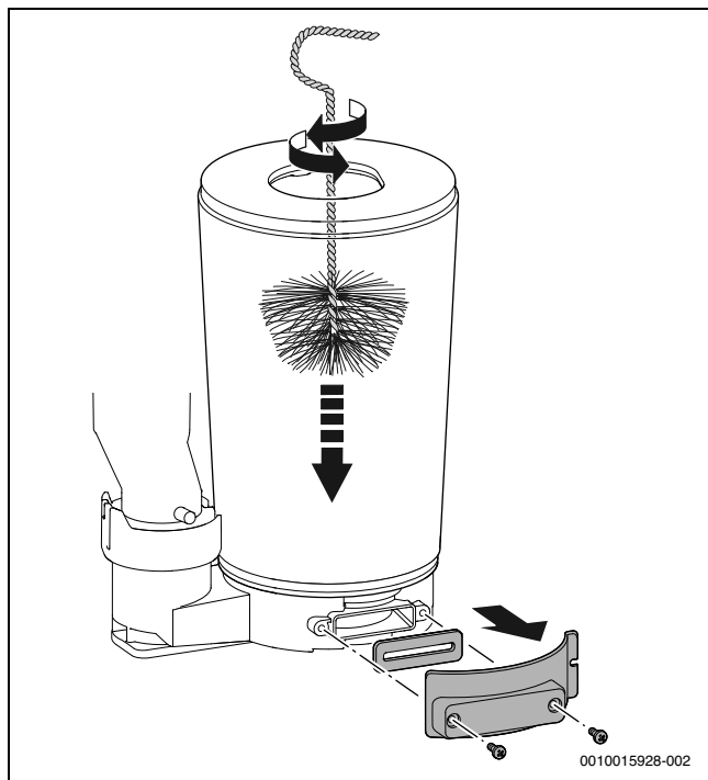
Pav. 49 Šiluminio bloko valymas
