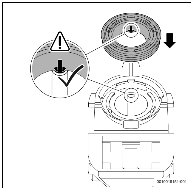
Pav. 55 Naujos sandarinimo detalės ant kondensato sifono uždėjimas
