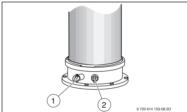
Pav. 41 Išmetamųjų dujų matavimo atvamzdis ir degimui naudojamą oro matavimo atvamzdį
