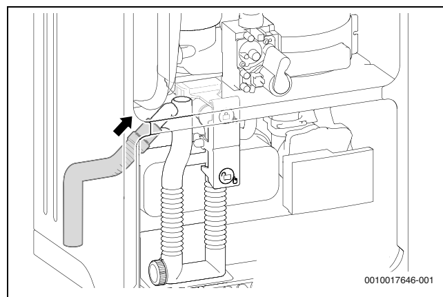
Pav. 26 Žarnos prie kondensato sifono montavimas
