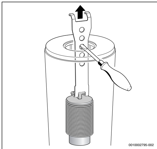
Pav. 48 Apatinio liepsnos kreiptuvo išėmimas
