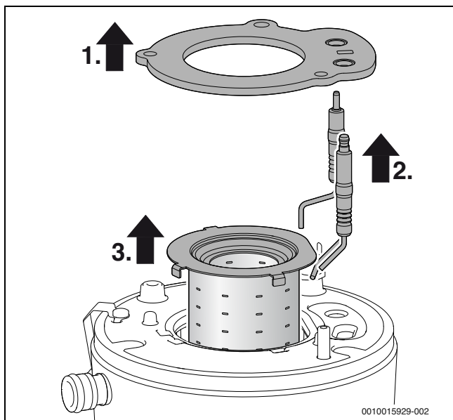
Pav. 46 Degiklio išėmimas
