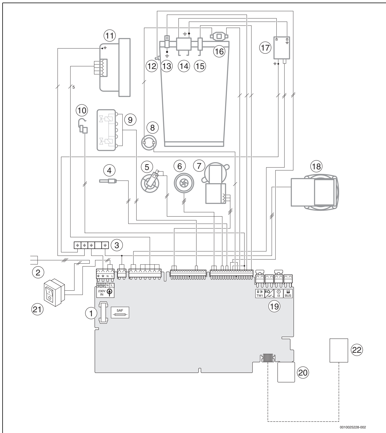
Pav. 73 Elektros laidų montavimas
