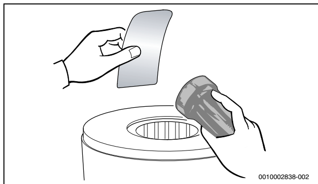
Pav. 50 Šilumos bloko patikra, ar nėra nuosėdų
