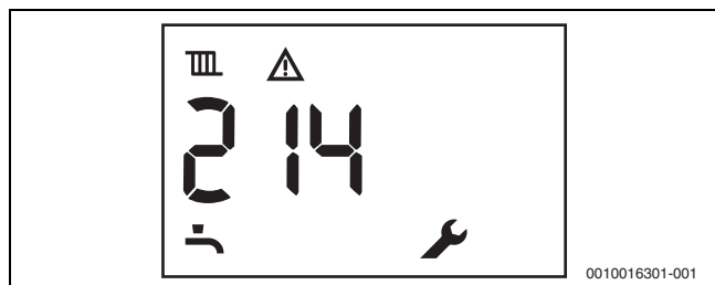
Pav. 72 Pavyzdys: neblokuojanti triktis
