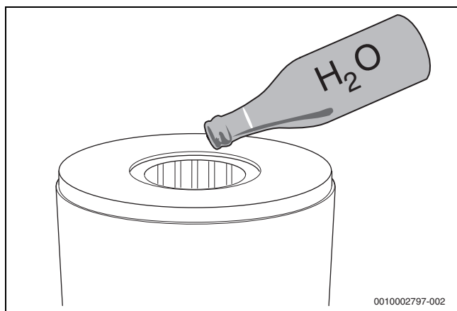
Pav. 51 Šilumos bloko praskalavimas vandeniu
