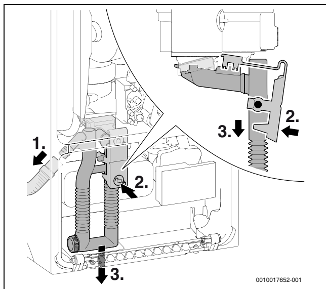
Pav. 52 Kondensato sifono išmontavimas
