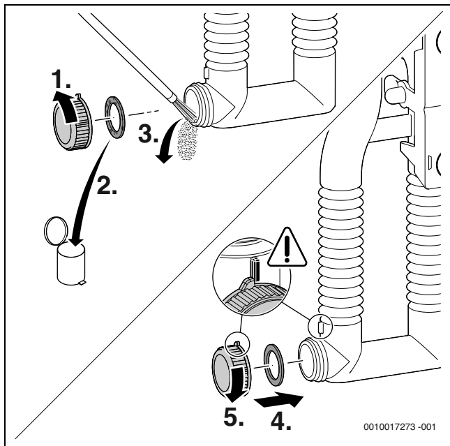
Pav. 53 Kondensato sifono valymas
