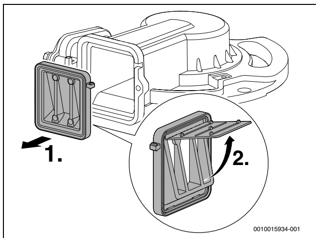
Pav. 45 Atbulinė sklendė maišymo įrenginyje
