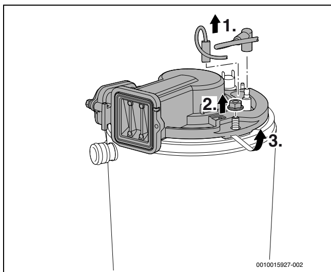
Pav. 44 Degiklio dangčio nuėmimas
