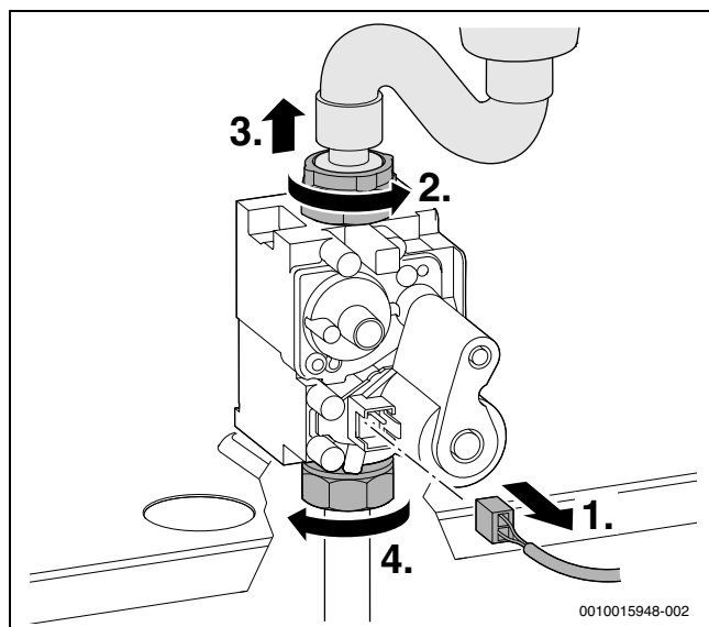
Pav. 61 Kištuko ištraukimas ir gaubiamųjų veržlių nuėmimas
