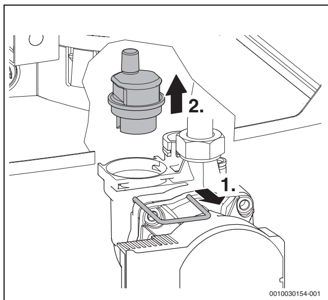
Pav. 64 Automatinio oro išleidimo įtaiso išmontavimas
