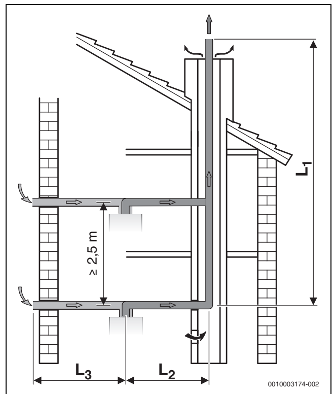
Pav. 20 Būdas, kai prie dūmtraukio jungiami keli įrenginiai su atskiru vamzdžiu, pagal C 83
