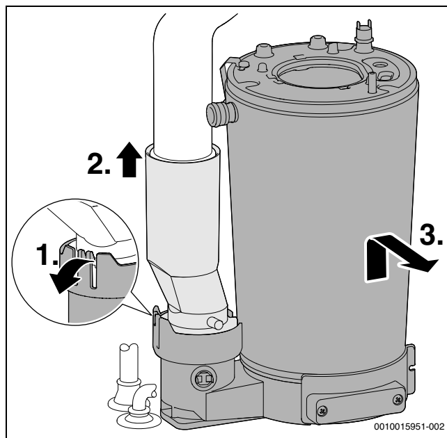
Att. 67 Katla bloka demontāža
