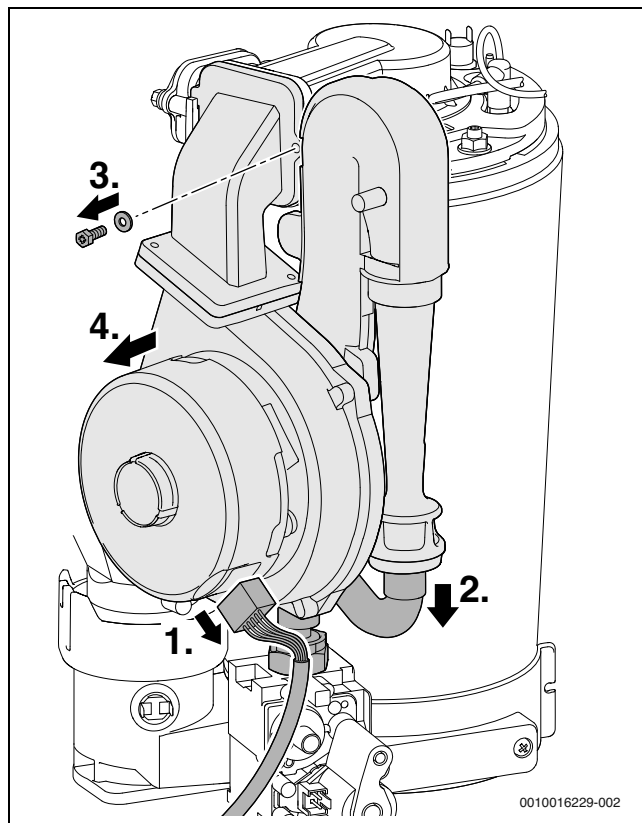
Att. 43 Ventilatora ar samaisīšanas kameru demontāža
