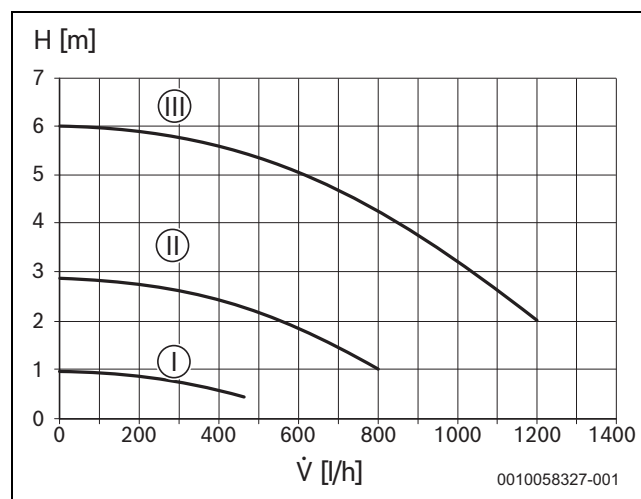
Att. 36 Apkures sūkņa raksturlikne (nemainīgs spiediens)
