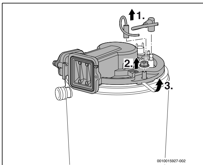
Att. 44 Degļa virsmas noņemšana
