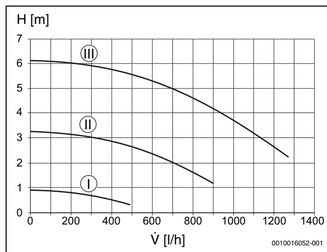
Att. 35 Apkures sūkņa raksturīgā (nemainīgs apgriezienu skaits)
