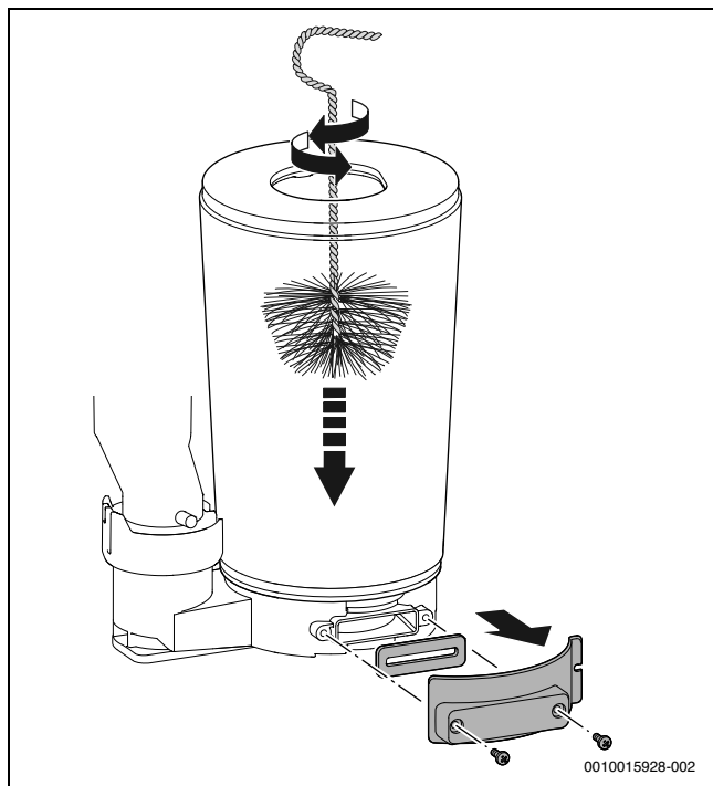
Att. 49 Katla bloka tīrīšana
