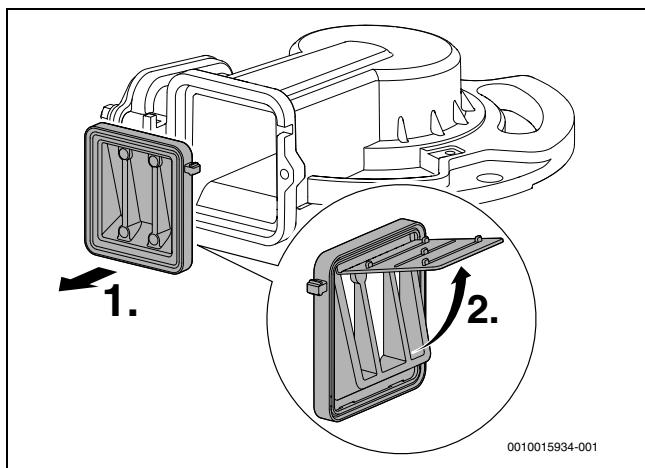
Att. 45 Pretvārsts samaisīšanas kamerā
