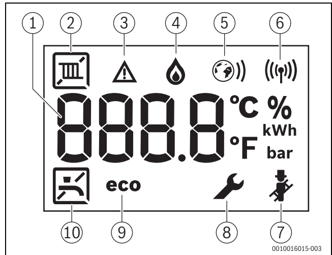
Att. 33 Displeja rādījumi
