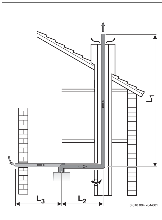
Att. 11 Dūmgāzu novadišana šāhtā atbilstoši C 53
