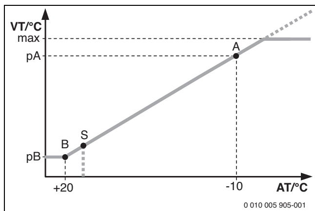
Att. 74 Apkures līkne
