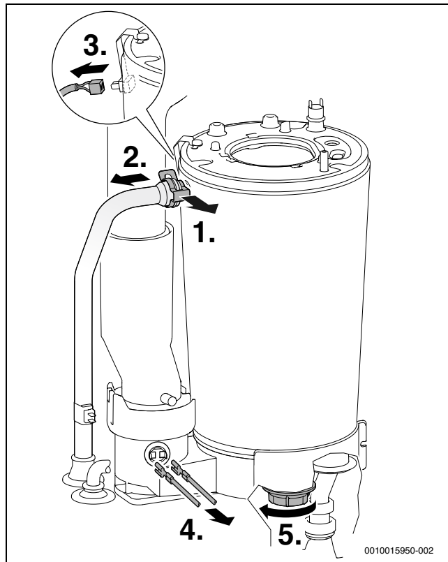
Att. 66 Atbrīvojiet turpgaitas cauruli un noņemiet kabeli.
