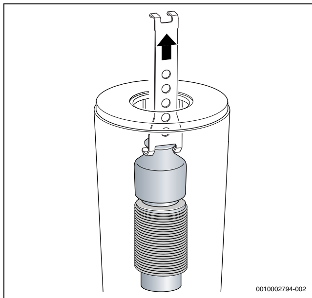
Att. 47 Augšējā liesmas novirzītāja izņemšana
