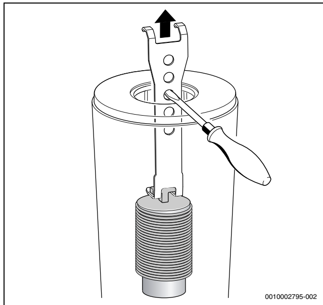
Att. 48 Apakšējā liesmas novirzītāja izņemšana
