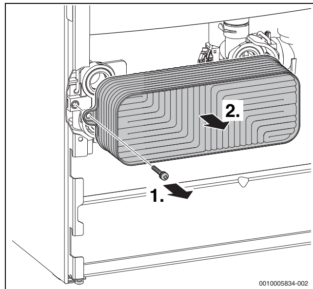
Att. 60 Plāksņu siltummaiņa demontēšana
