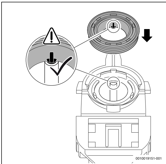
Att. 55 Jaunā blīvējuma uzlikšana uz kondensāta sifona
