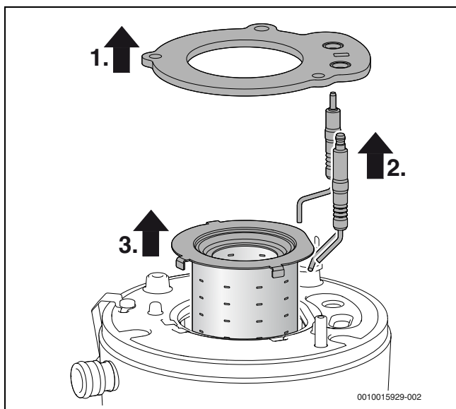
Att. 46 Degļa izņemšana
