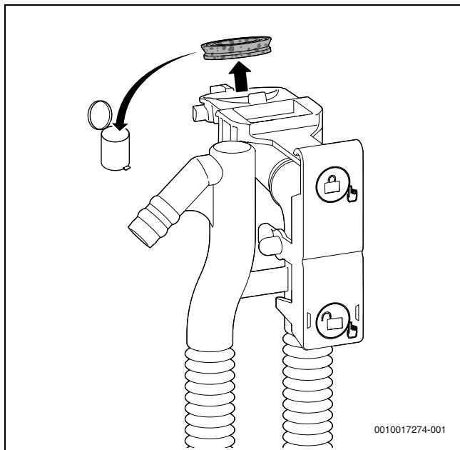
Att. 54 Blīvējuma nomaiņa augšā pie kondensāta sifona
