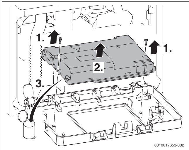
Att. 68 Pārsega noņemšana un vadības plates nomainīšana
