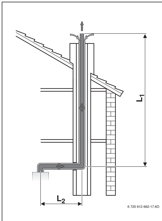
Att. 10 Dūmgāzu novadišanas sistēma ar koncentrisku cauruli šāhtā atbilstoši C 33
