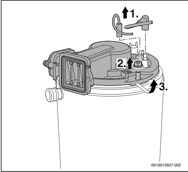
Res. 37 Brülör kapağının çözülmesi
