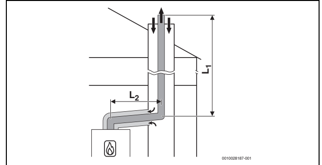
Res. 9 Havalandırma boşluğunda C 93x uyarınca sabit atık gaz tahliyesi ve kurulum yerinde konsantrik hava-atık gaz taşıma sistemi
