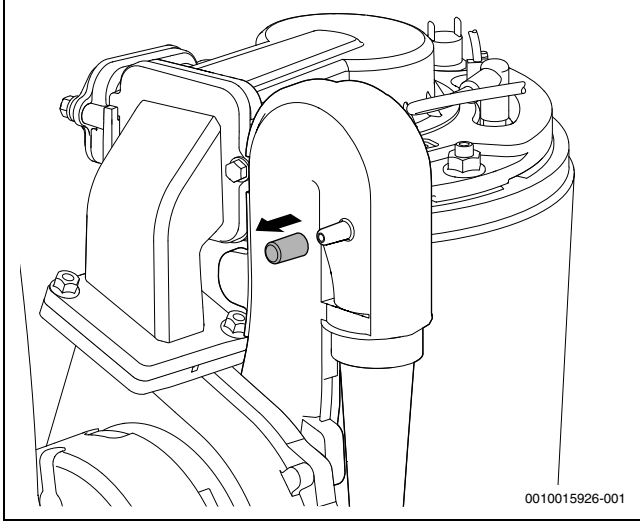
Res. 35 Karıştırma ünitesindeki ölçüm ağzı
