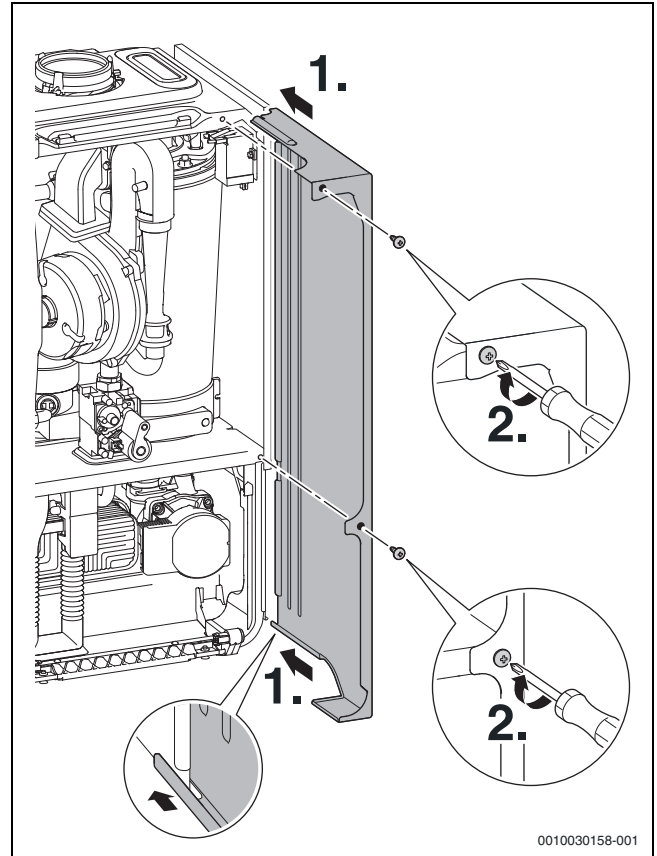
Res. 63 Yan dış sacın tekrar takılması
