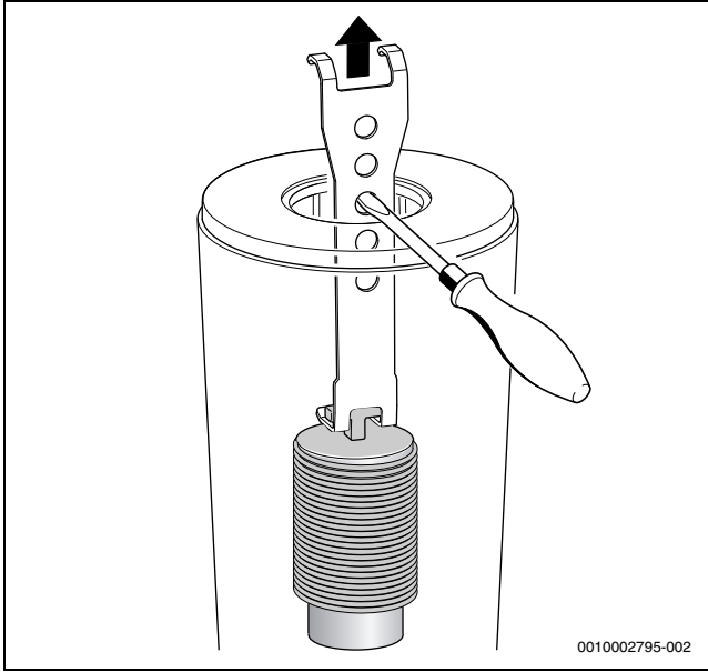
Res. 41 Alttaki atık gaz yönlendiricisinin çıkarılması
