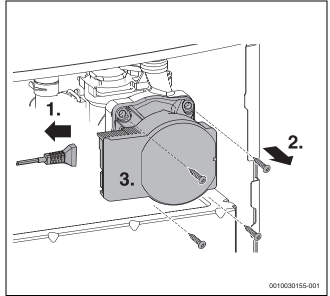
Res. 56 Sirkülasyon pompasının sökülmesi
