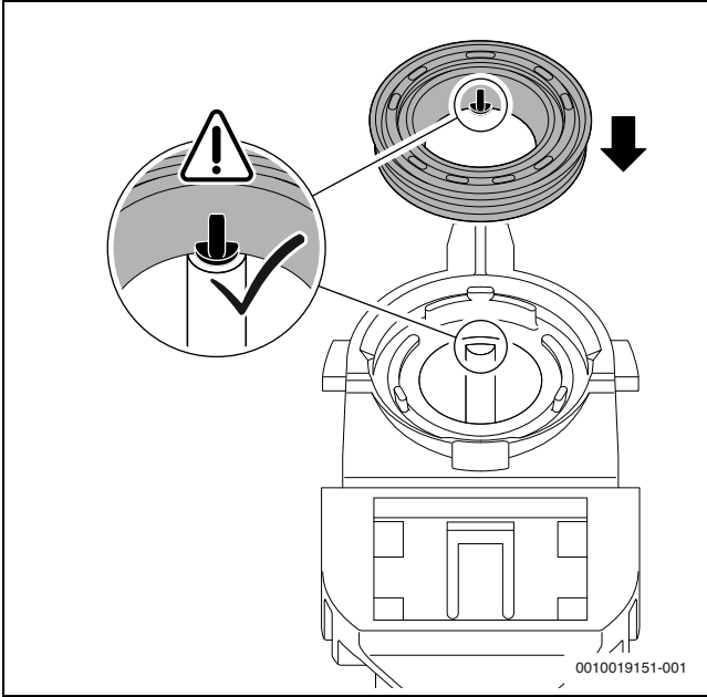
Res. 48 Yeni contanın yağuşma suyu sifonunda doğru konumlandırılması
