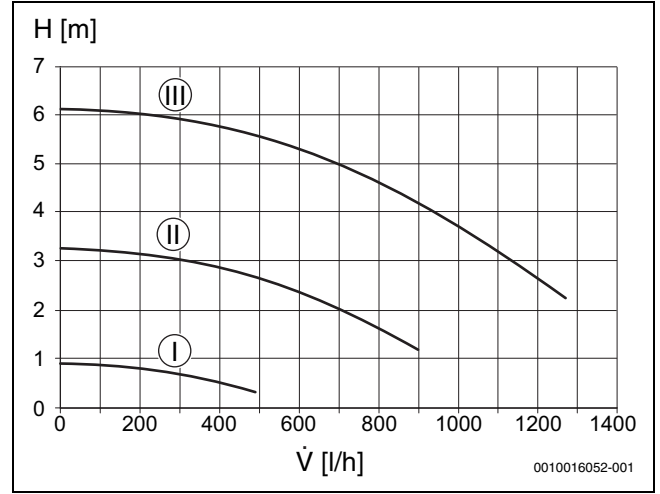
Res. 27 Sirkülasyon pompası karakteristik eğrisi (sabit devir sayısı)
