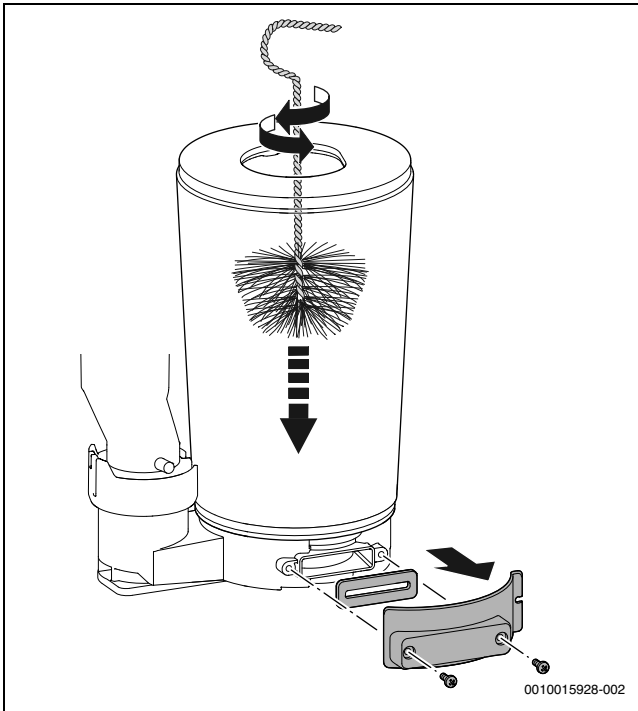
Res. 42 Isı bloğunun temizlenmesi
