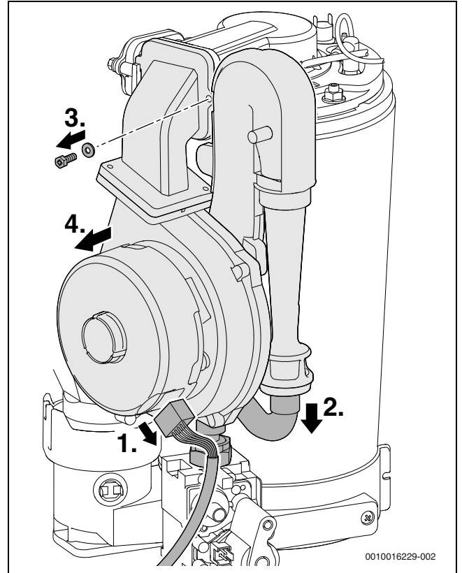
Res. 36 Karıştırma ünitesi ile birlikte fanın sökülmesi
