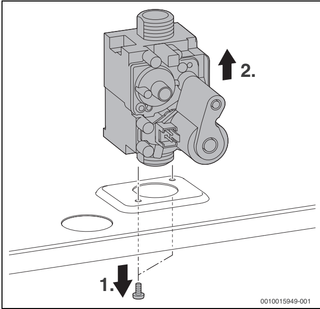
Res. 55 Gaz armatürünün sökülmesi
