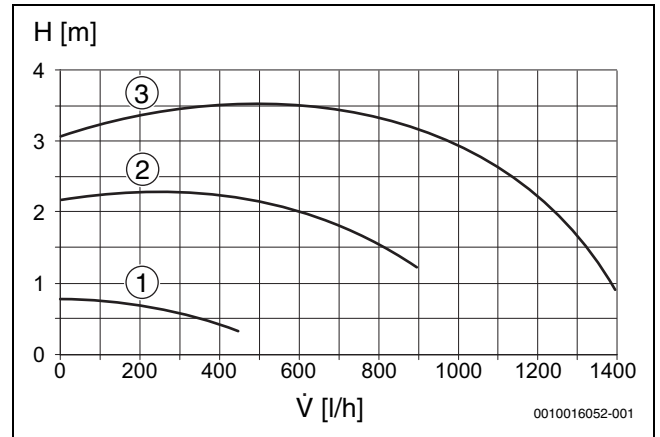
Res. 29 Sirkülasyon pompası karakteristik eğrisi (oransal basınç)
