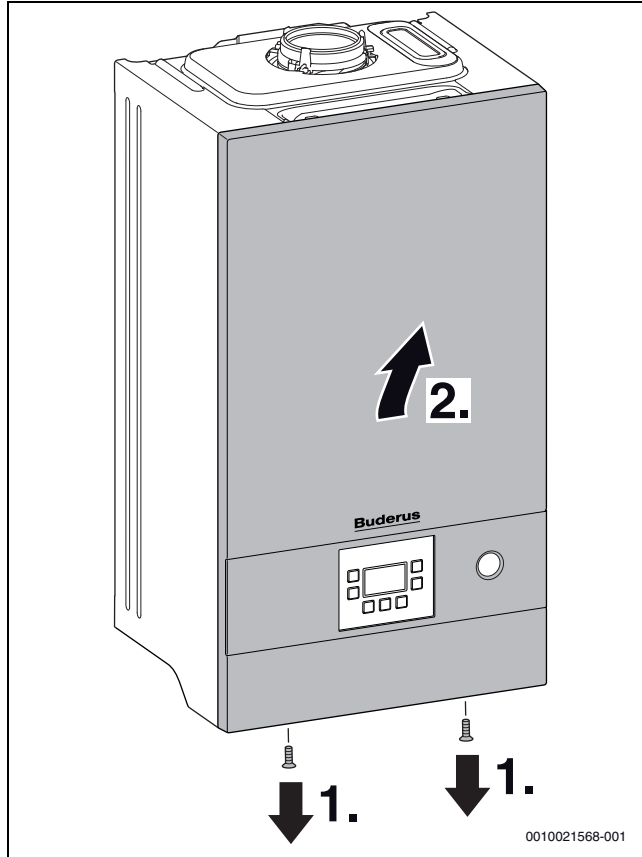
Res. 16 Ön dış sacın çıkarılması
