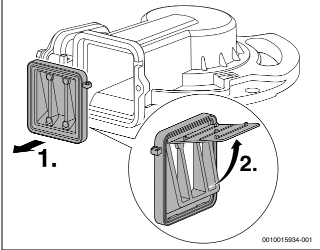
Res. 38 Karıştırma ünitesindeki çekvalf
