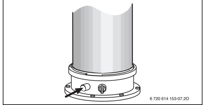
Res. 30 Atık gaz ölçüm ağızı
