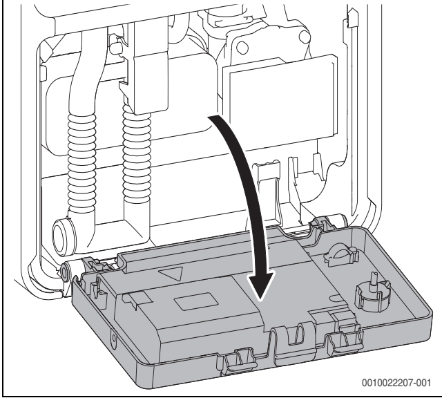
Res. 21 Elektronik sisteminin aşağı doğru açılması
