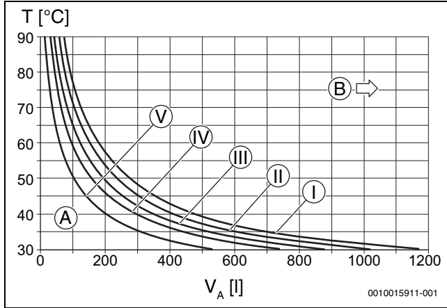
Res. 15 Genleşme tankının karakteristik eğrileri
