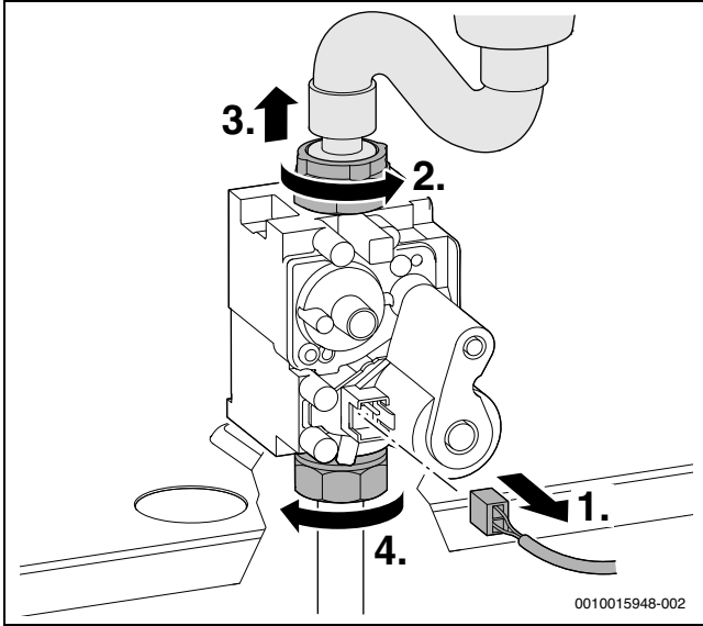
Res. 54 Fişin çekilmesi ve rakor somunların çözülmesi
