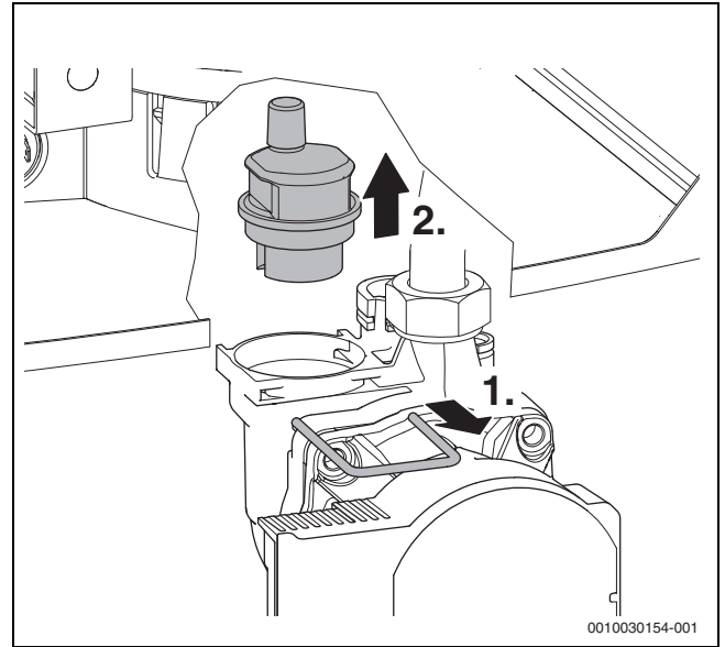
Res. 57 Otomatik hava pürjörünün sökülmesi
