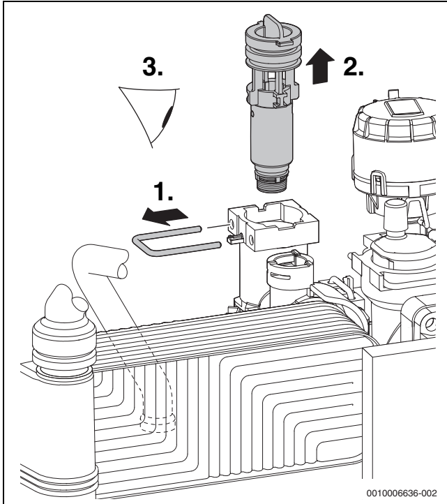
Res. 52 Soğuk su borusundaki süzgecin kontrol edilmesi
