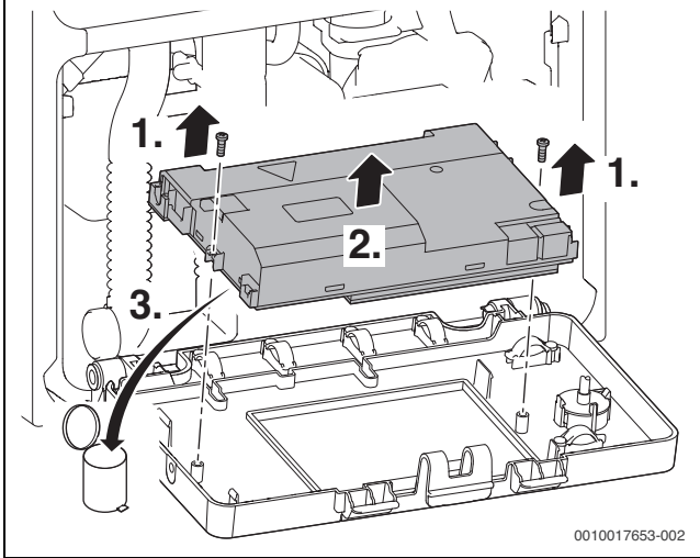
Res. 61 Muhafaza kapağının çıkarılması ve elektronik devre kartın değiştirilmesi
