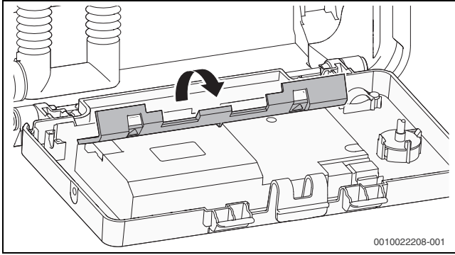
Res. 22 Kapağın açılması
