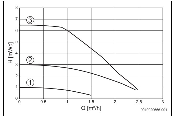
Res. 28 Sirkülasyon pompasının karakteristik eğrisi (sabit basınç)
