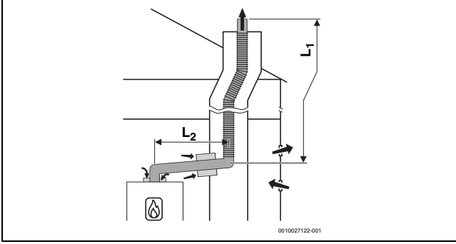
Res. 12 Cihazda oda havasına bağlı hava beslemeli ve kurulum yeri ile havalandırma boşluğu arasında konsantrik bağlantı parçalı, havalandırma boşluğunda B 23p /B 53p uyarınca esnek atık gaz tahliyesi
