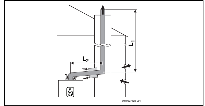
Res. 11 Cihazda oda havasına bağlı hava beslemeli ve kurulum yeri ile havalandırma boşluğu arasında konsantrik bağlantı parçalı, havalandırma boşluğunda B 23p /B 53p uyarınca sabit atık gaz tahliyesi
