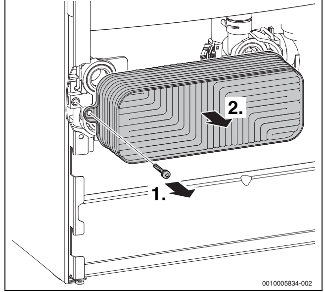
Res. 53 Plakalı eşanjörün sökülmesi
