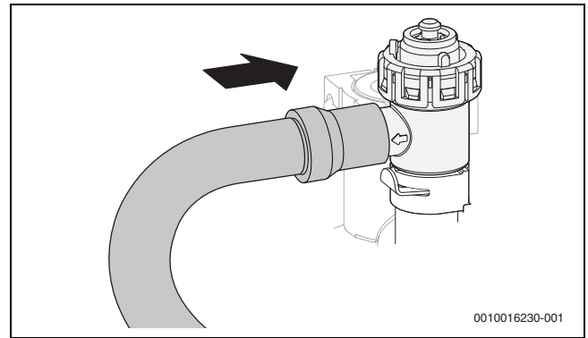
Res. 17 Emniyet ventili hortumunun monte edilmesi
