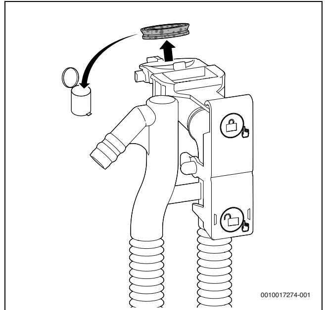
Res. 47 Yoğuşma suyu sifonundaki üst contanın değiştirilmesi
