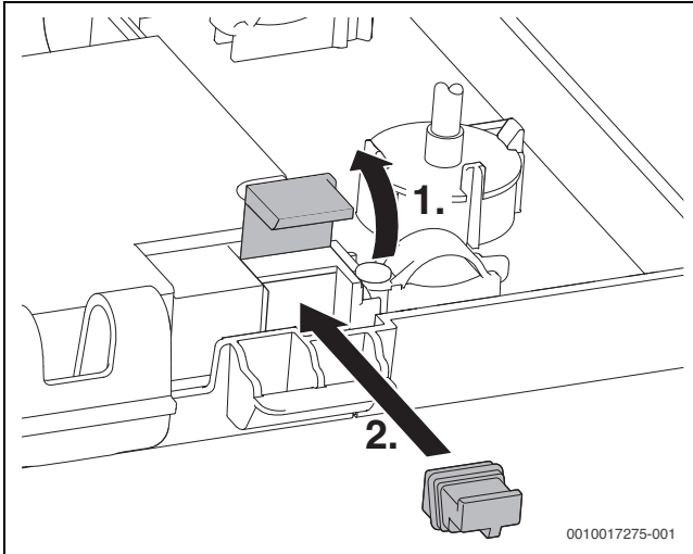
Res. 62 Kod anahtarının takılması
