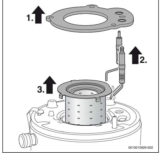
Res. 39 Brülörün çıkartılması
