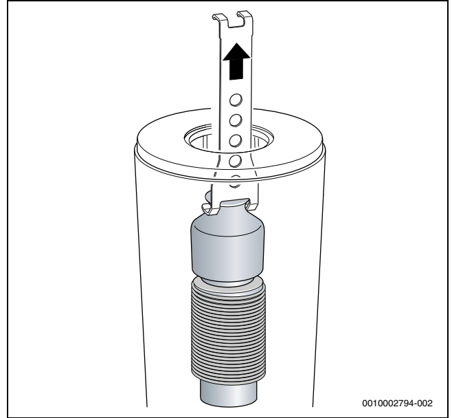
Res. 40 Üstteki atık gaz yönlendiricisinin çıkarılması
