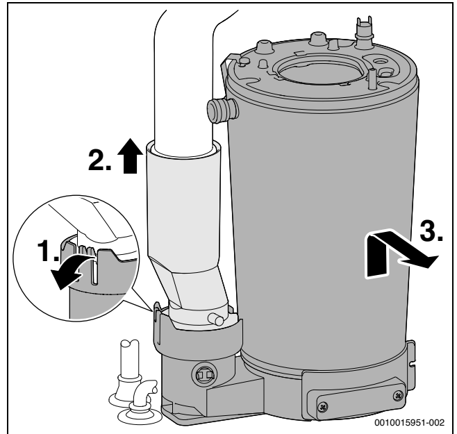
Res. 60 Isı bloğunun sökülmesi
