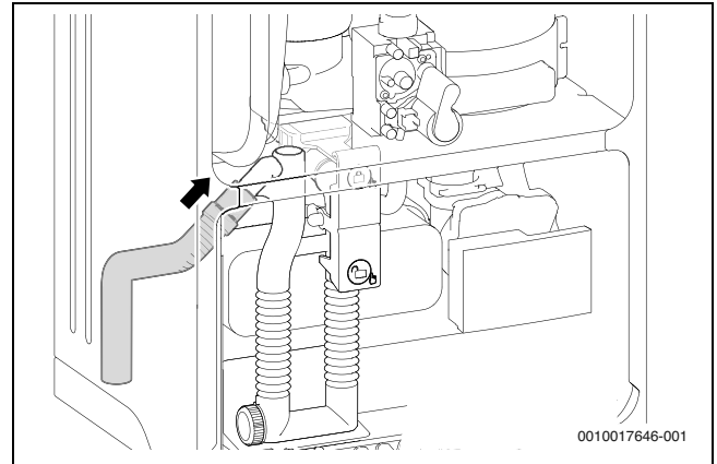
Res. 18 Hortumun yoğuşma suyu sifonuna monte edilmesi
