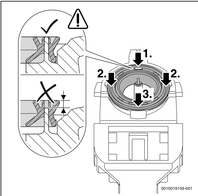
Res. 49 Contanın bastırılması
