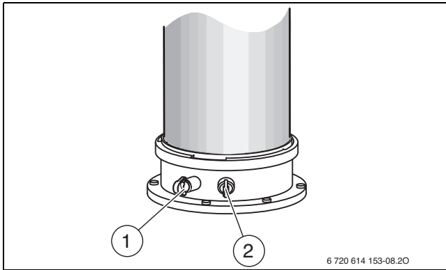
Res. 34 Atık gaz ölçüm ağzı ve yanma havası ölçüm ağzı
