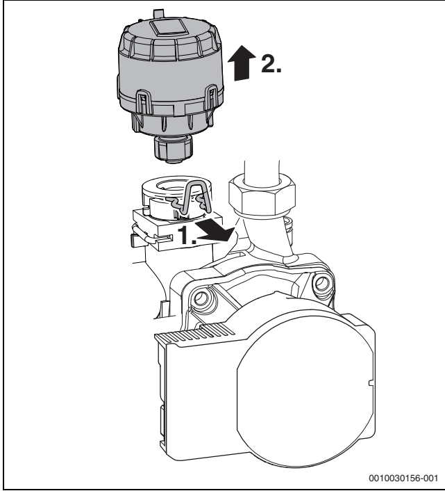
Res. 58 3 yollu vananın motorunun sökülmesi
