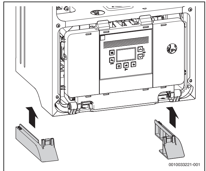
Res. 64 Yan plastik çıtaların takılması
