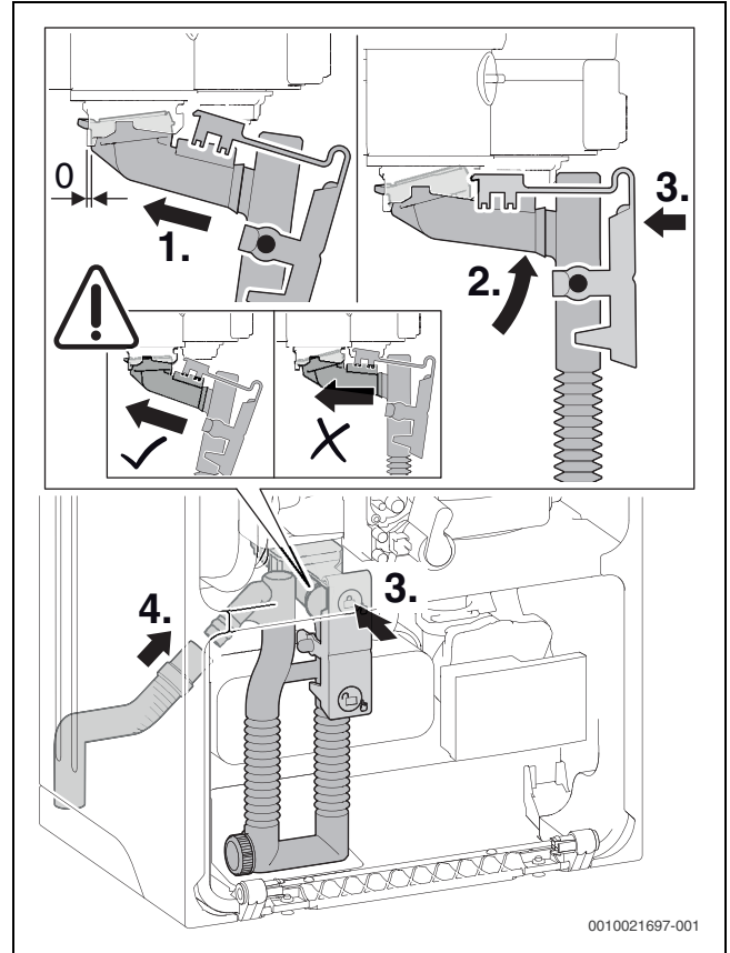
Res. 50 Yoğuşma suyu sifonunun takılması
