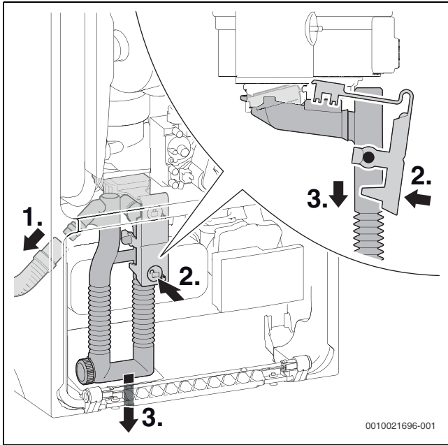
Res. 45 Yoğuşma suyu sifonunun sökülmesi
