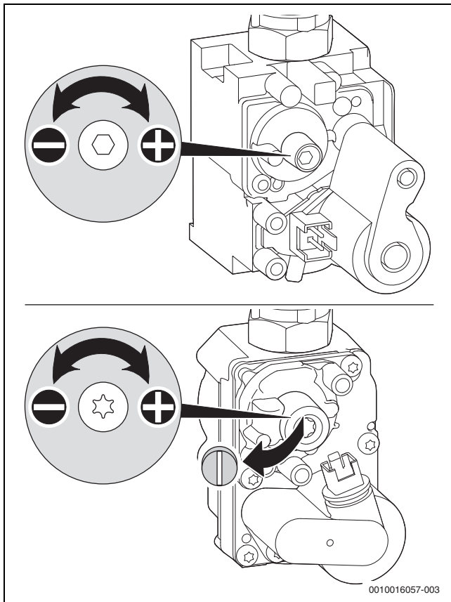
Res. 32 Gaz armatürünün ayar vidasındaki mührün sökülmesi
