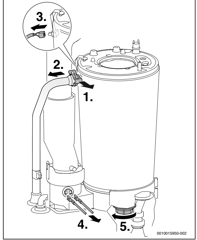
Res. 59 Gidiş suyu borusunu çözün ve kabloyu çekip çıkarın
