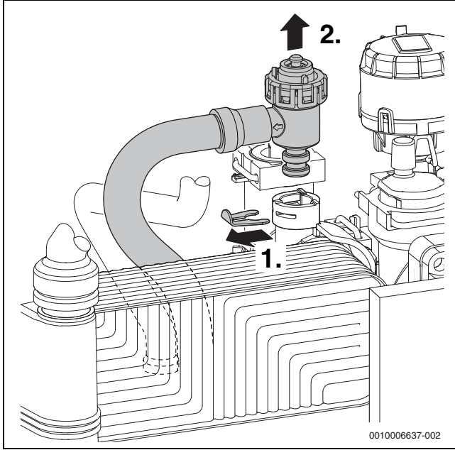
Res. 51 Emniyet ventilinin (ısıtma devresi) çıkarılması
