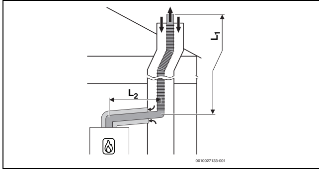
Res. 10 Havalandırma boşluğunda C 93x uyarınca esnek atık gaz tahliyesi ve kurulum yerinde konsantrik hava-atık gaz taşıma sistemi
