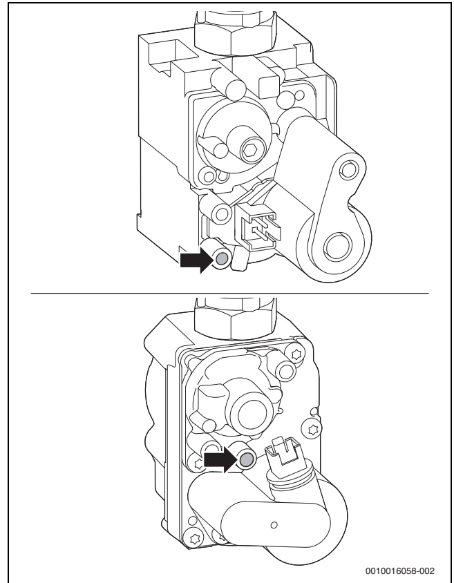
Res. 33 Gaz bağlantı basıncı için ölçüm ağızı
