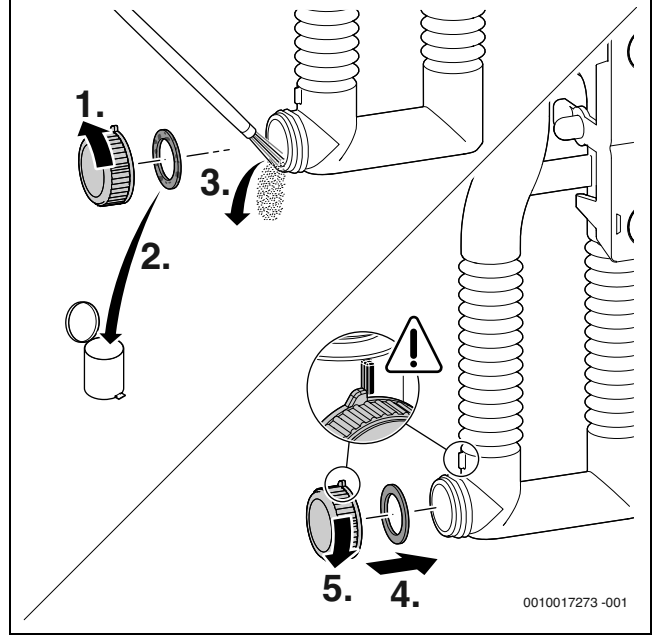
Res. 46 Yoğuşma suyu sifonunun temizlenmesi
