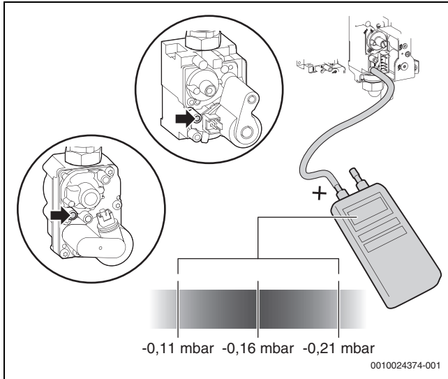
Res. 31 Fark basıncın ölçülmesi
