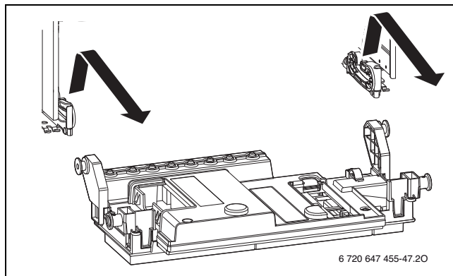
Pav. 81 Valdymo prietaiso išėmimas
