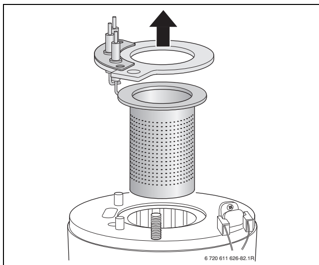
Pav. 61 Degiklio išėmimas
