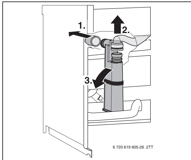
Pav. 67 Kondensato sifono išmontavimas
