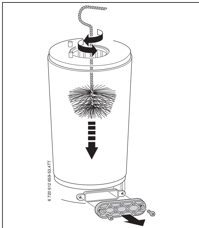
Pav. 64 Šiluminio bloko valymas
