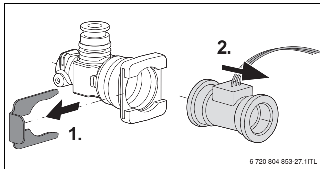
Pav. 71 Turbinos nuėmimas nuo šalto vandens vamzdžio
