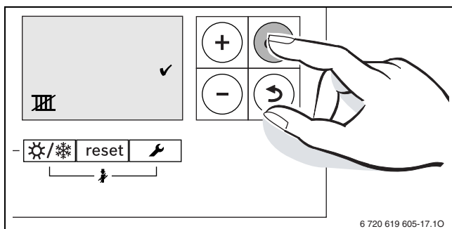
Pav. 47 Rankinio vasaros režimo patvirtinimas
