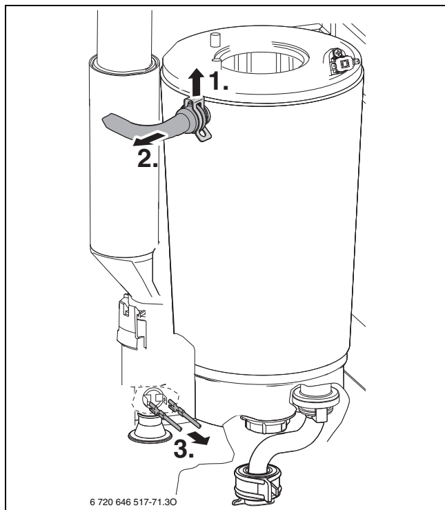
Pav. 82 Tiekiamo srauto vamzdžio ir kabelio atjungimas
