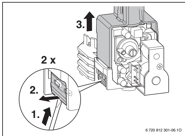
Pav. 77 Dujinės armatūros išmontavimas
