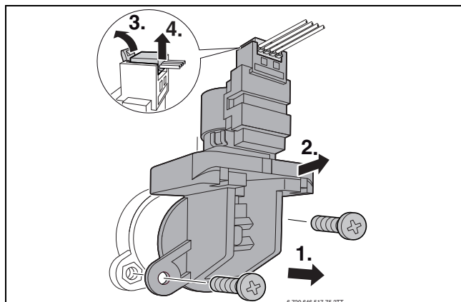
Pav. 74 3-eigio vožtuvo išmontavimas
