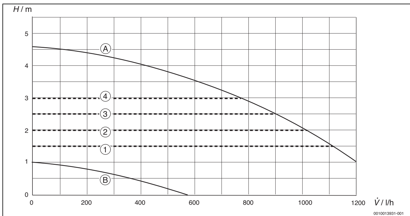
Pav. 89 Siurblio charakteristikos laukai ir charakteristikos
