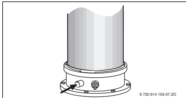
Pav. 52 Išmetamųjų dujų matavimo atvamzdžio
