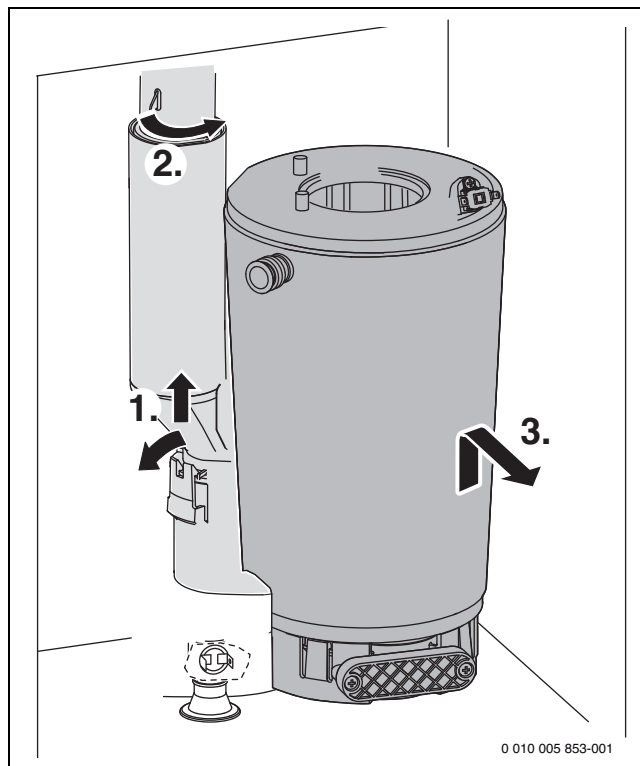
Pav. 84 Šiluminio bloko išmontavimas
