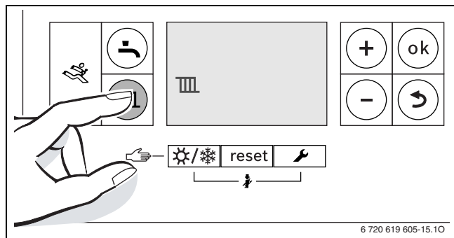
Pav. 38 Šildymo režimo rodmuo
