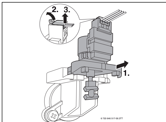
Pav. 73 3-eigio vožtuvo variklio išmontavimas
