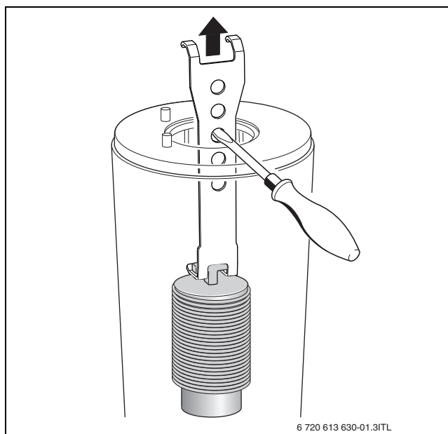
Pav. 63 Apatinio liepsnos kreiptuvo išėmimas
