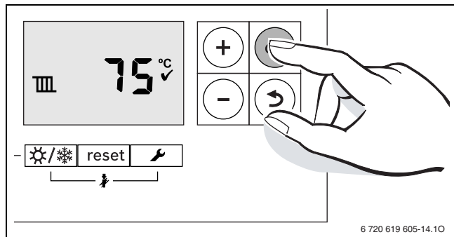
Pav. 39 Šildymo režimo rodmens patvirtinimas
