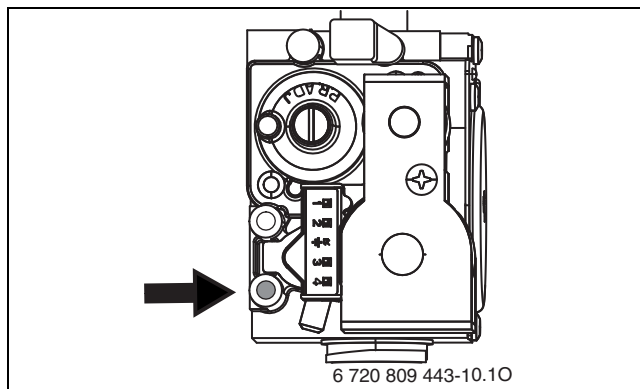
Pav. 55 Dujų slėgio prijungimo taške matavimo atvamzdis
