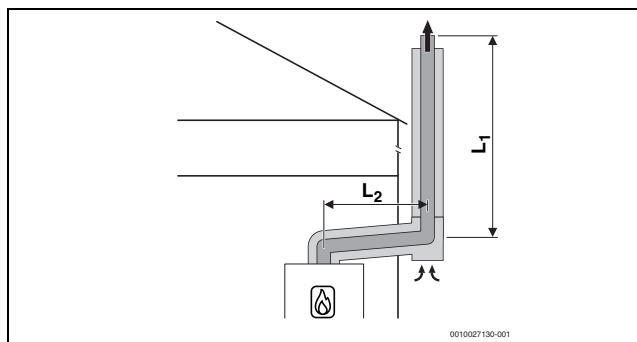
Pav. 13 Koncentrinis oro-išmetamųjų dujų kanalas pagal C 53x ant lauko sienos
