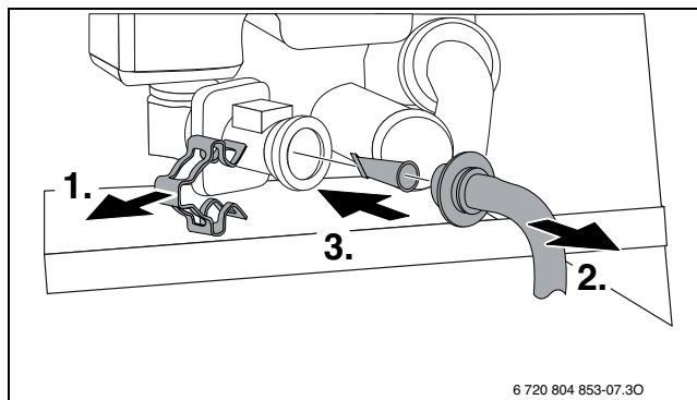
Pav. 70 Filtro išėmimas iš šalto vandens vamzdžio
