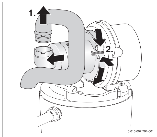
Pav. 59 Įsiurbimo vamzdžio ir maišymo įrenginio išmontavimas
