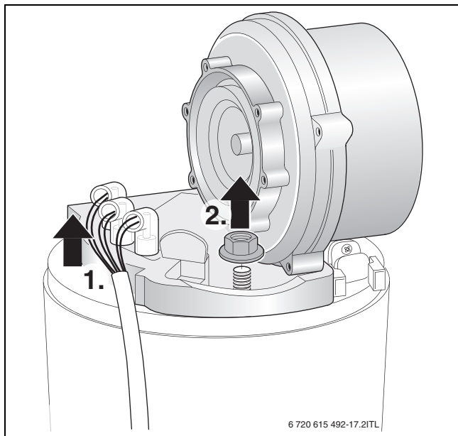
Pav. 60 Ventiliatoriaus išėmimas
