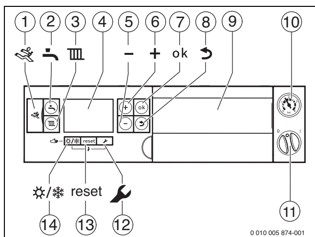
Pav. 36 Valdymo pultas, esant atidarytam valdymo pulto dangteliui
