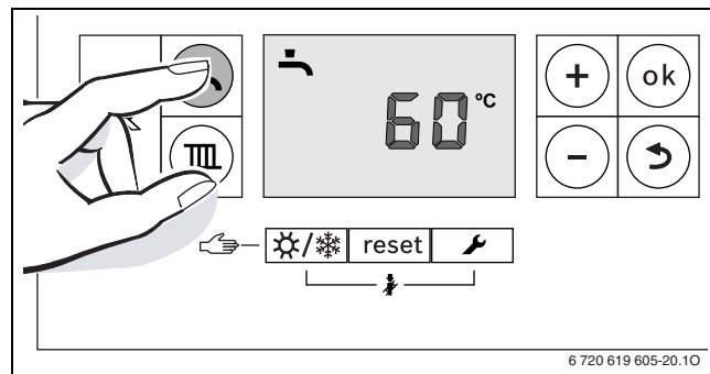
Pav. 44 Karšto vandens temperatūros rodmuo
