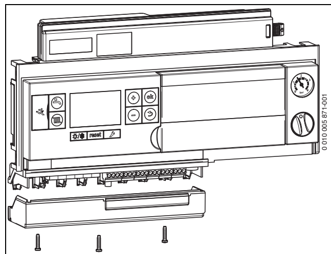
Pav. 34 Dangčio nuėmimas
