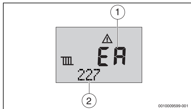
Pav. 86 Pavyzdys: apribojančios trikties rodmuo
