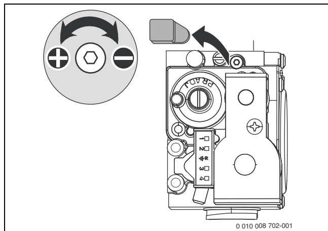
Pav. 53 Plombos nuėmimas
