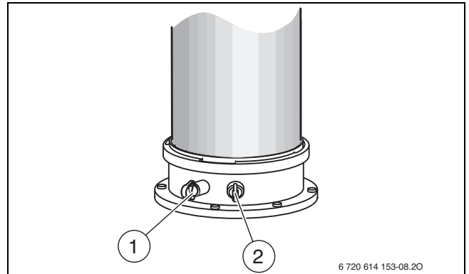
Pav. 57 Išmetamųjų dujų matavimo atvamzdis ir degimui naudojamo oro matavimo atvamzdis
