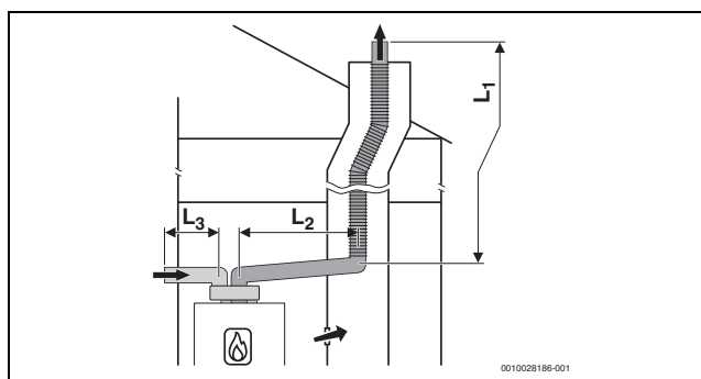
Pav. 12 Lanksti išmetamųjų dujų sistema pagal C 53 šachtoje ir oro-išmetamųjų dujų kanalas su atskirais vamzdžiais oro tiekimui ir išmetamųjų dujų išvedimui pastatymo patalpoje
