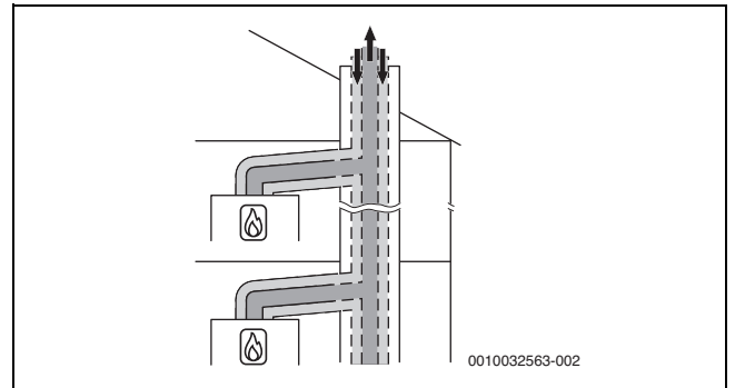
Pav. 20 Būdas, kai prie dūmtraukio jungiami keli įrenginiai pagal C (10)3x su koncentrinio oro-išmetamųjų dujų kanalu pastatymo patalpoje
