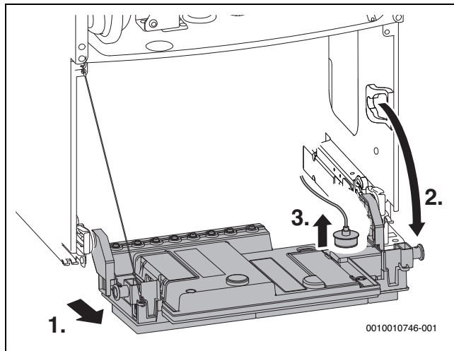
Pav. 79 Valdymo prietaiso nulenkimas žemyn
