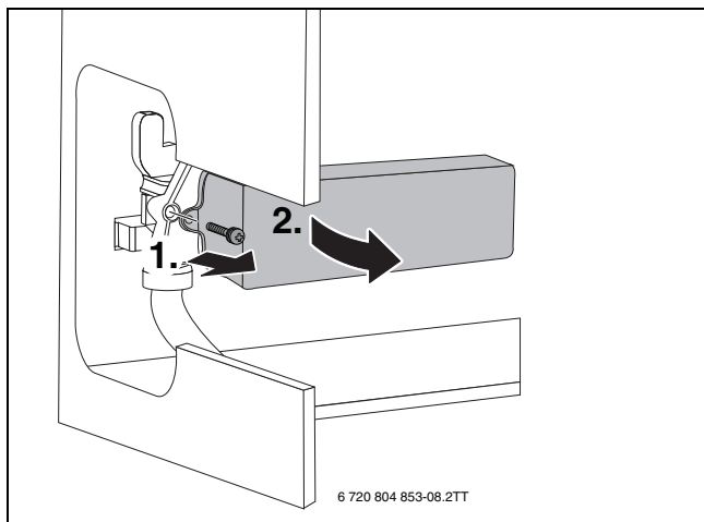
Pav. 69 Plokštelinio šilumokaičio išmontavimas
