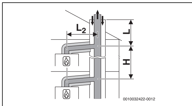
Pav. 22 Būdas, kai prie dūmtraukio jungiami keli įrenginiai pagal C_{(14)3x} su bendra standžia išmetamųjų dujų sistema ir koncentrinio oro-išmetamųjų dujų kanalu pastatymo patalpoje
