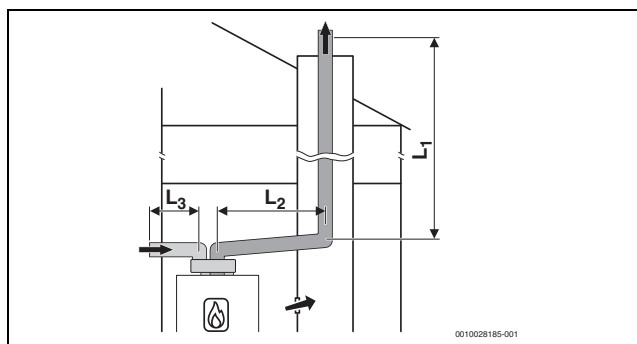
Pav. 11 Standi išmetamųjų dujų sistema pagal C 53 šachtoje ir oro-išmetamųjų dujų kanalas su atskirais vamzdžiais oro tiekimui ir išmetamųjų dujų išvedimui pastatymo patalpoje
