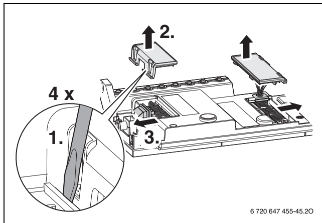
Pav. 80 Dangčio nuėmimas
