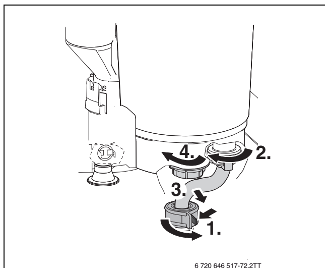
Pav. 83 Veržlių nuėmimas ir grįžtančio srauto vamzdžio atjungimas
