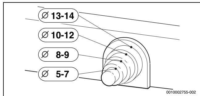
Pav. 35 Apsaugos nuo laidų ištraukimo pritaikymas pagal kabelio skersmenį
