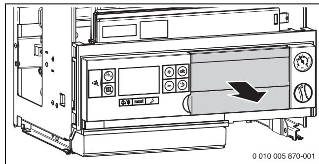
Pav. 33 Dangčio nuėmimas ir valdymo bloko montavimas
