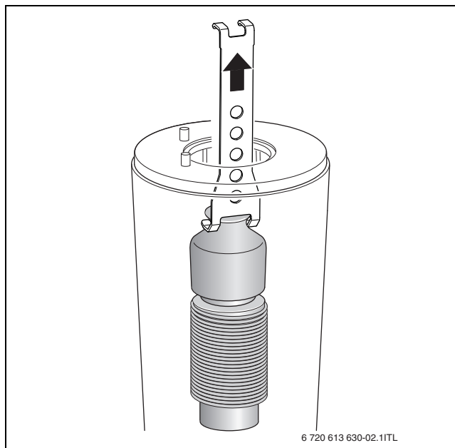
Pav. 62 Viršutinio liepsnos kreiptuvo išėmimas
