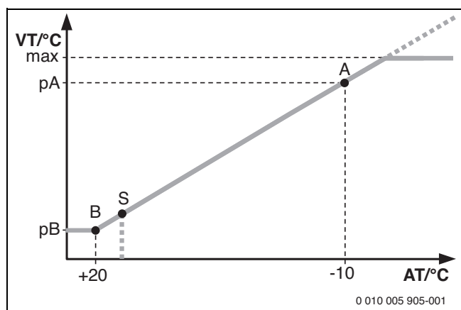
Pav. 88 Šildymo kreivė
