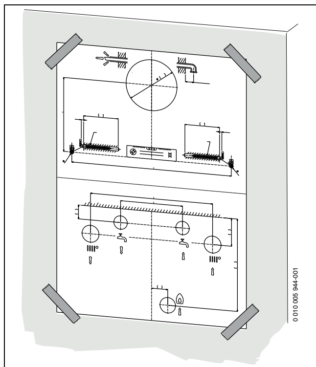
Рис. 14 Монтажный шаблон
