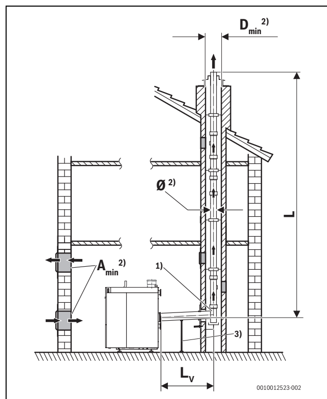
Fig. 18 Condotto combusto intubato in cavedio, variante 1
