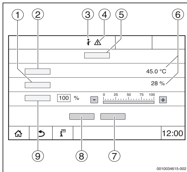
Obr. 14 Zobrazení Test spalín > nastavení kotle
