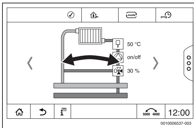
Obr. 10 Přejíždění prstem
