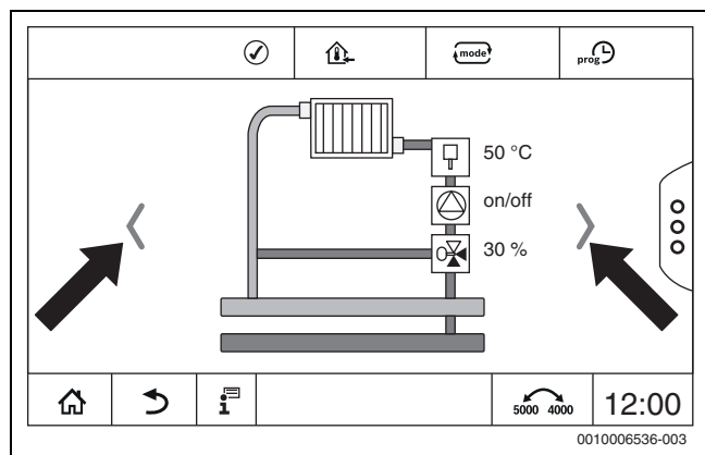
Obr. 9 Listování
