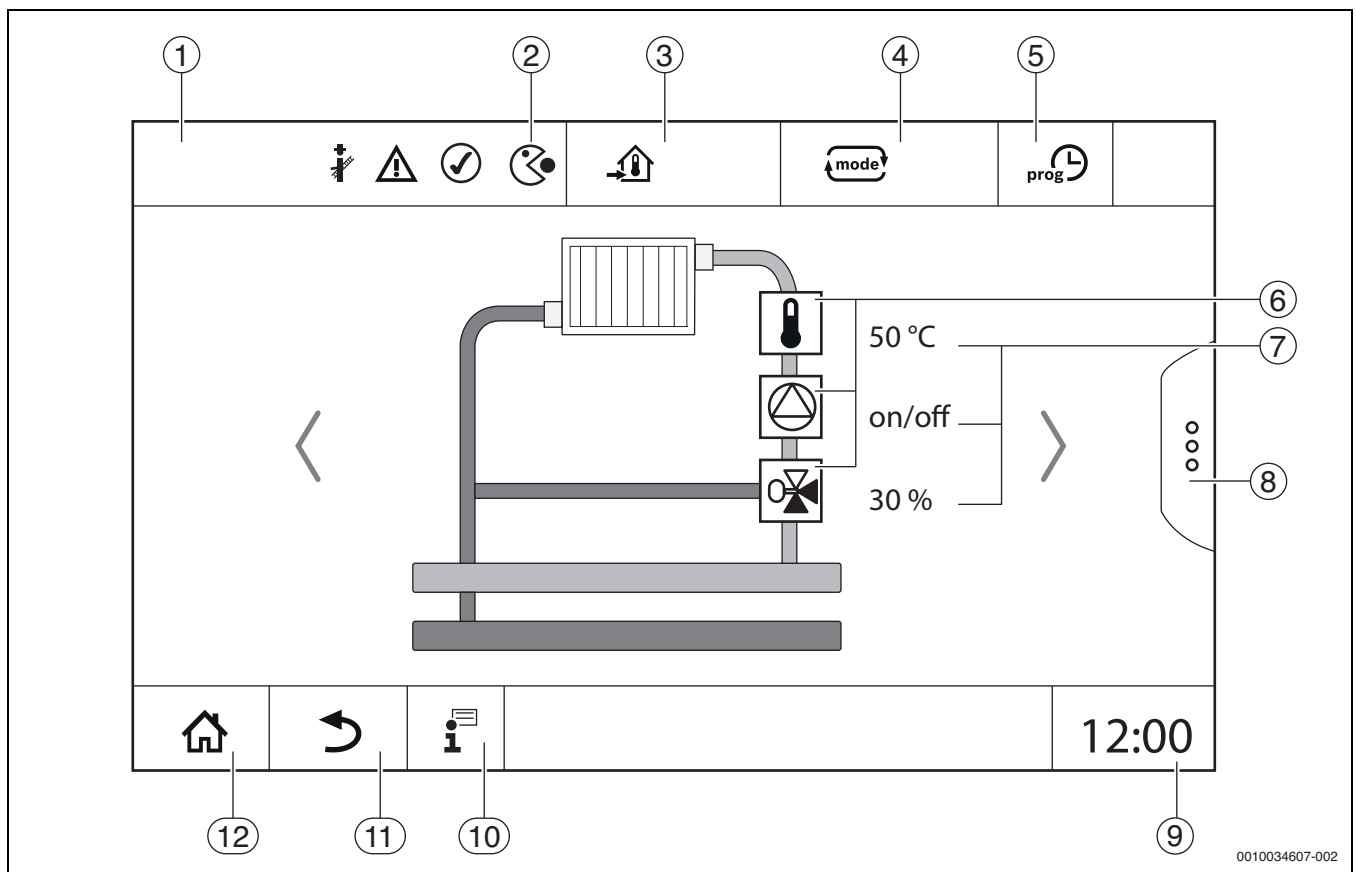
Obr. 6 Ovládací a zobrazovací prvky (příklad)
